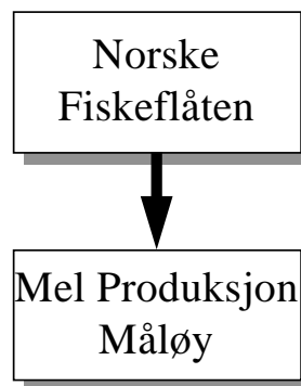
Figur 3.4.1 Produktre for framstilling av fiskemel.
