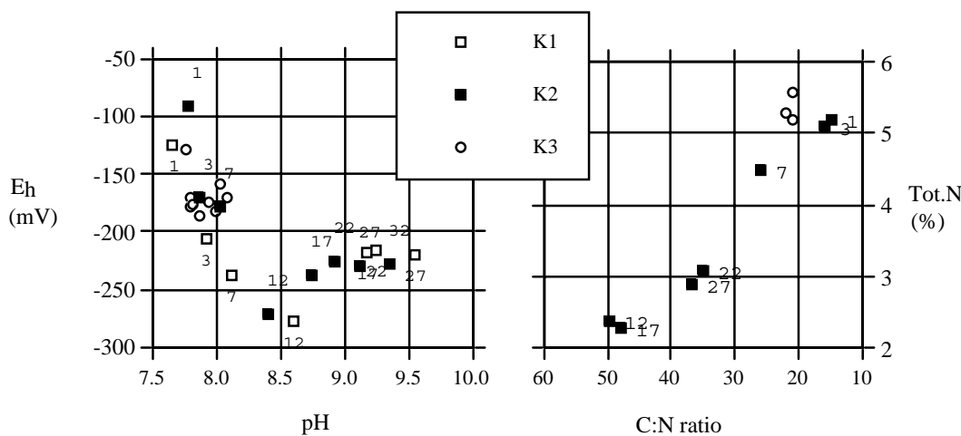
Figur 4. Plot av pH mot E_h og tot.N mot C:N forholdet i alle prøver analysert i K1, K2 og K3. Tallene angir respektive sedimentdyb på K1 og K2.
