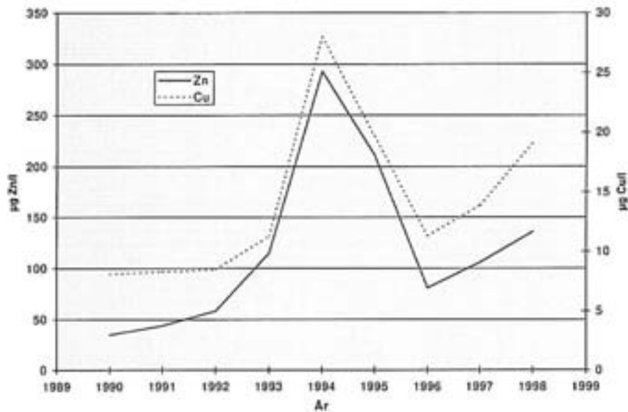
Figur 6. Årlige middelverdier for kobber og sink ved st. 6B.
