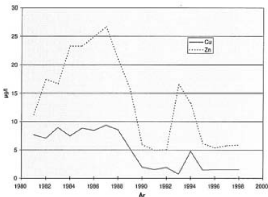
Figur 11. Middelverdier for kobber og sink 1981-98. St. 11 Utløp Vektarbotn.
