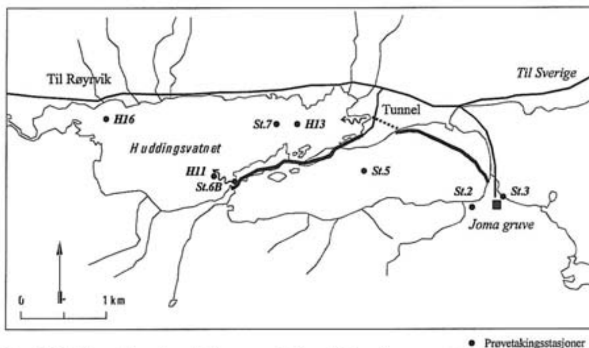
Figur 3. Huddingsvatn med markering av prøvetakingsstasjoner for vann- og sedimentprøver.
