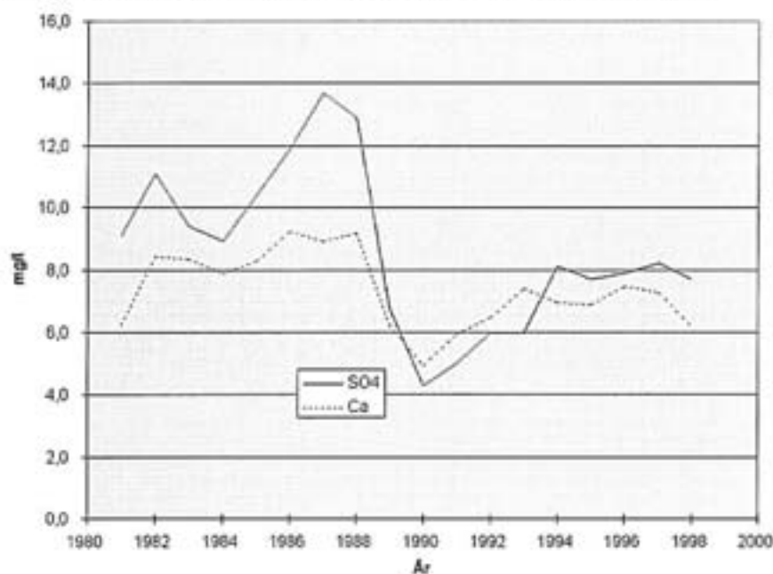
Figur 10. Middelverdier for sulfat og kalsium 1981-98. St. 11 Utløp Vektarbotn.
