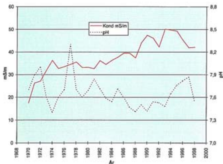
Figur 4. Utviklingen i middelverdier for pH og konduktivitet i gruvevannet fra Joma
