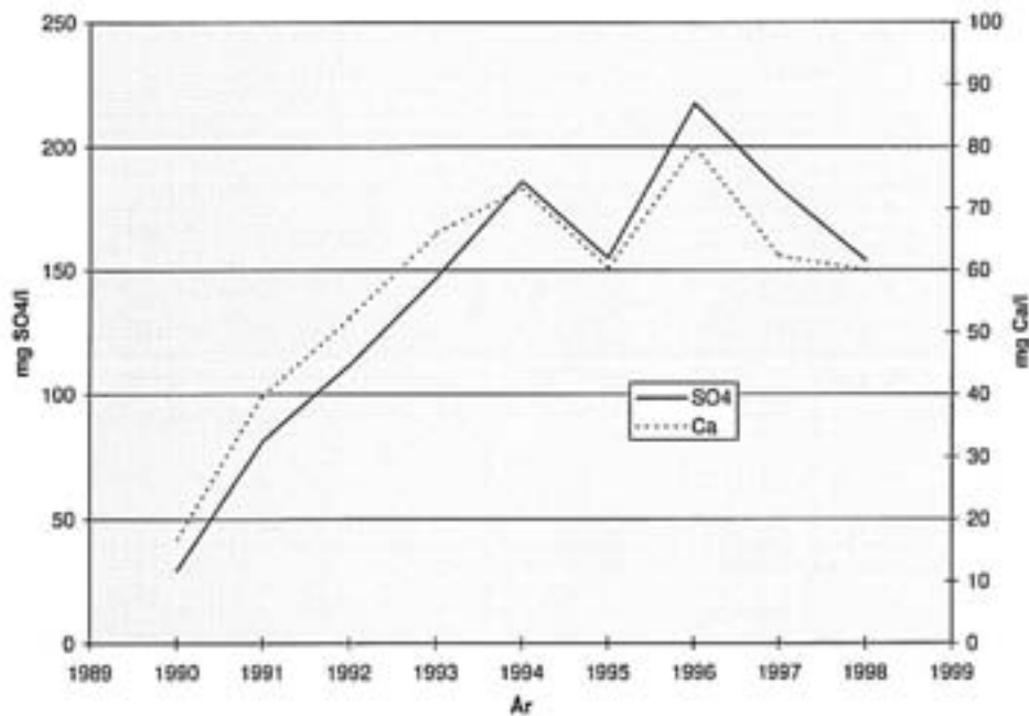
Figur 7. Årlige middelverdier for sulfat og kalsium ved st. 6B.
