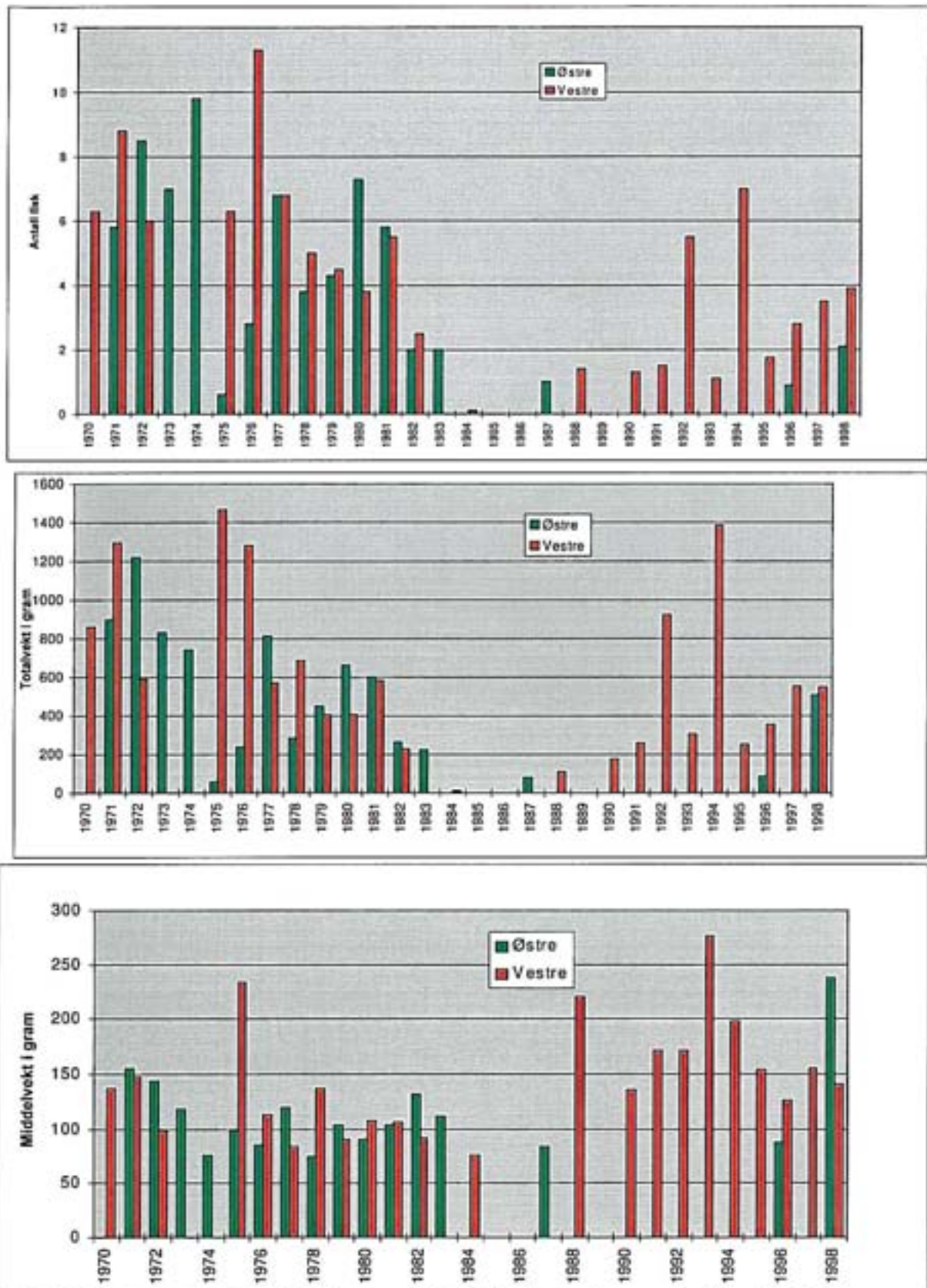
Figur 13. Fangst pr. garnnett i Huddingsvatn i 1970-98. Fire utvalgte maskevidder: 21, 26, 35 og 40 mm. Gruvestart 1972- og -tiltak 1989.
