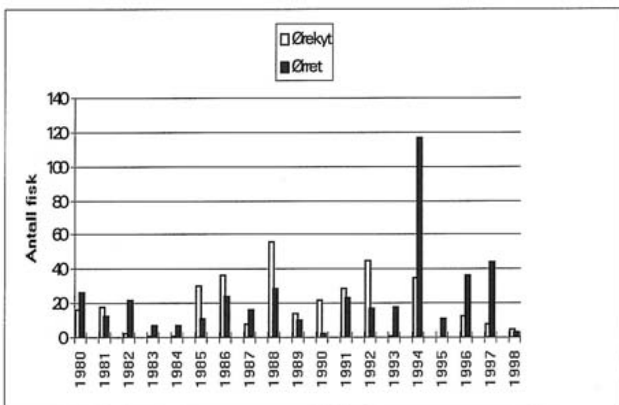
Figur 17. Elektrofiske i Huddingselva (st. 8) 1980-1998. Antall fisk pr. 30 minutter.
