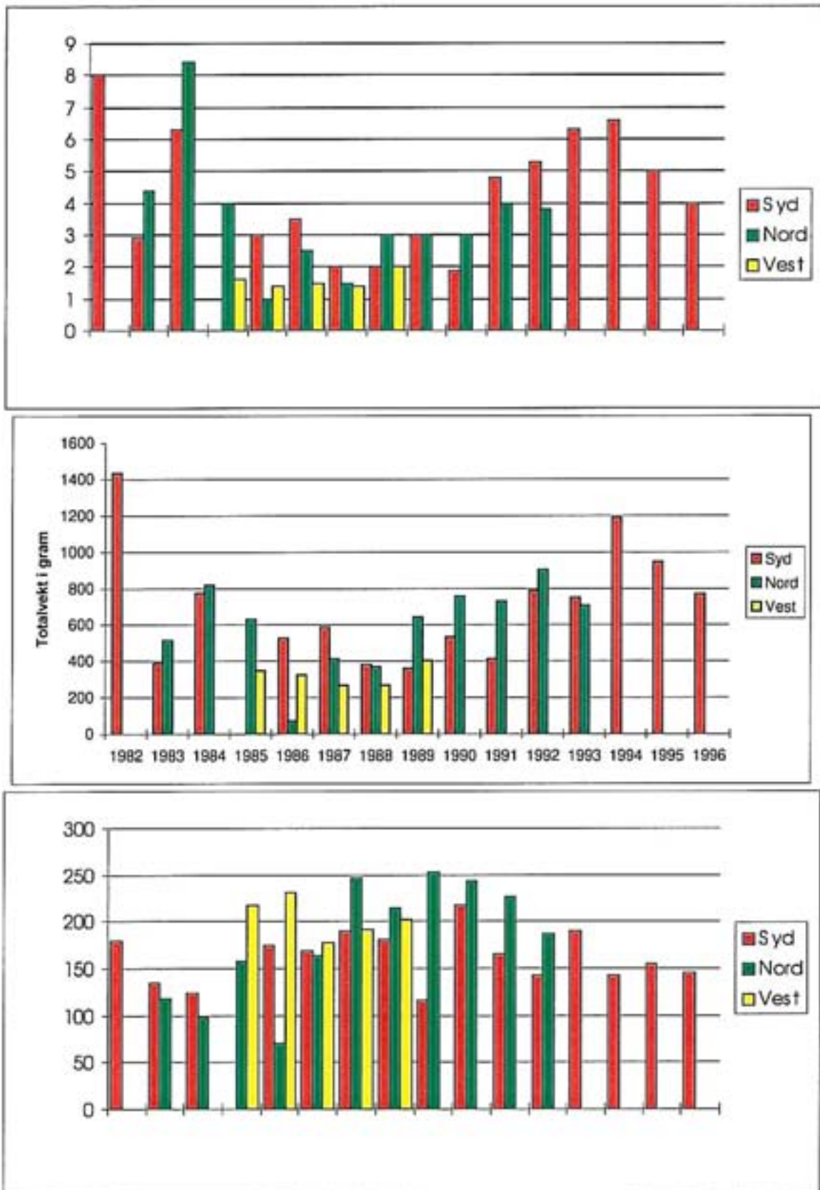
Figur 14. Fangst pr. garnnett i Vektarbotn 1982-1997. "Jensen"-serie.
