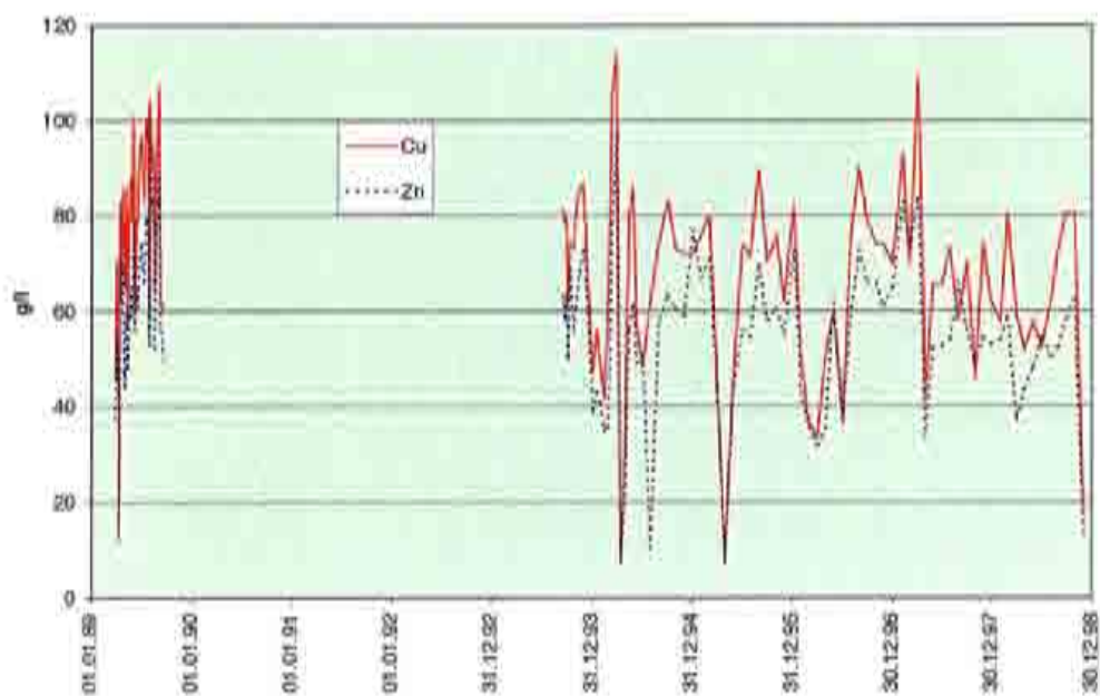
Figur 19. Kobber- og sinkkonsentrasjoner ved st.2 (slamdamm)1989-1998.
