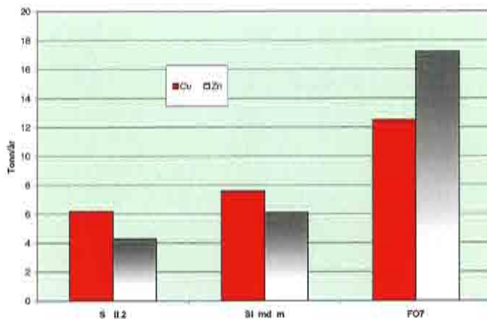
Figur 29. Årstransport av kobber og sink for stasjonene ved Follidal sentrum i 1998.
