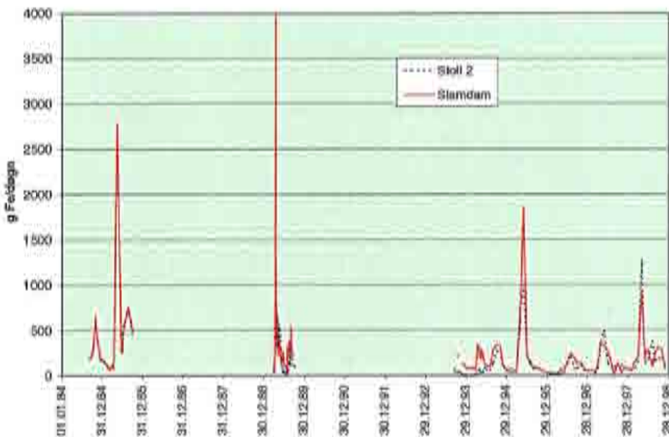
Figur 25. Transport av jern fra gruveområdet i Folldal sentrum ved Stasjon 1-stoll 2 og Stasjon 2-samlet avløp på drenering nedenfor gamle slamdam.
