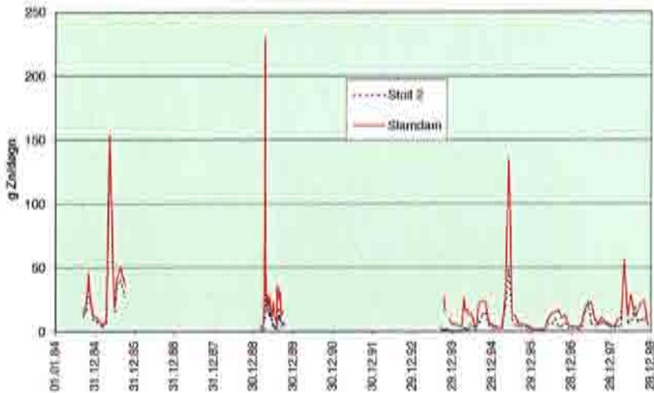
Figur 24. Transport av sink fra gruveområdet i Folldal sentrum ved Stasjon 1-stoll 2 og Stasjon 2-samlet avløp på drenering nedenfor gamle slamdam.
