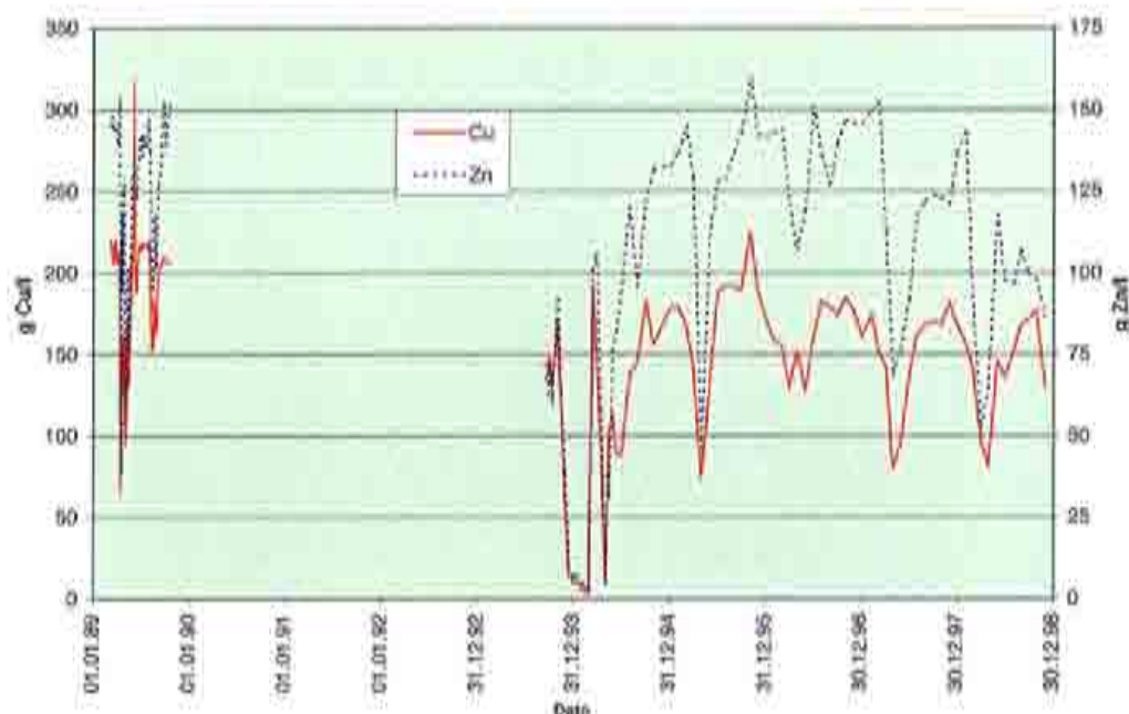
Figur 17. Kobber- og sinkkonsentrasjoner ved st.1 (stoll 2) 1989-1998.
