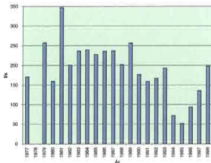
Figur 3. Tidsveiede årsmiddelvannføringer ved overløpet av slamdamm Hjerkin
