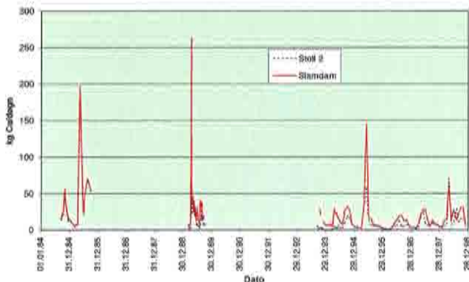
Figur 23. Transport av kobber fra gruveområdet i Follidal sentrum ved Stasjon 1-stoll2 og Stasjon 2-samlet avløp på drenerledning nedenfor gamle slamdam.
