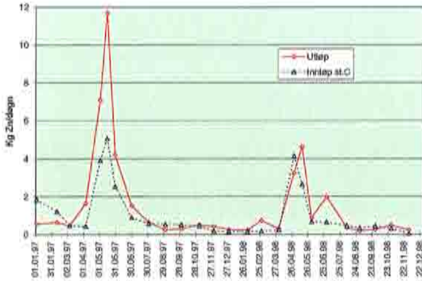
Figur 21. Sinktransport i innløpsbekk (st.C) og ved overløp av slamdam, Hjerking 1998.
