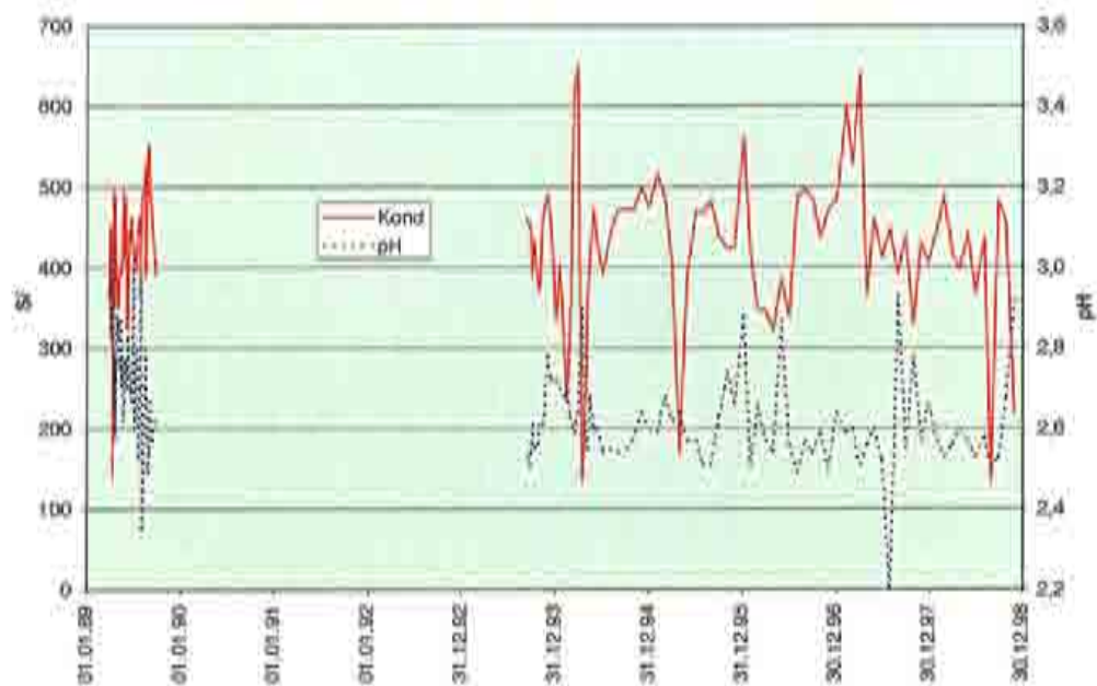
Figur 18. pH- og konduktivetsobservasjoner ved st.2 (slamdamm)1989-1998.
