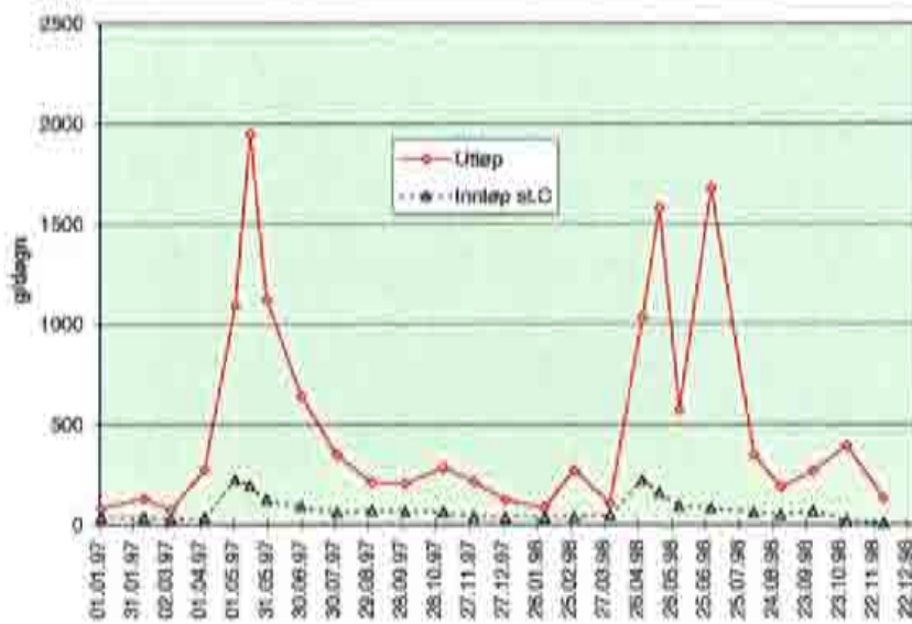
Figur 22. Sulfattransport i innløpsbekk (st.C) og ved overløp av slamdam, Hjerking 1998.
