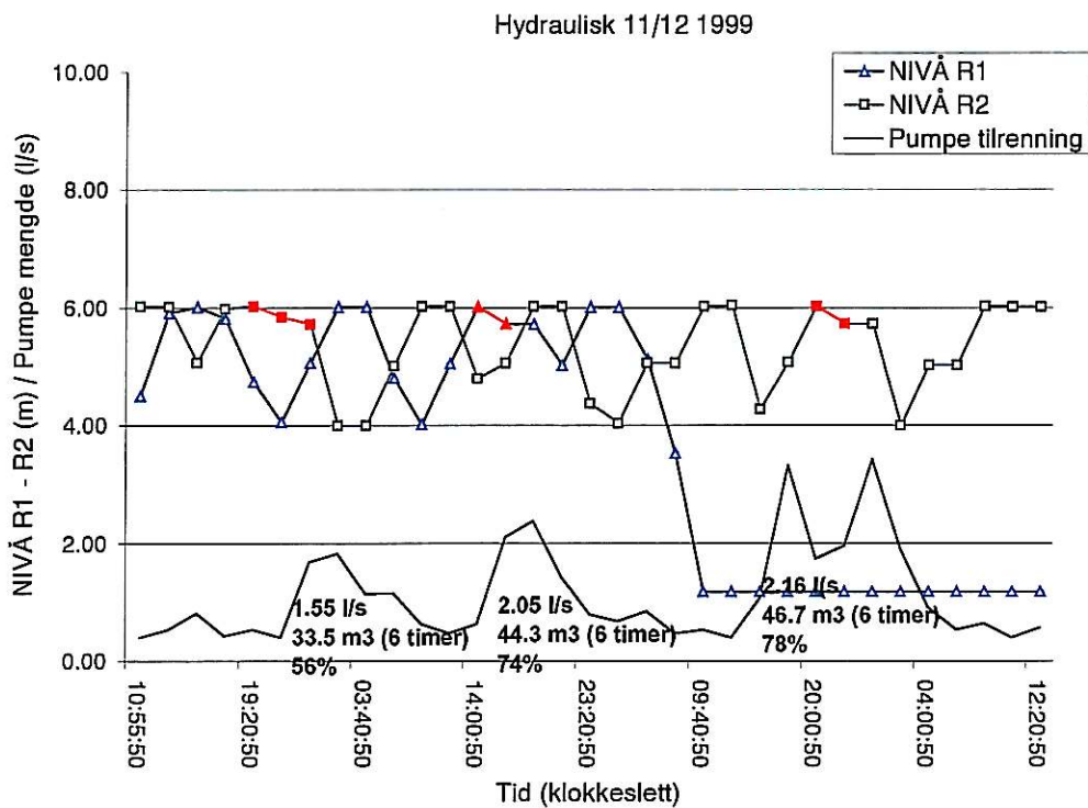
Figur 16. Figuren viser drenering av vann gjennom basseng 1 den 27/10 1998 (nedbørsrikt døgn) og den 9 - 11/12 1999 (nedbørsfattig periode). Slamtildeling er merket med rødt. Gjennomstrømming av dreneringsvann fremgår av sort heltrukken linje.
