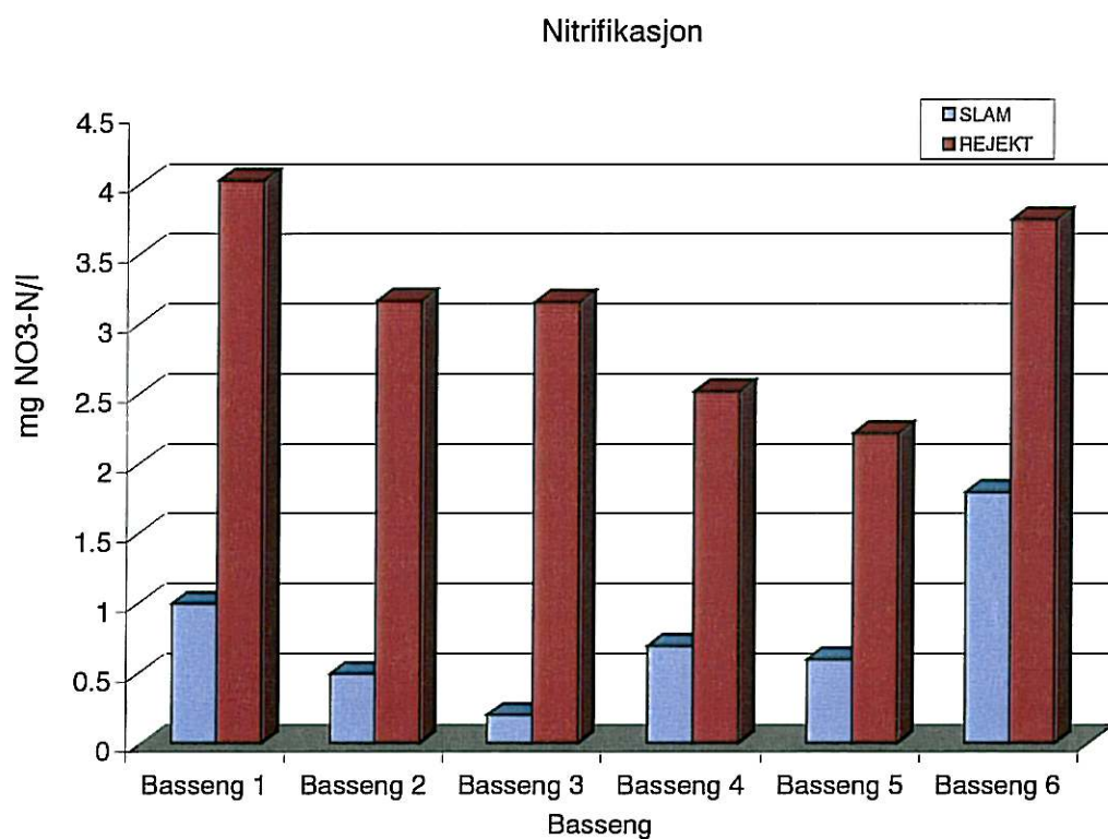
Figur 27. Konsentrasjonen av NO 3 -N i slammet fra rensanlegget og i rejektivannet fra de ulike bassengene.
