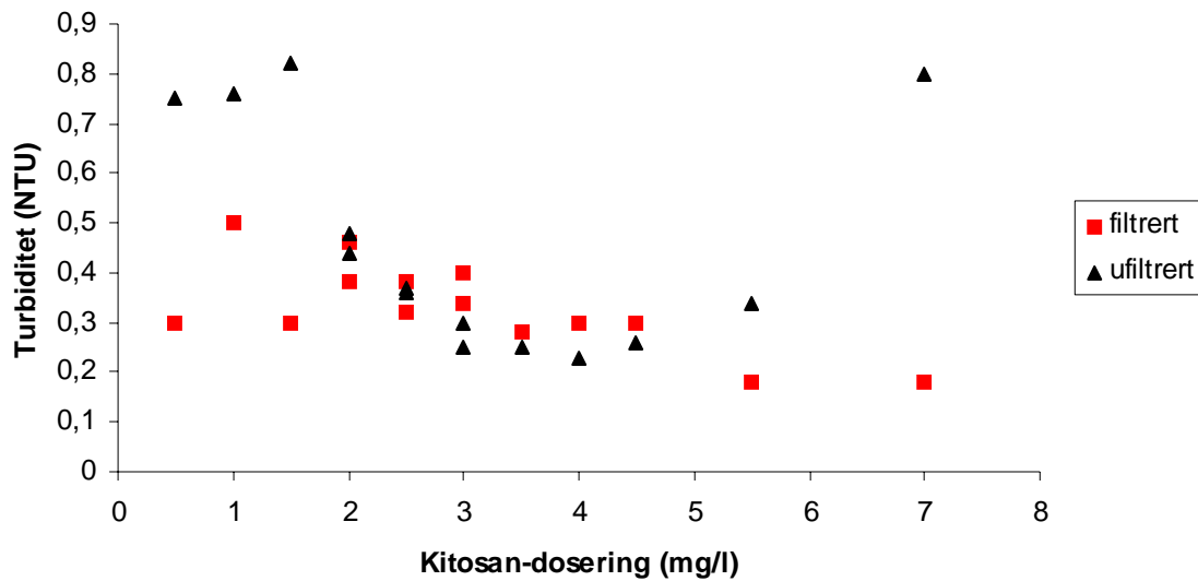
Figur 3. Turbiditet (filtrert og ufiltrert) ved økende kitosan-doseringer i jar-tester hvor pH ble justert til 6. Råvannets turbiditet i filtrert og ufiltrert prøve var henholdsvis 0,28 og 0,72 NTU.
