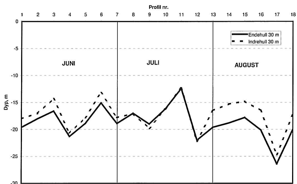
Figur 5. AB-side og CD-side. Beregning av innlagringsdyp for utslipp av avløpsvann i juni-august gjennom utløpsledning til 30 m dyp og diffusorens innerste hull og endehull. Den øvre horisontale akse viser profilnr.
