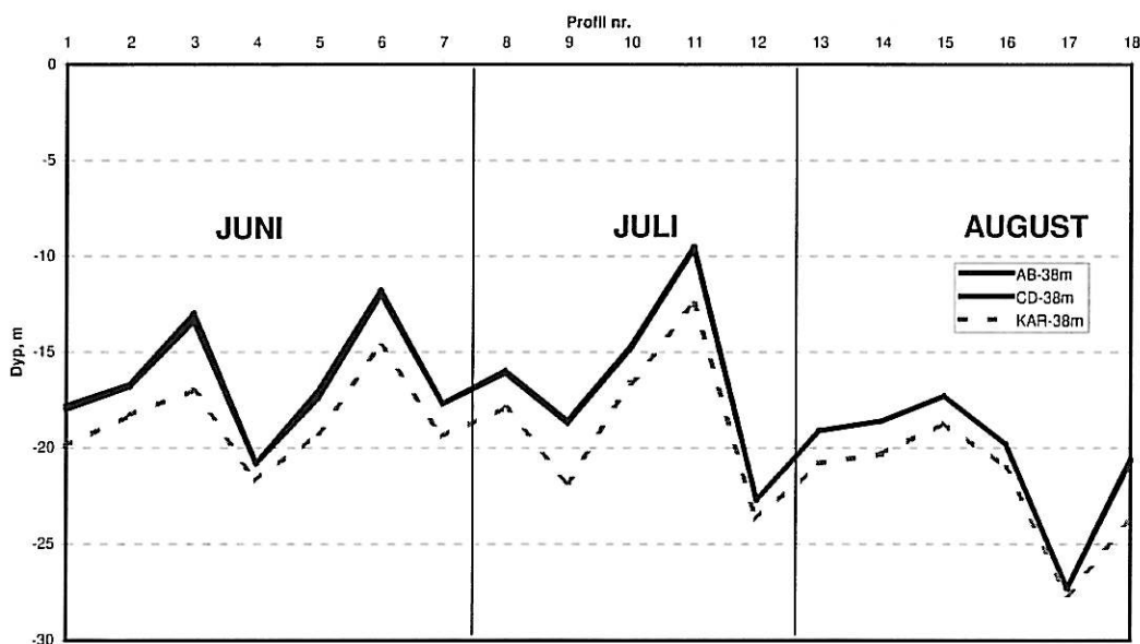
Figur 4. Innlagringsdyp for utslipp fra AB-side, CD-side og KAR-side i 38 m dyp uten diffusor i juni, juli og august. AB-side og CD-side har i alt vesentlig samme innlagringsdyp. For datoer som profilene representerer, se Vedlegg A.
