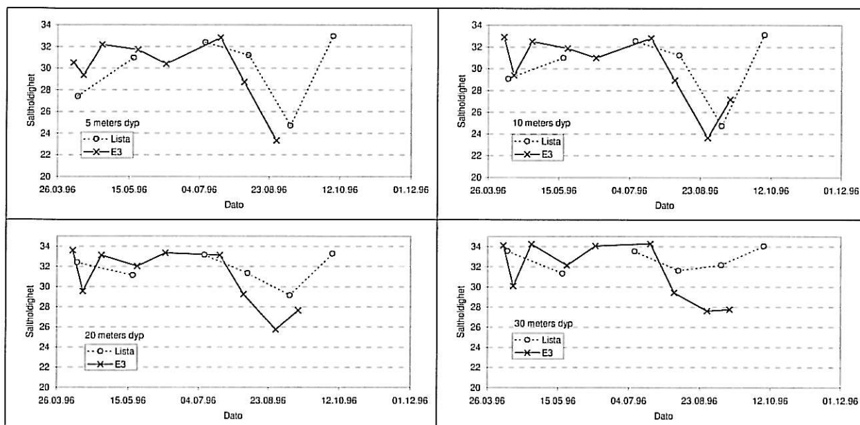
Figur 4. Saltholdighet på 5, 10, 20 og 30 meters dyp ved Sørågapet (E3) og Lista.
