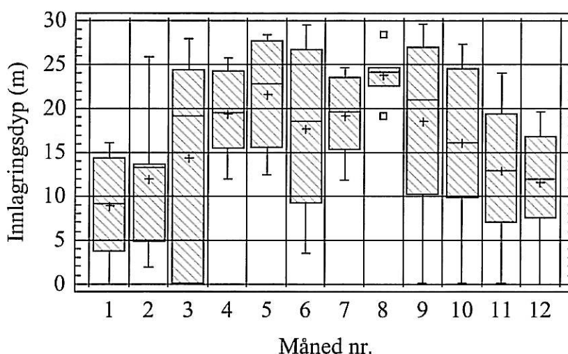
Figur 8. Beregnet innlagingsdyp ut fra sjiktningen ved Lista (80 observasjoner fordelt på ulike måneder fra tidsrommet 1990-96). Utslippsdyp 40 m. (Merk vertikal akse: største dyp øverst.)
