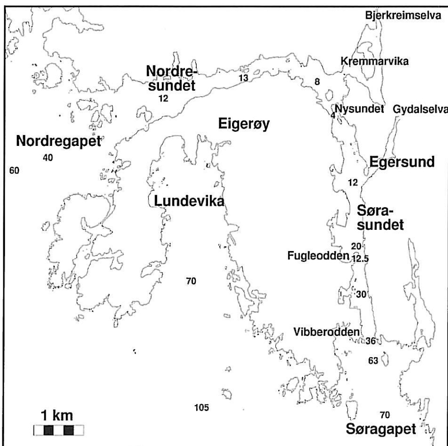
Figur 1. Kart over Eigersund havn, Eigerøy og nærliggende område. Tallene viser bunndyp i meter.
