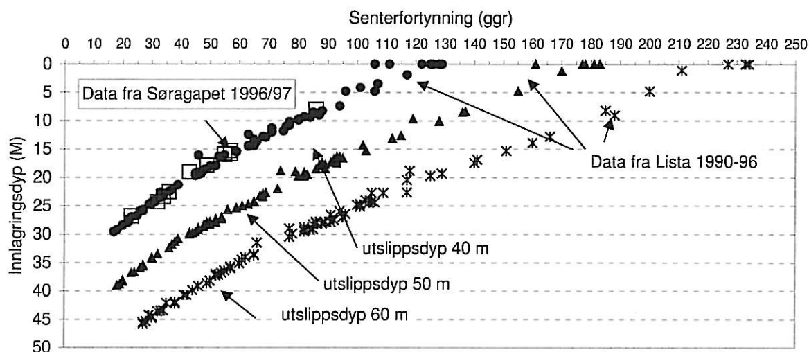
Figur 7. Innlagring og senterfortynning for det planlagte utslippet til Sørøragapet beregnet på observasjoner fra Lista 1990-96. Utslippsdyp 40, 50 og 60 m.
