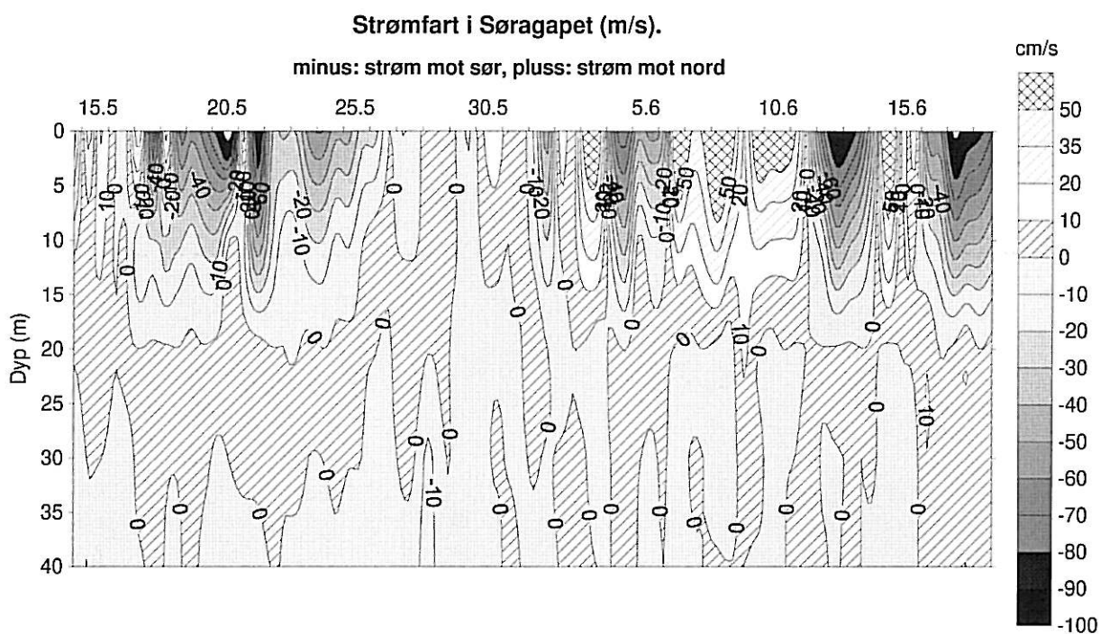
Figur 18. Midlere nord/syd strømmer i Søragapet (DCM 12). Hastigheten er målt over 16 meters intervaller. Dato på horisontal akse.
