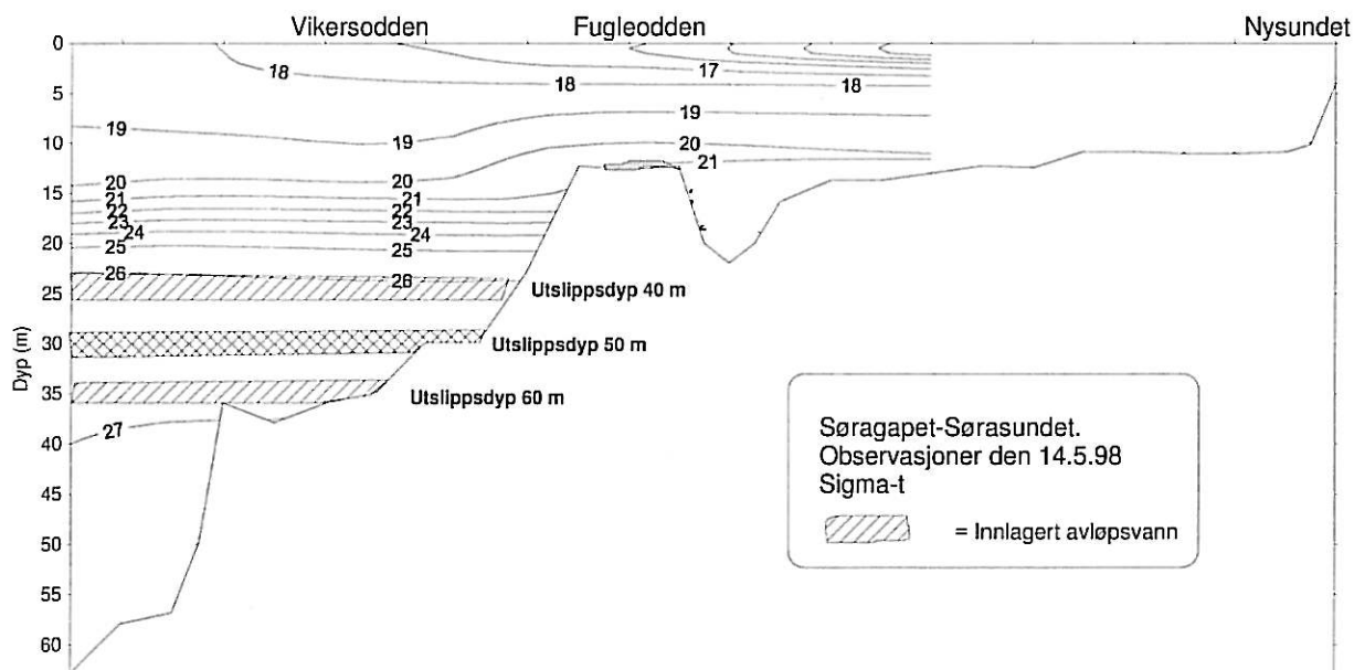
Figur 17. Vannets egenvekt (sigma-t) i Søragapet og innover i Sørasedet den 14/5-1998 og spredningen av innlagret avløpsvann ved utslipp på 40, 50 og 60 meters dyp i Søragapet.
