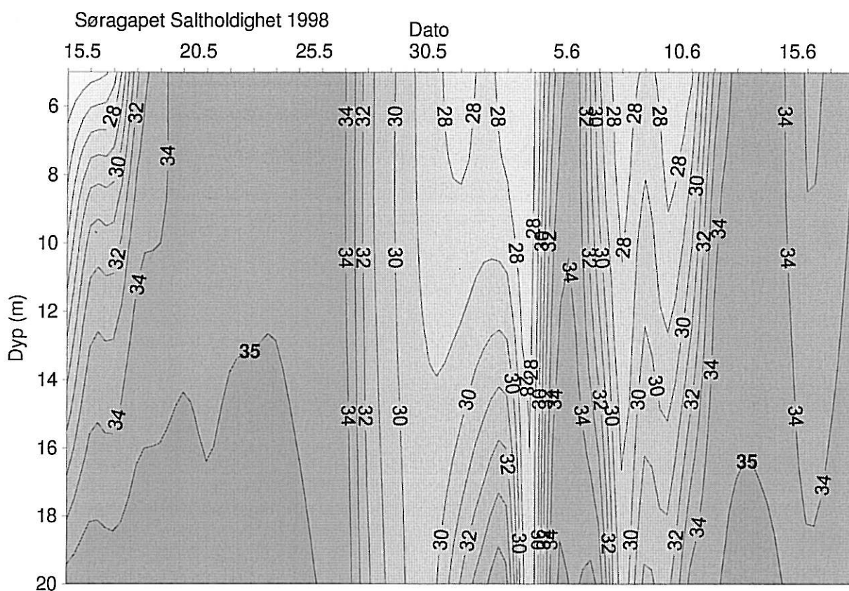
Figur 20. Saltholdighetsvariasjonen i Sørágapet. Døgnmiddel av 10 minutters observasjoner.
