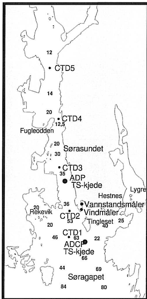
Figur 3. Kart over Egersund havn, Sørgapet og Sørasundet. Målestasjonene er merket. Tallene viser dyp i meter.
