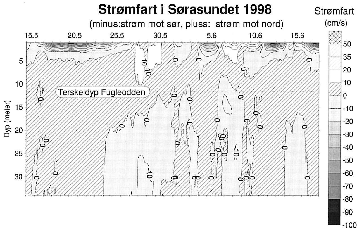
Figur 19. Midlere nord/syd strømmer i Sørasundet (ADP). Hastigheten er målt over 1 meters intervaller. Dato på horisontal akse.
