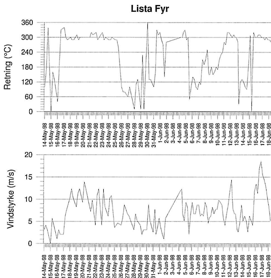
Figur 22. Vindmålinger ved Lista Fyr. Data fra Meteorologisk institutt.
