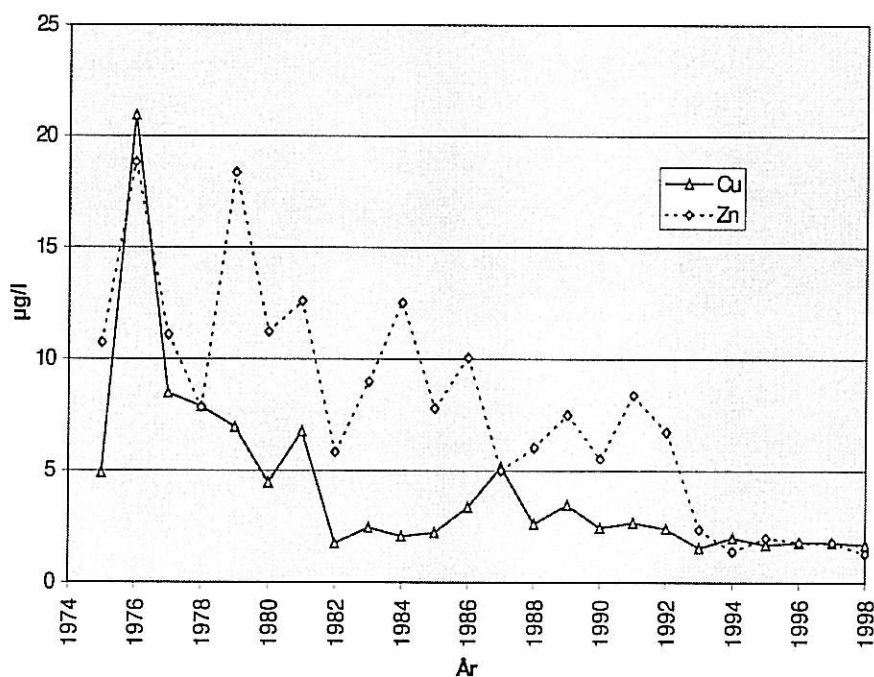
Figur 7 Kobber- og sinkkonsentrasjoner presentert som tidsveide middelverdier (µg/l). Stasjon : Rønningen for perioden 1975 - 1993 og for Bjørset fra 1994 - 1998.
