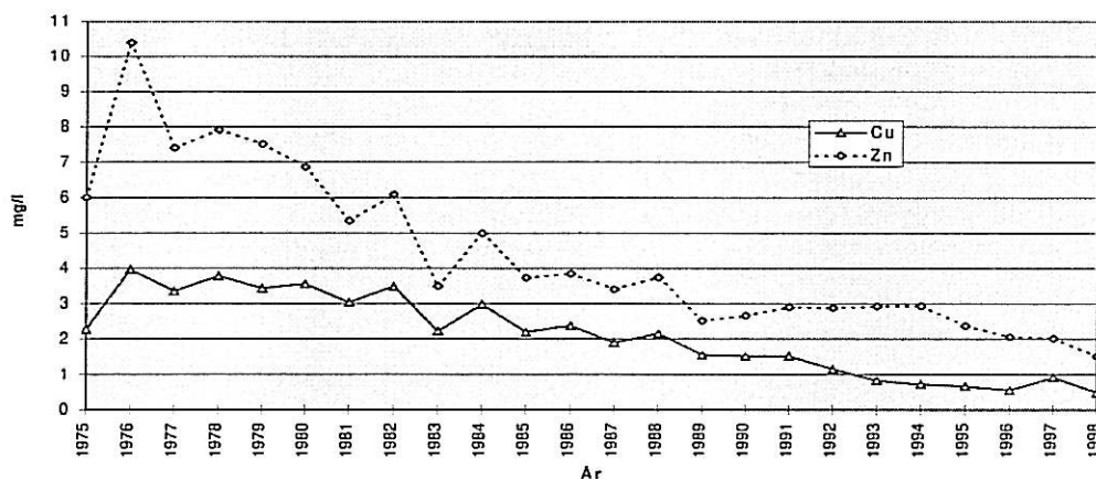
Figur 6. Kobber- og sinkkonsentrasjoner presentert som tidsveide middelerverdier for stasjonen i Raubekken ved Salberg for perioden 1975-1998. ( mg / l ).
