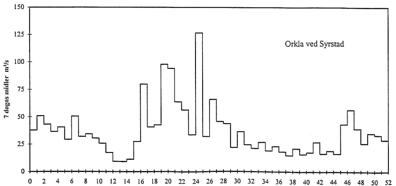
Figur 4. B : Karakteristiske 7-døgns midler for vannføringen i Orkla ved Syrstad i 1996.
