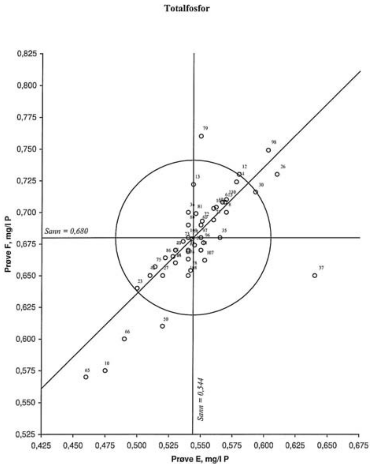
Figur 11. Youdendiagram for totalfosfor, prøvepar EF Akseptansegrensen, angitt med en sirkel, er 10 %
