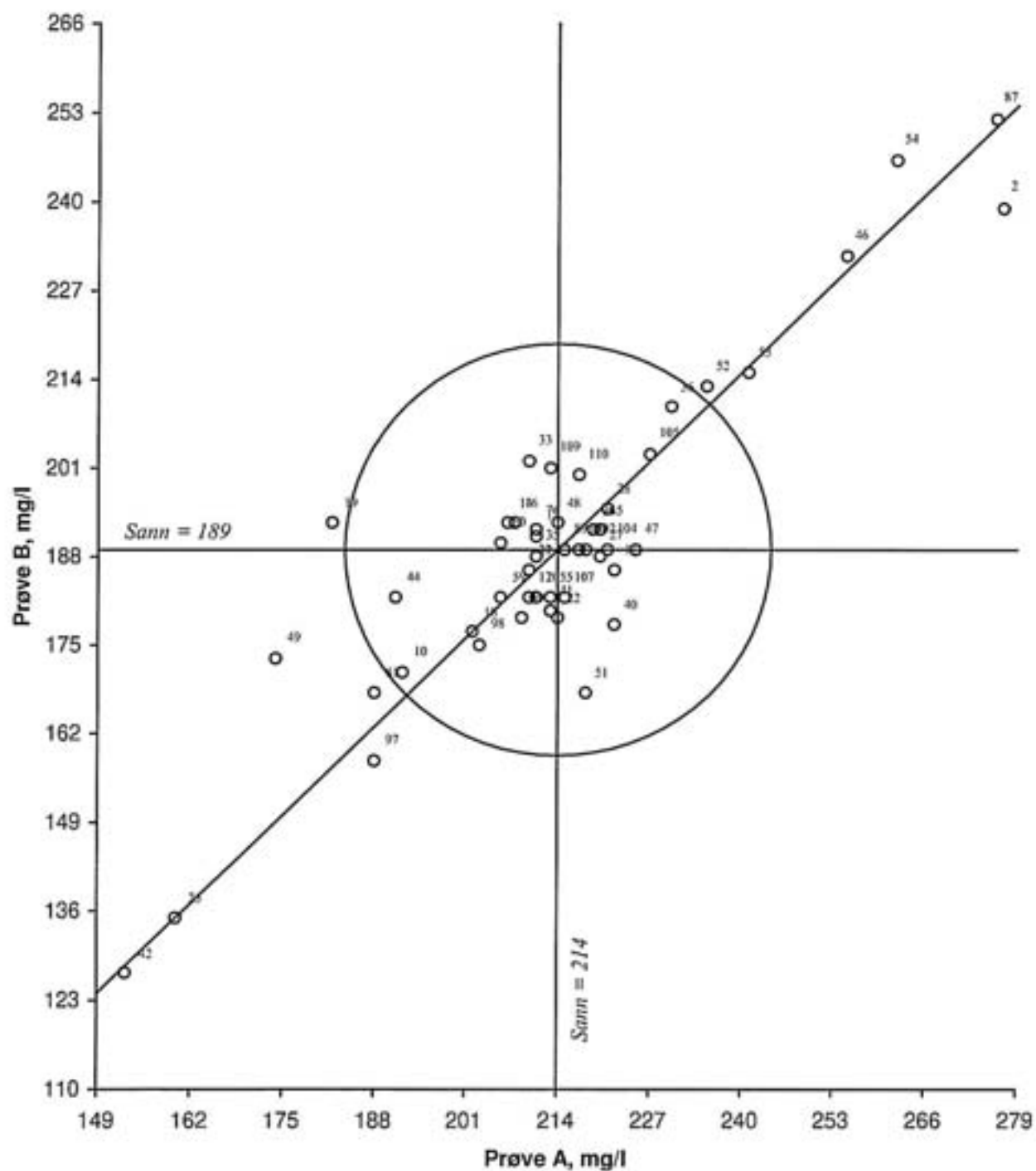
Figur 5. Youdendiagram for suspendert stoff, gløderest, prøvepar AB Akseptansgrensen, angitt med en sirkel, er 15 %
