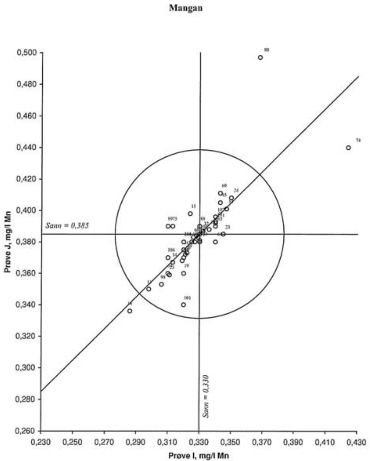
Figur 27. Youdendiagram for mangan, prøvepar IJ Akseptansegrensen, angitt med en sirkel, er 15 %
