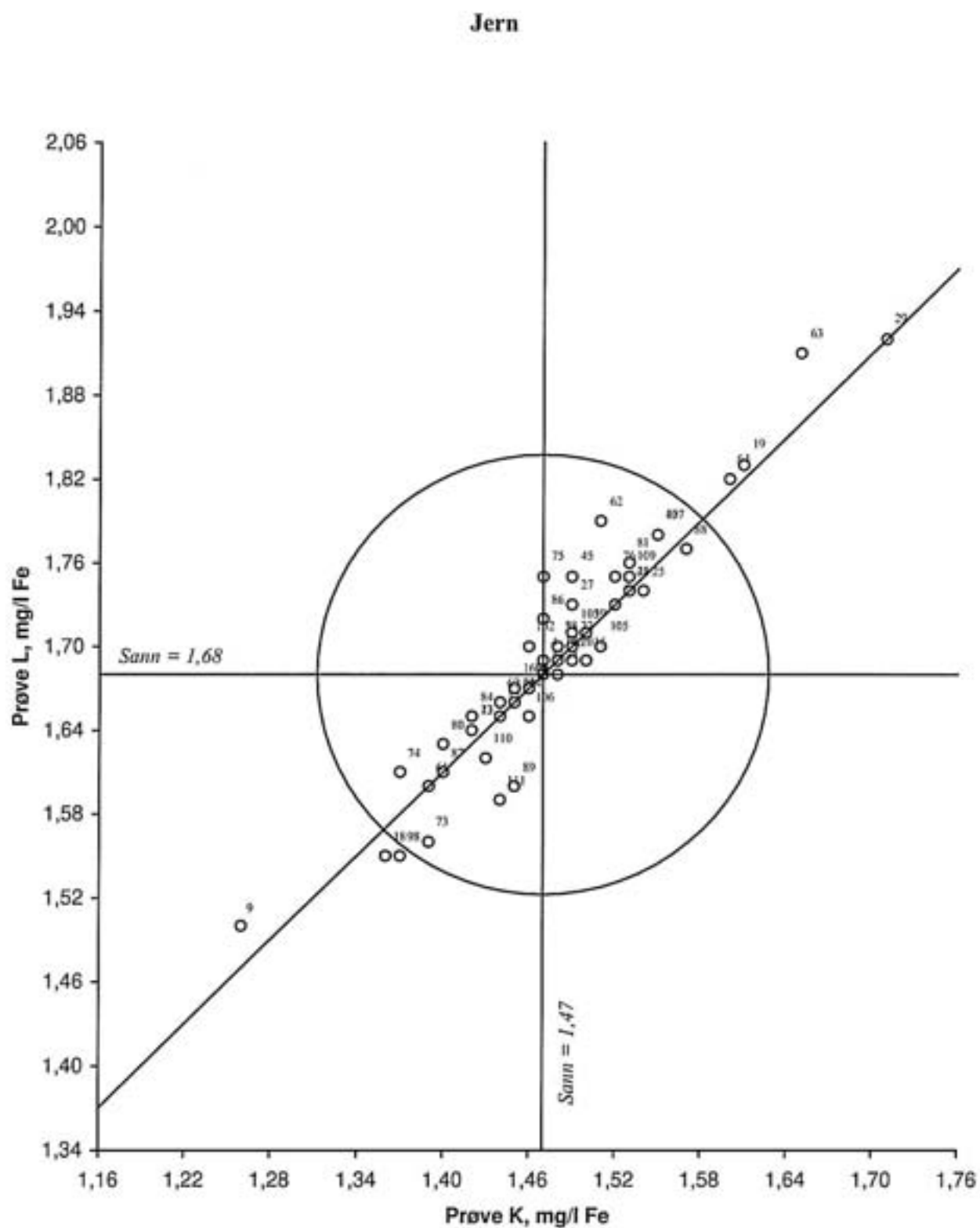
Figur 20. Youdendiagram for jern, prøvepar KL Akseptansgrensen, angitt med en sirkel, er 10 %
