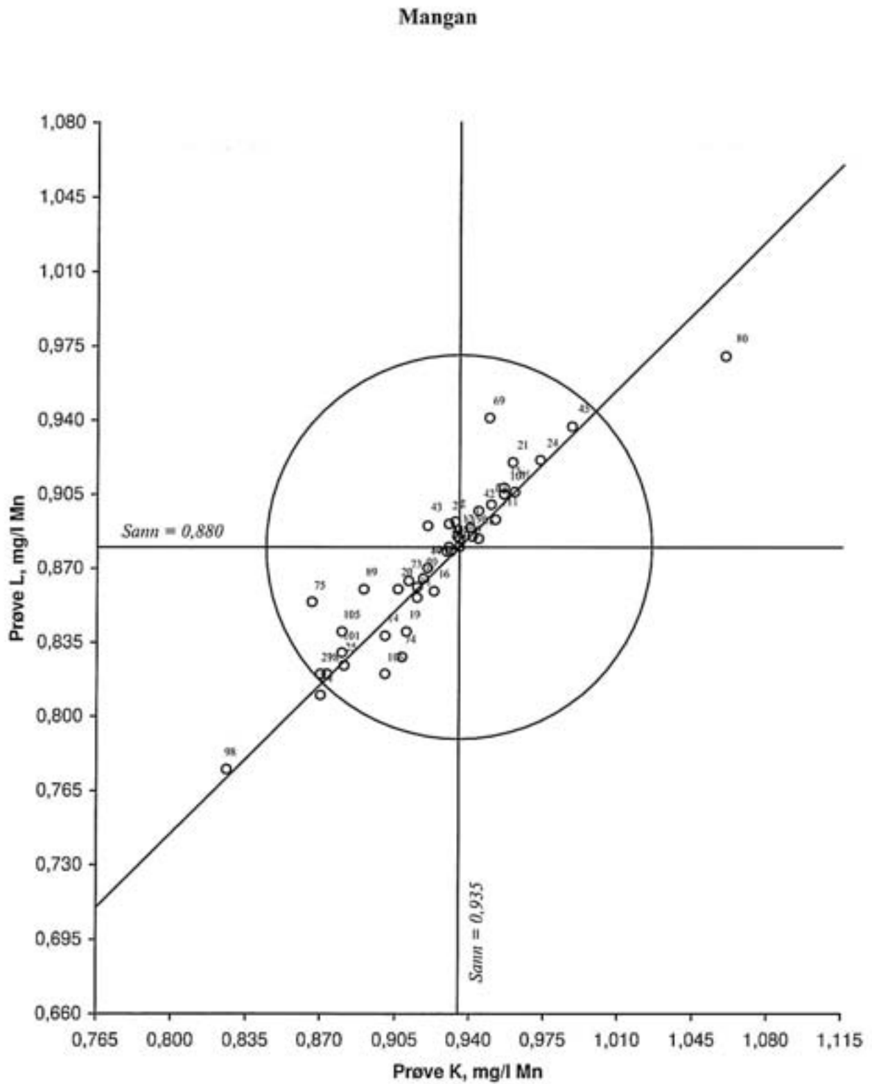
Figur 28. Youdendiagram for mangan, prøvepar KL Akseptansgrensen, angitt med en sirkel, er 10 %
