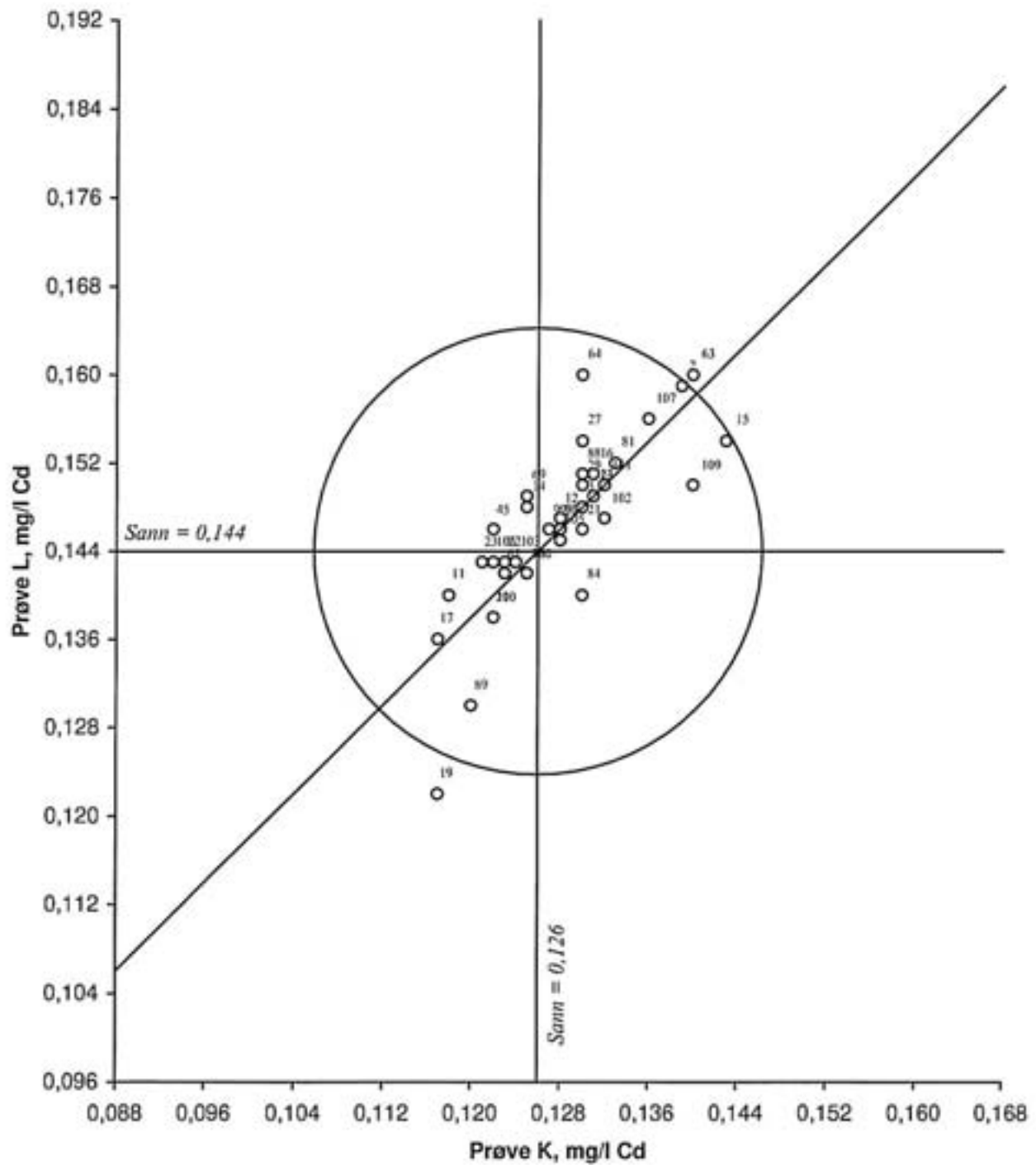
Figur 22. Youdendiagram for kadmium, prøvepar KL Akseptansgrensen, angitt med en sirkel, er 15 %
