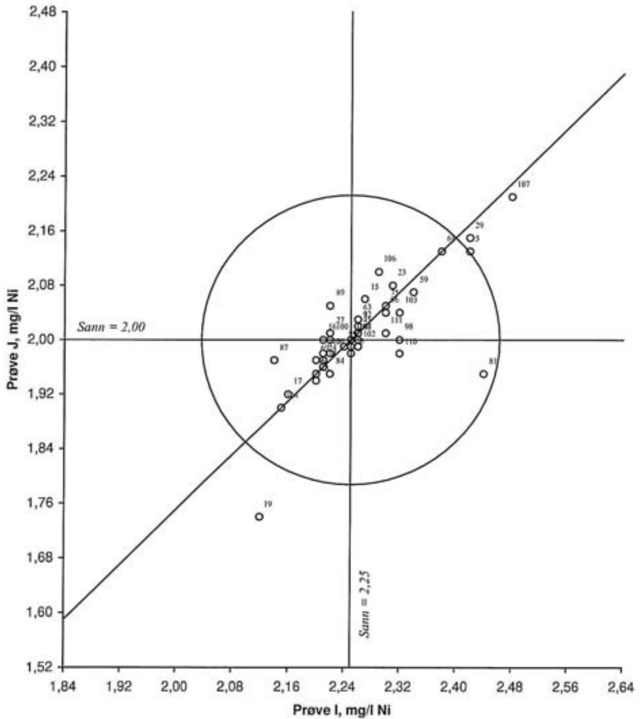
Figur 29. Youdendiagram for nikkell, prøvepar IJ Akseptansegrensen, angitt med en sirkel, er 10 %
