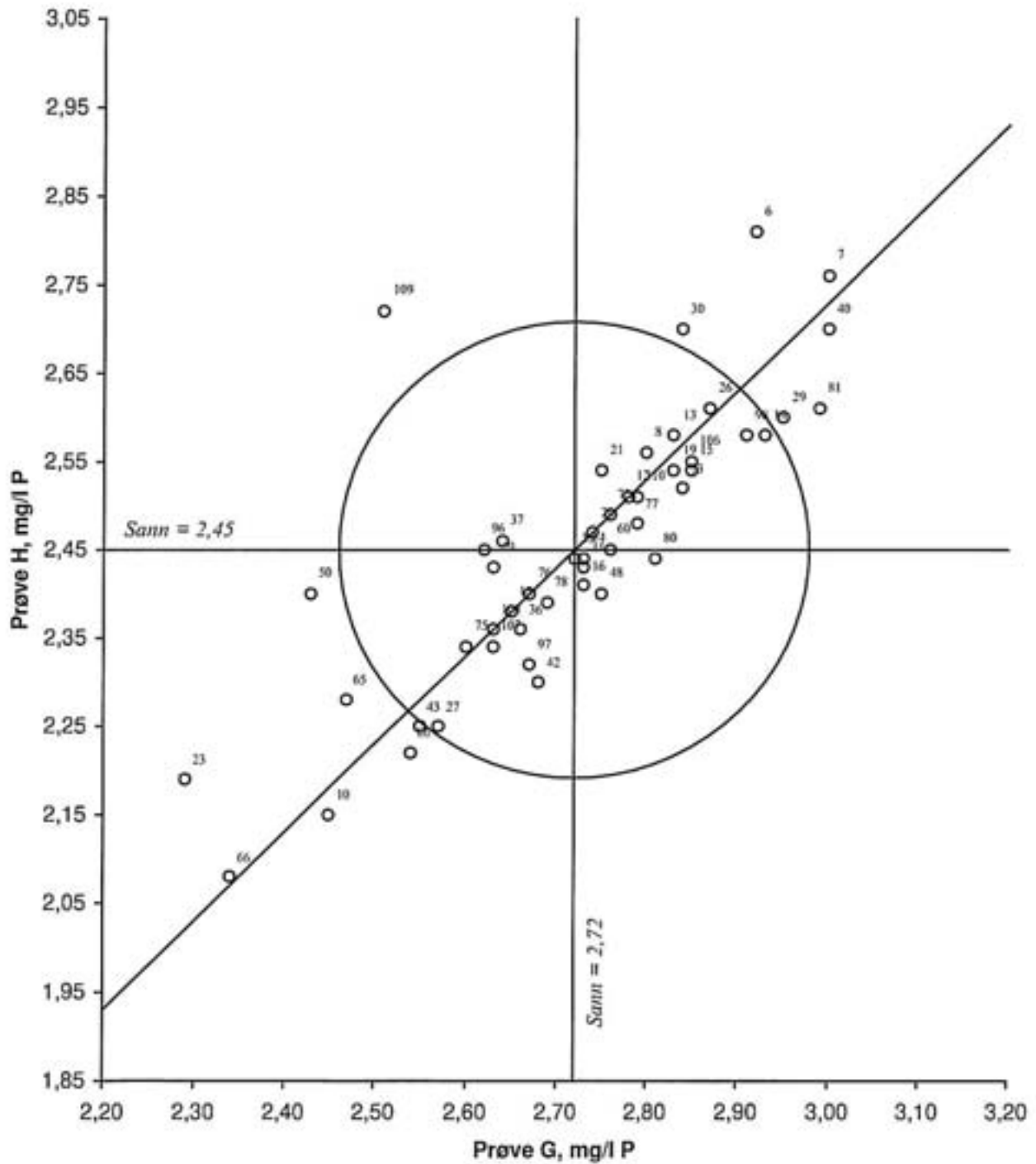
Figur 12. Youdendiagram for totalfosfor, prøvepar GH Akseptansesgrensen, angitt med en sirkel, er 10 %
