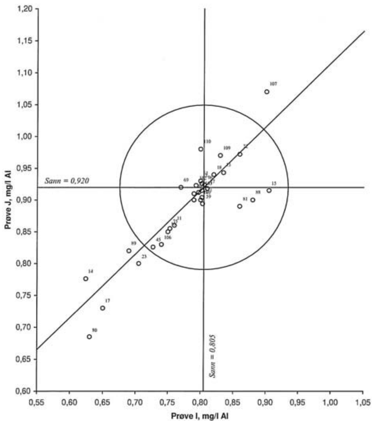
Figur 15. Youdendiagram for aluminium, prøvepar IJ Akseptansgrensen, angitt med en sirkel, er 15 %
