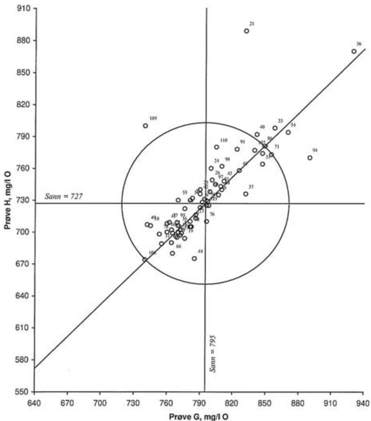
Figur 8. Youdendigram for kjemisk oksygenforbruk, \text{COD}_{\text{Cr}} , prøvepar GH. Akseptansesegrensen, angitt med en sirkel, er 10 %.
