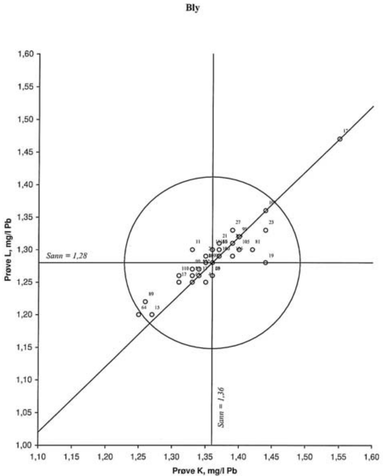
Figur 18. Youdendiagram for bly, prøvepar KL Akseptansegrensen, angitt med en sirkel, er 10 %
