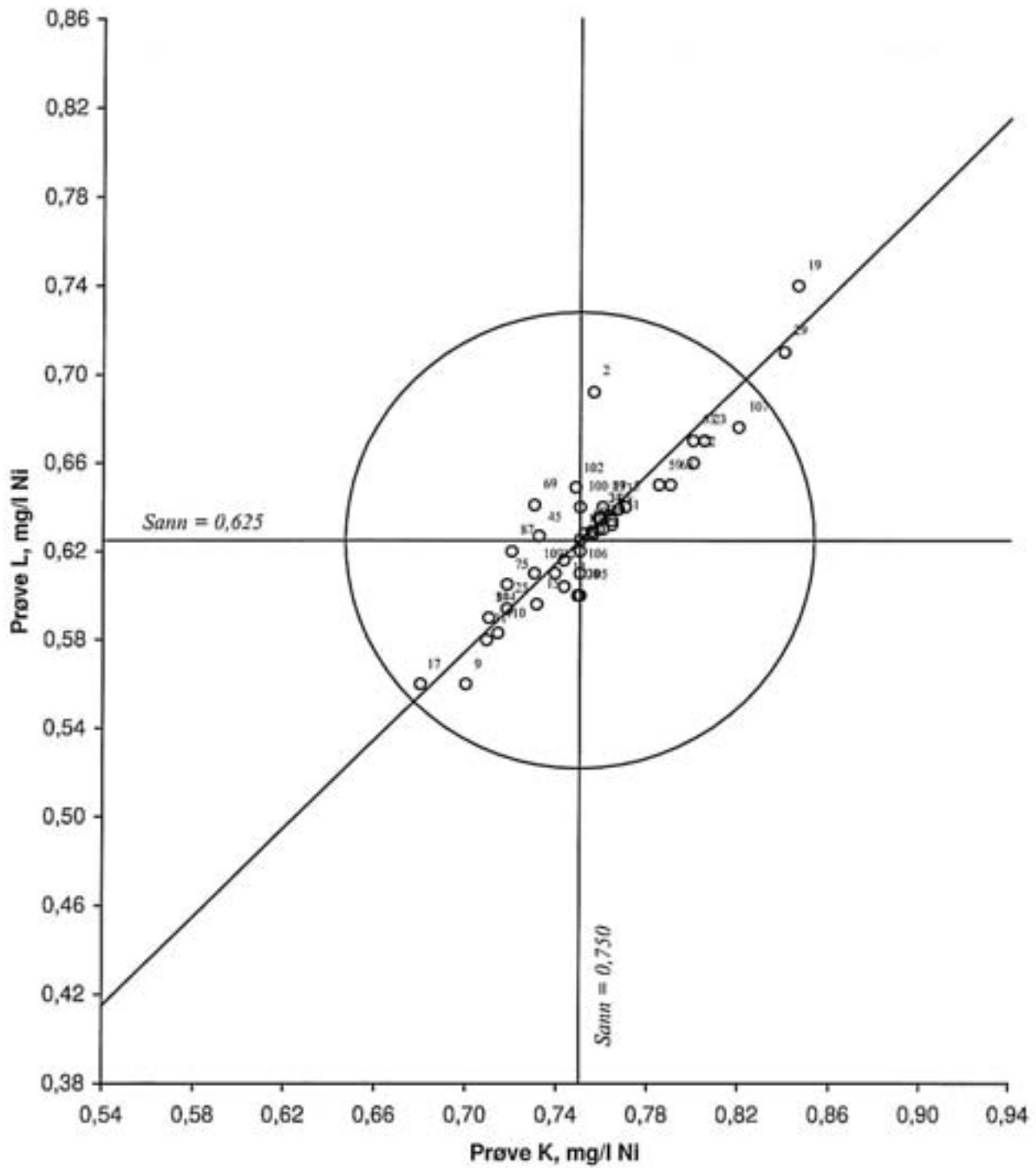
Figur 30. Youdendiagram for nikkell, prøvepar KL Akseptansesegrensen, angitt med en sirkel, er 15 %
