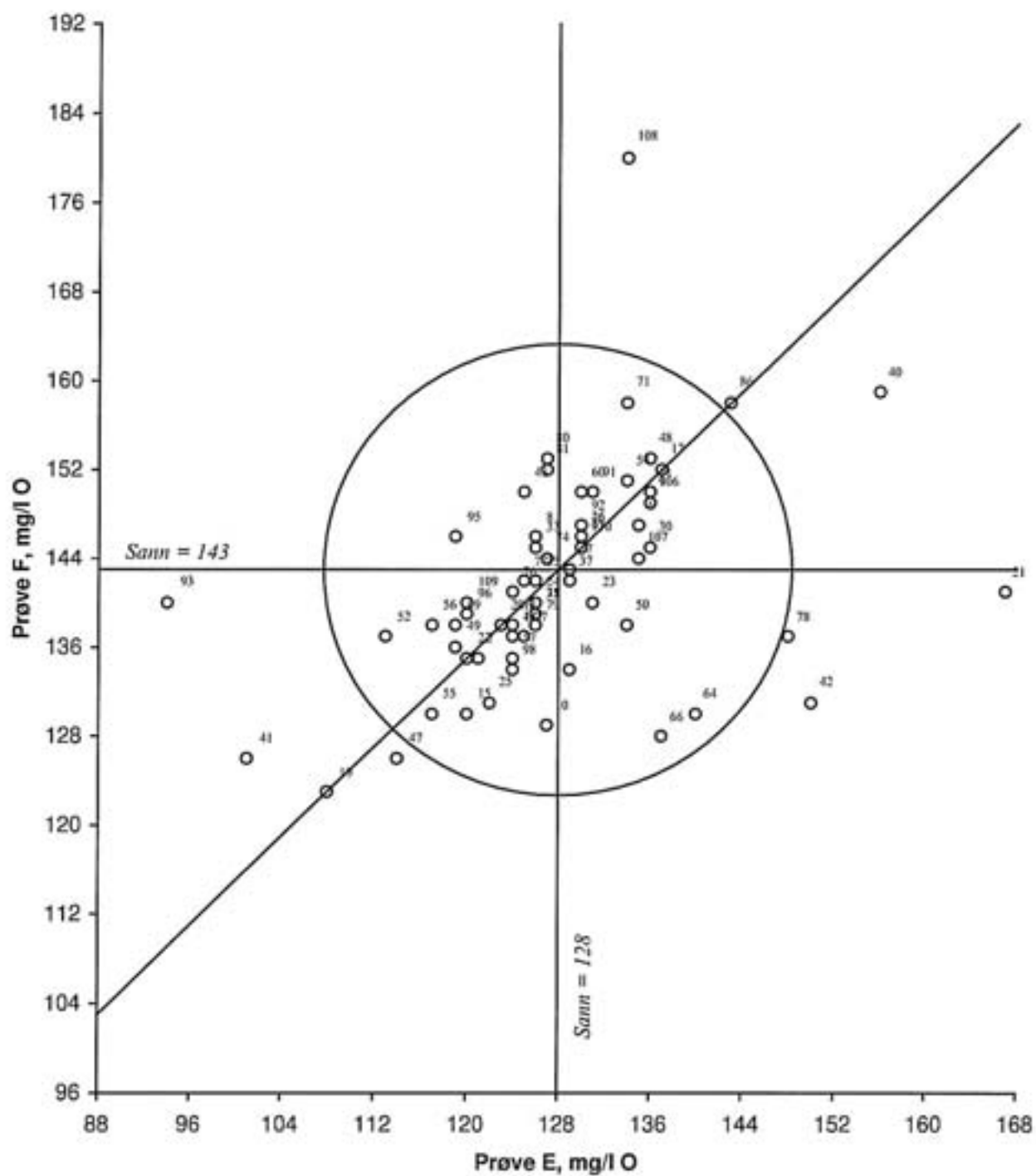
Figur 7. Youdendigram for kjemisk oksygenforbruk, \text{COD}_{\text{Cr}} , prøvepar EF. Akseptansesegrensen, angitt med en sirkel, er 15 %
