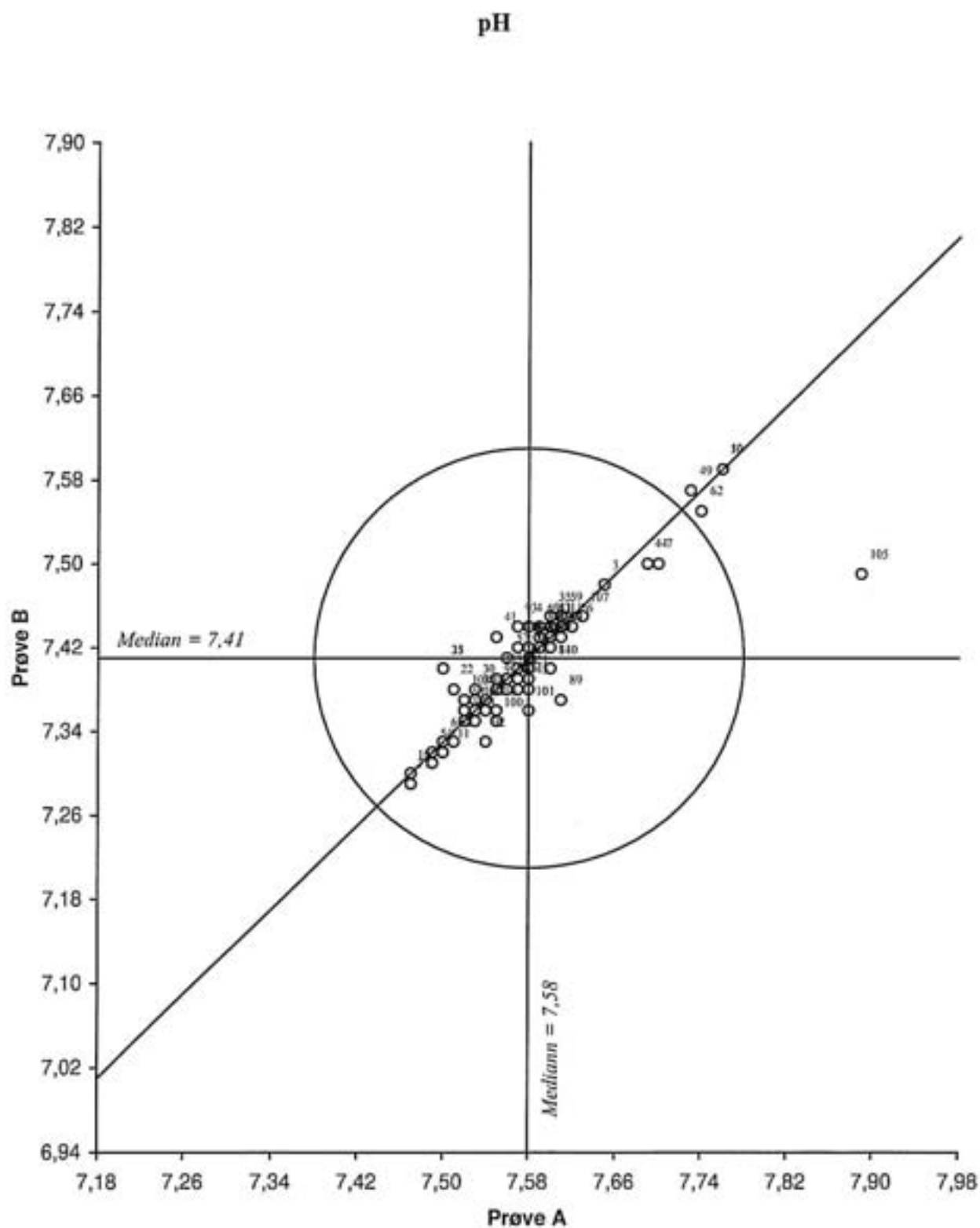
Figur 1. Youdendiagram for pH, prøvepar AB Akseptansesgrensen, angitt med en sirkel, er 0,2 pH-enhet
