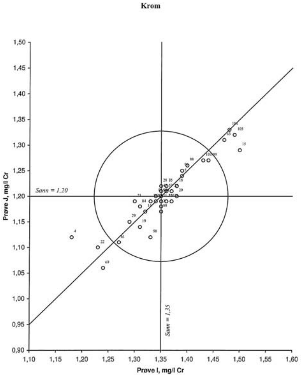
Figur 25. Youdendiagram for krom, prøvepar IJ Akseptansegrensen, angitt med en sirkel, er 10 %
