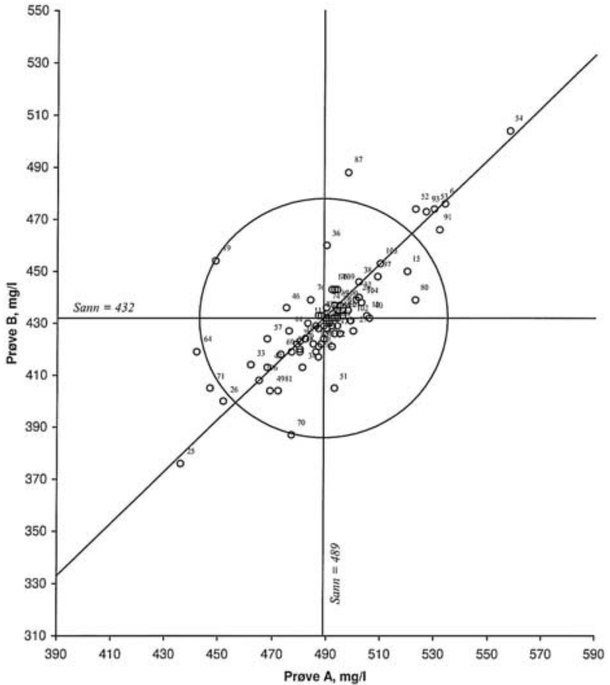
Figur 3. Youdendigram for suspendert stoff, tørrstoff, prøvepar AB Akseptansgrensen, angitt med en sirkel, er 10 %
