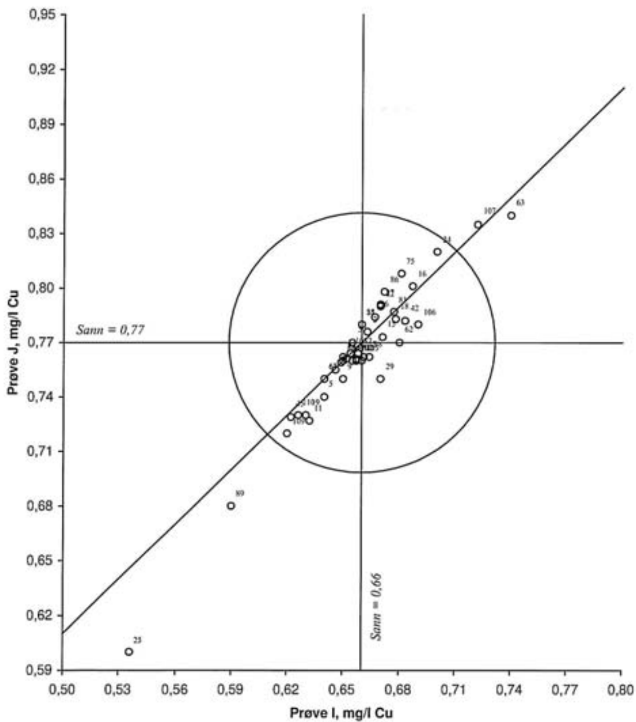
Figur 23. Youdendiagram for kobber, prøvepar IJ Akseptansgrensen, angitt med en sirkel, er 10 %
