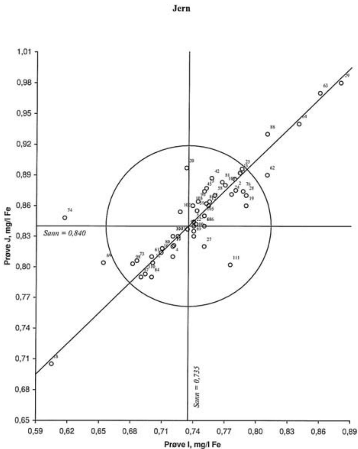
Figur 19. Youdendiagram for jern, prøvepar IJ Akseptansesgrensen, angitt med en sirkel, er 10 %
