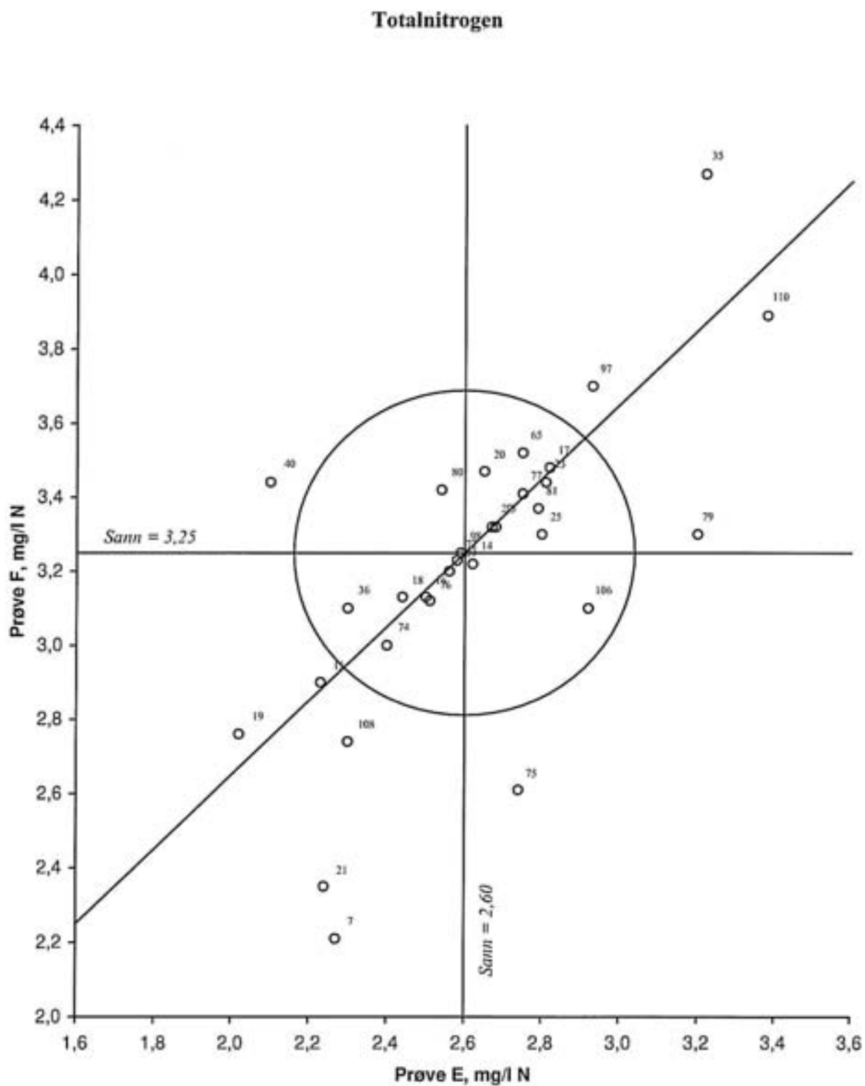
Figur 13. Youdendiagram for totalnitrogen, prøvepar EF Akseptansesgrensen, angitt med en sirkel, er 15 %
