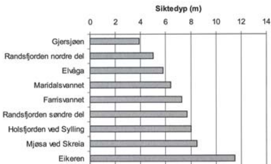
Figur 5-2 Siktedyp i søndre del av Holsfjorden sammenliknet med en del andre innsjøer som er sentrale i drikkevannssammenheng. Gjersjøen 1997 (Faafeng og Oredalen 1998), Randsfjorden 1997 (Løvik og Røgnerud 1998), Elvåga og Maridalsvannet 1994 (Wold 1995), Eikeren 1997 (Berge og Brettum 1999), Holsfjorden ved Sylling 1979-81 (Berge og medarb 1985).
