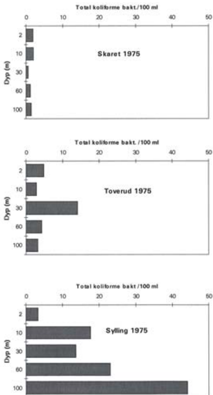
Figur 9-4 Middelerverdier av total koliforme bakterier ved de angitte stasjoner fra SIFF's undersøkelser i 1975 (Myhrstad 1976).
