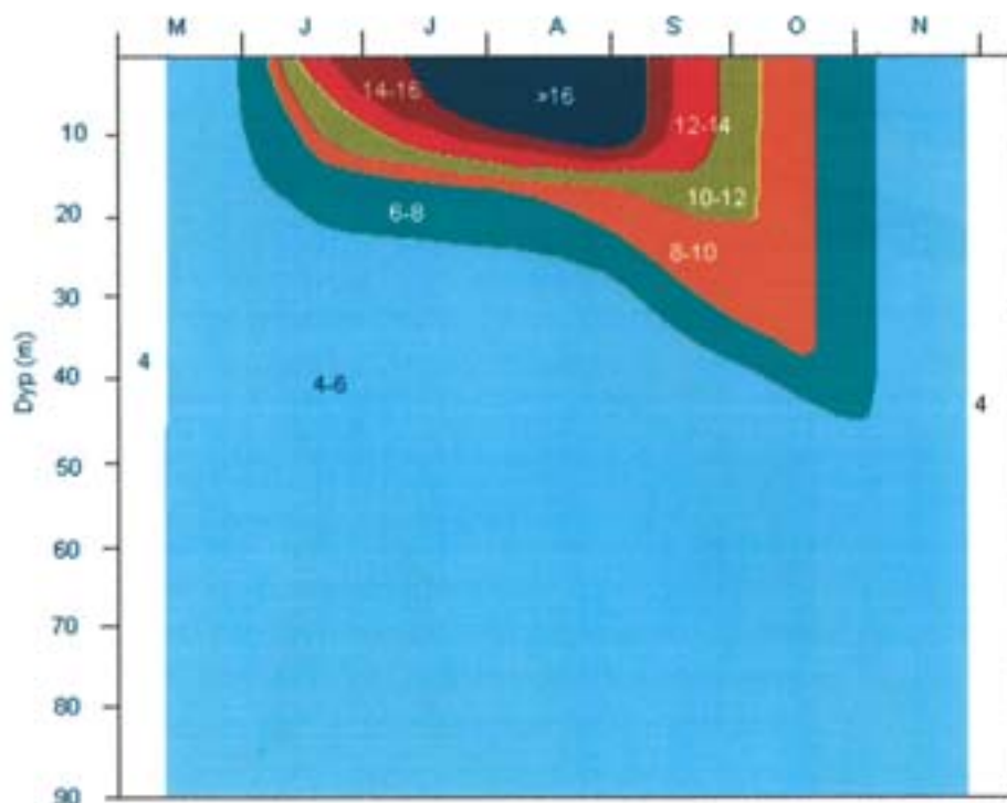
Figur 4-1 Temperaturforholdene i Tyrifjorden i sommerhalvåret fra overflaten og ned til 90m dyp, °C (fra Berge 1981).
