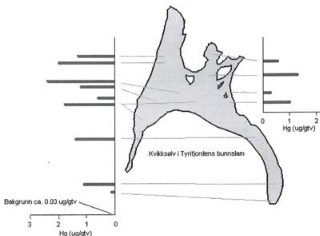
Figur 14-1 Middelkonsentrasjonen av kvikksølv i det forurensede sedimentsjikt på forskjellige steder i Tyri-fjorden (etter Berge og medarb 1983)
