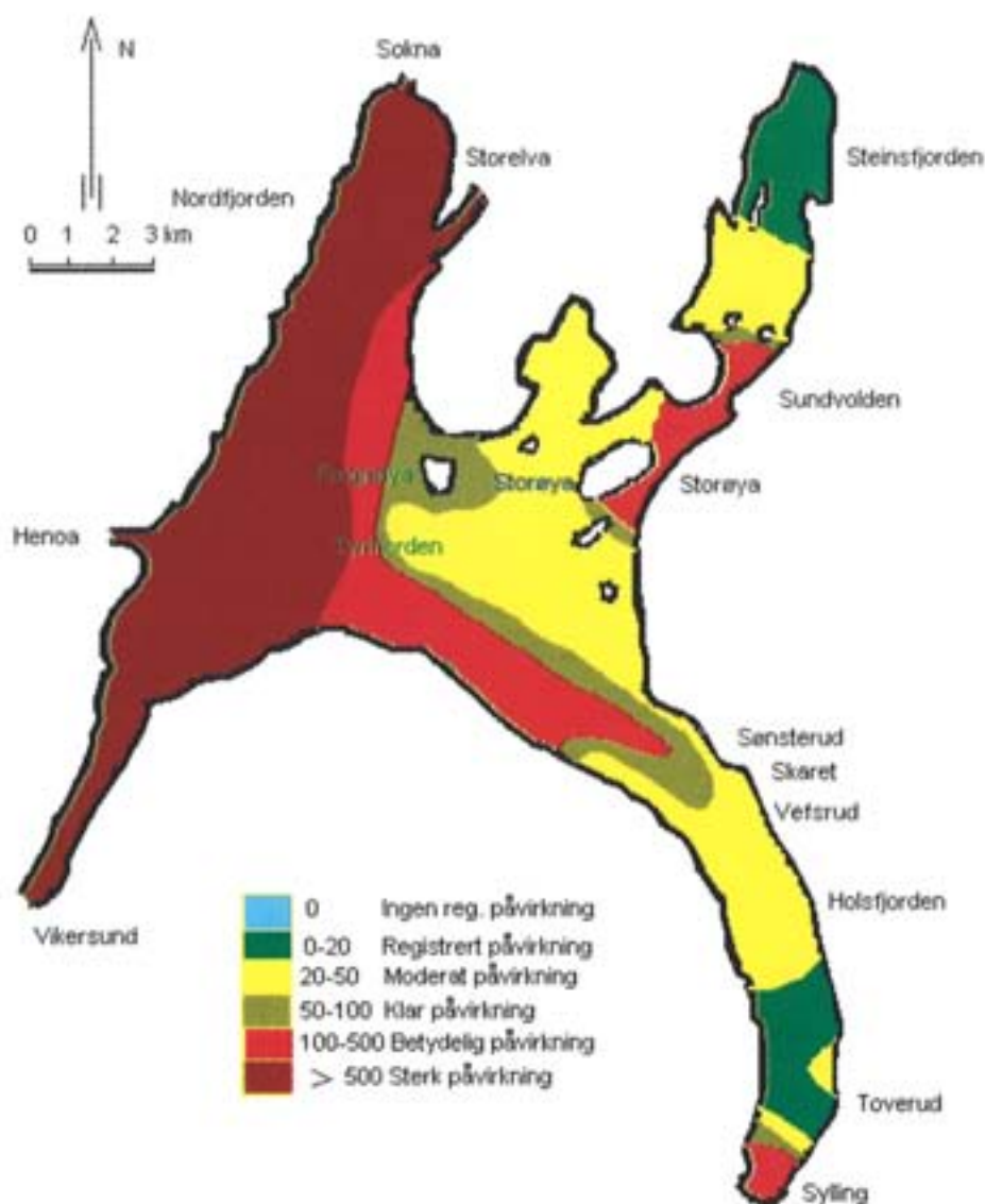
Figur 7-2 Midlere konsentrasjon (antall/l) av total koliforme bakterier (37 °C) i overflatesjiktet 0-30m under sommerstagnasjonen 1980. Etter Riise og Solberg (1983).
