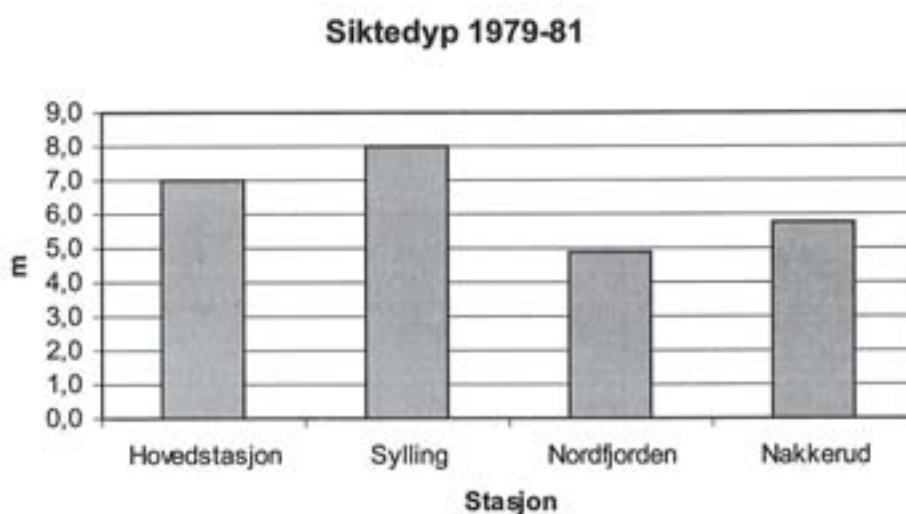
Figur 5-1 Siktedypet ved de ulike stasjoner i Tyrifjorden gitt som middelerdi av 36 observasjoner gjennom årene 1979-81 (fra Berge og medarb 1985).
