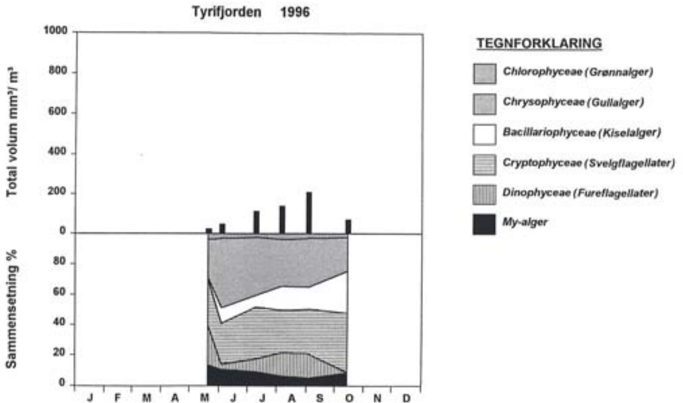
Figur 10-5 Algevolum og sammensetning av de viktigste hovedgrupper i algesamfunnet i Tyrifjorden fra 1996 (Bratli og medarb 1998).
