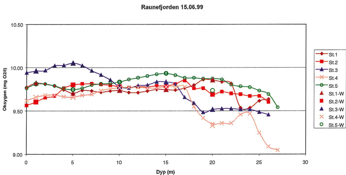
Figur 5. Oksygenprofiler 15. juni 1999.
