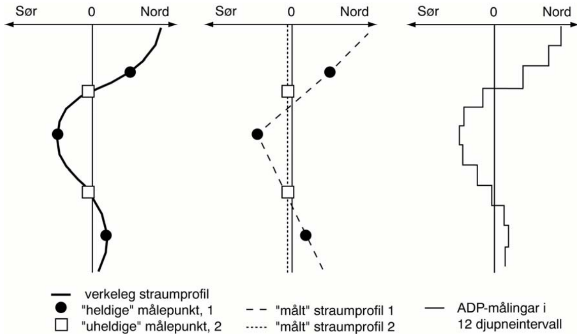
Figur 4. Prinsippsskisse som syner "sant" strømsprofil og "målte" profiler basert på ulike antal målepunkt i vertikalen, og ulik plassering av desse. Dersom måledjupa (eller målecellene for ein ADP) fell saman med sjikt der strømmen er sterkast, vil ein kunne få eit godt bilete av tilhøva, mens måling berre i sjikt med svak strøm vil gi eit feil bilete. Med fleire målepunkt eller djupneceller tilnærmar målt profil seg til "sant" profil.
