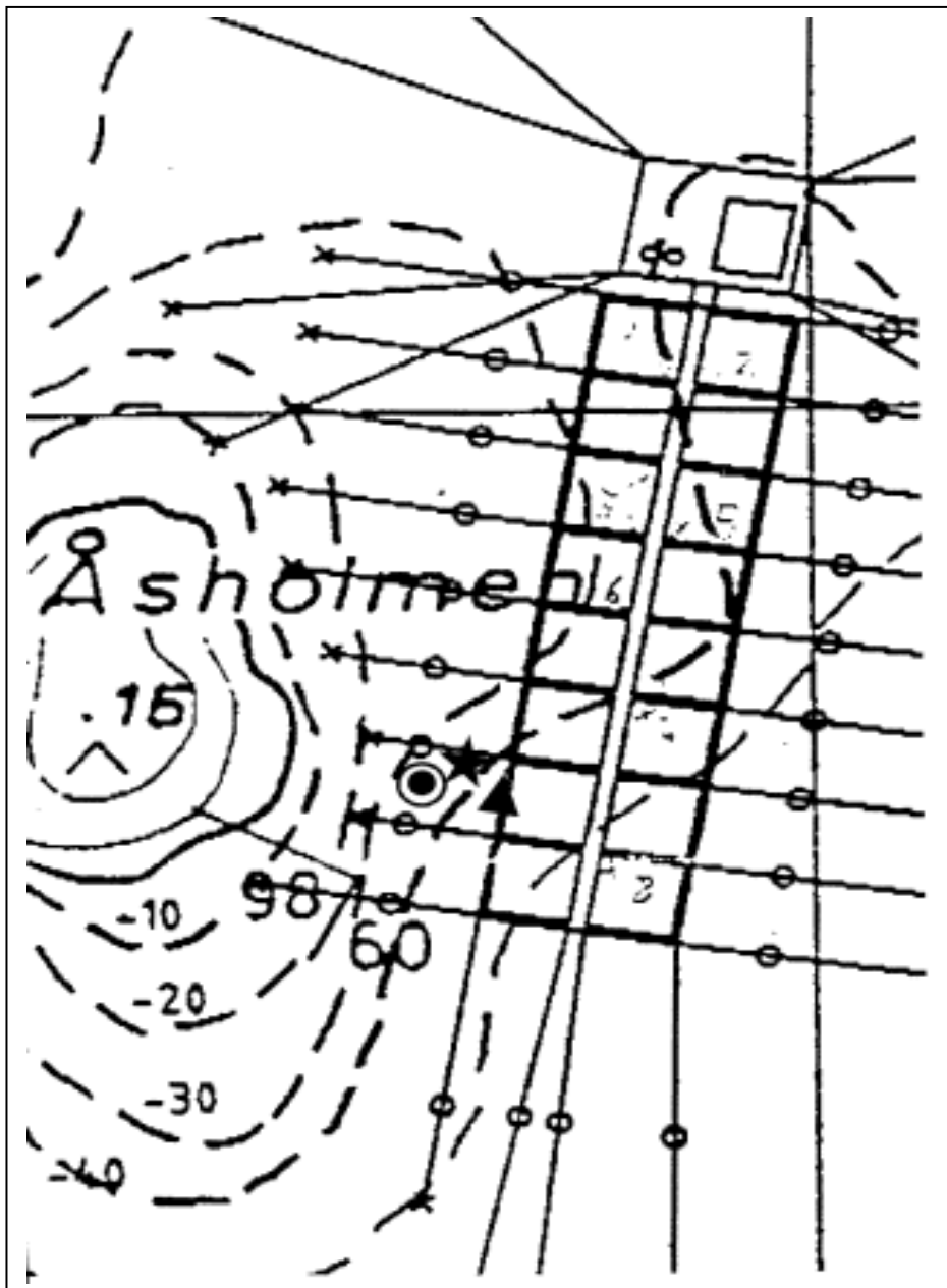
Figur 2. Forstørret kartskisse av anlegget. Måleposisjon for strømmåling i januar 1999, er avmerkt. \sigma : Aanderaa RCM og Sensordata SD6000 ca 3 m frå kvarandre, på merdkanten, H: Aanderaa RCM nær botn, \lambda : NORTEK ADP Doppler målar i ramme nær botn.
