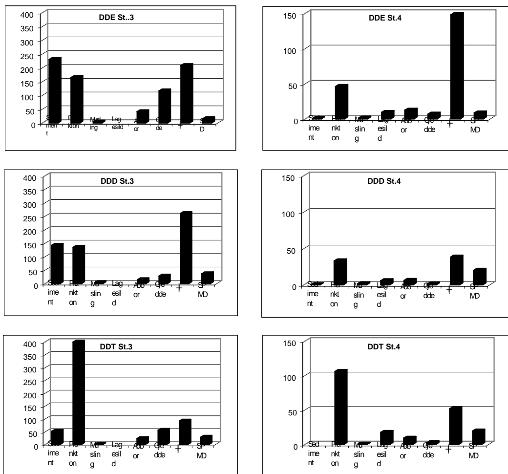
Figur 8. Konsentrasjoner av DDE, DDD og DDT i µg/kg tørrvekt for sedimenter, dyreplankton, abbor, ål, gjedde, lagesild, andemusling og triolein (SPMD) fra Ørsjøen.
