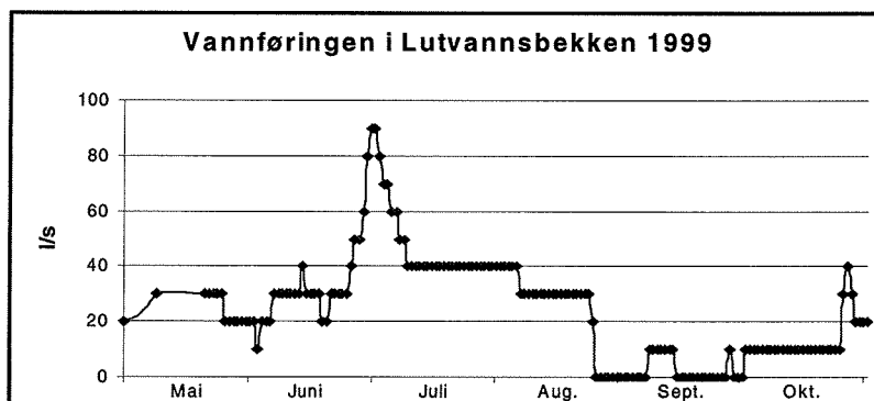
Fig. 3 Variasjoner i vannstand i Søndre og Nordre Puttjern og vannføringen i Puttjernsbekken (P1) og Lutvannsbekken (L0) i 1999.
