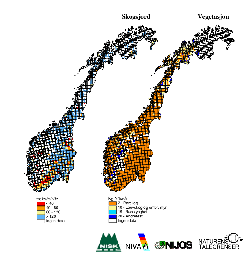
Figur 2. Tålegrenser for overgjødning av vegetasjon med nitrogen (Esser og Tomter 1996) basert på empiriske verdier, og tålegrenser for skogsjord i Norge beregnet med MAGIC-modellen (Frognér et al. 1994).
