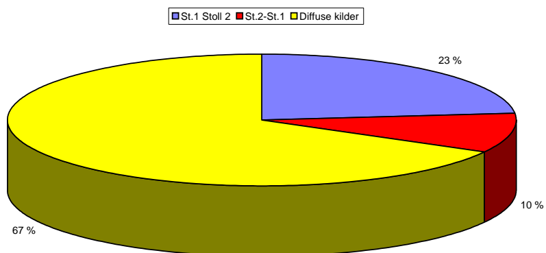
Figur 13. %-vis fordeling av sulfattransport på de enkelte kilder i 1999.
