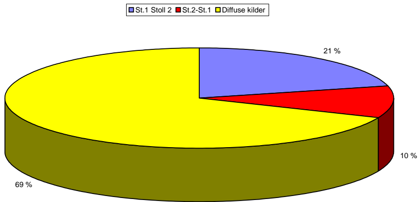
Figur 11. %-vis fordeling av sinktransport på de enkelte kilder i 1999.
