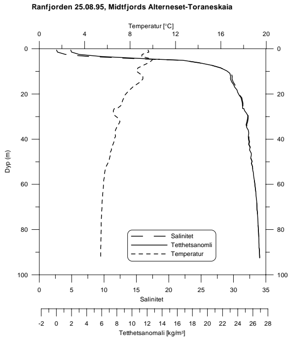
Figur 11. Hydrografimålinger 26.08.95 (forts.).
