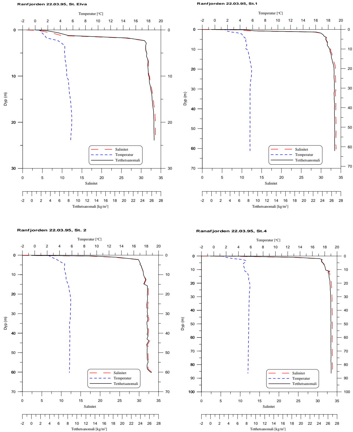
Figur 8. Hydrografimålinger 22.03.95.
