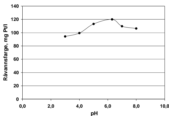
Figur 1. Fargetallet i råvannet ved ulike pH.
