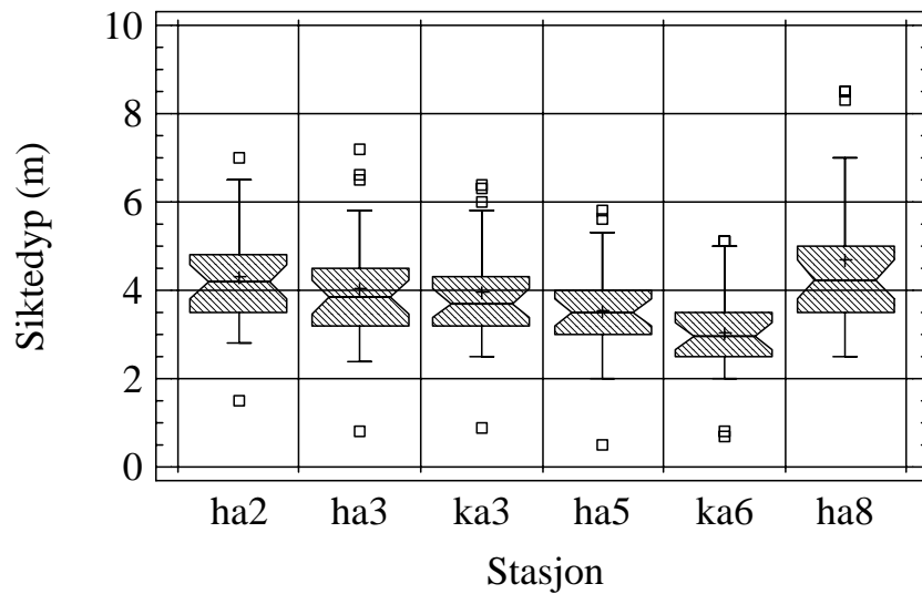
Figur 16. Siktedyp i juni-august på ulike stasjoner i havnebassenget 1999-2000. (observasjoner en gang pr. uke). Data fra overvåkingsprogrammet for indre Oslofjord
