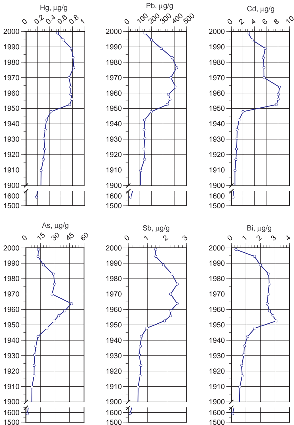
Figur 6. Mensvatn, Grenland. Konsentrasjoner av Hg, Pb, Cd, As, Sb og Bi i daterte sedimentsjikt.
