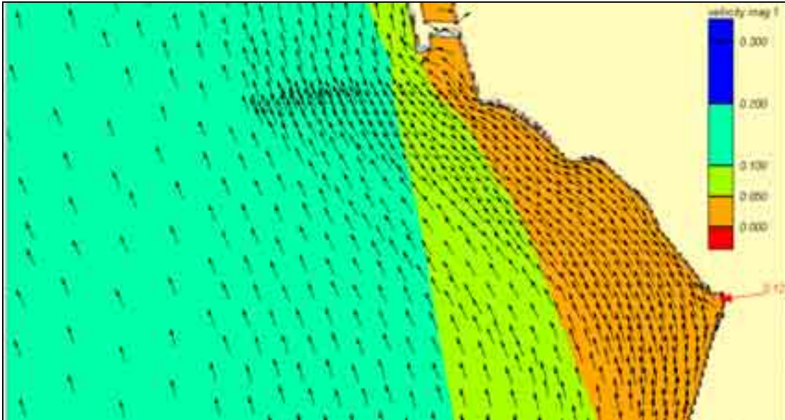
Figur 18. Scenario 1: Strømbilde (strømfart i m/s og strømpiler) for 0-2 m vannlag, uten betongmoloer og brygger. Tidevann strømmer nordover. Vannføring i bekken: 0.12 \text{ m}^3/\text{s} .
