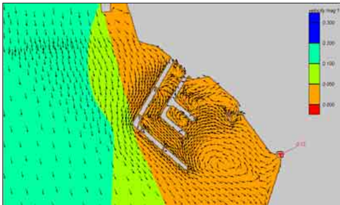
Figur 22. Scenario 5: Strømbilde (strømfart i m/s og strømpiler) for 0-2 m vannlag, med ny betongmolo. Tidevann strømmer sørover. Vannføring i bekken: 0.12 m 3 /s.
