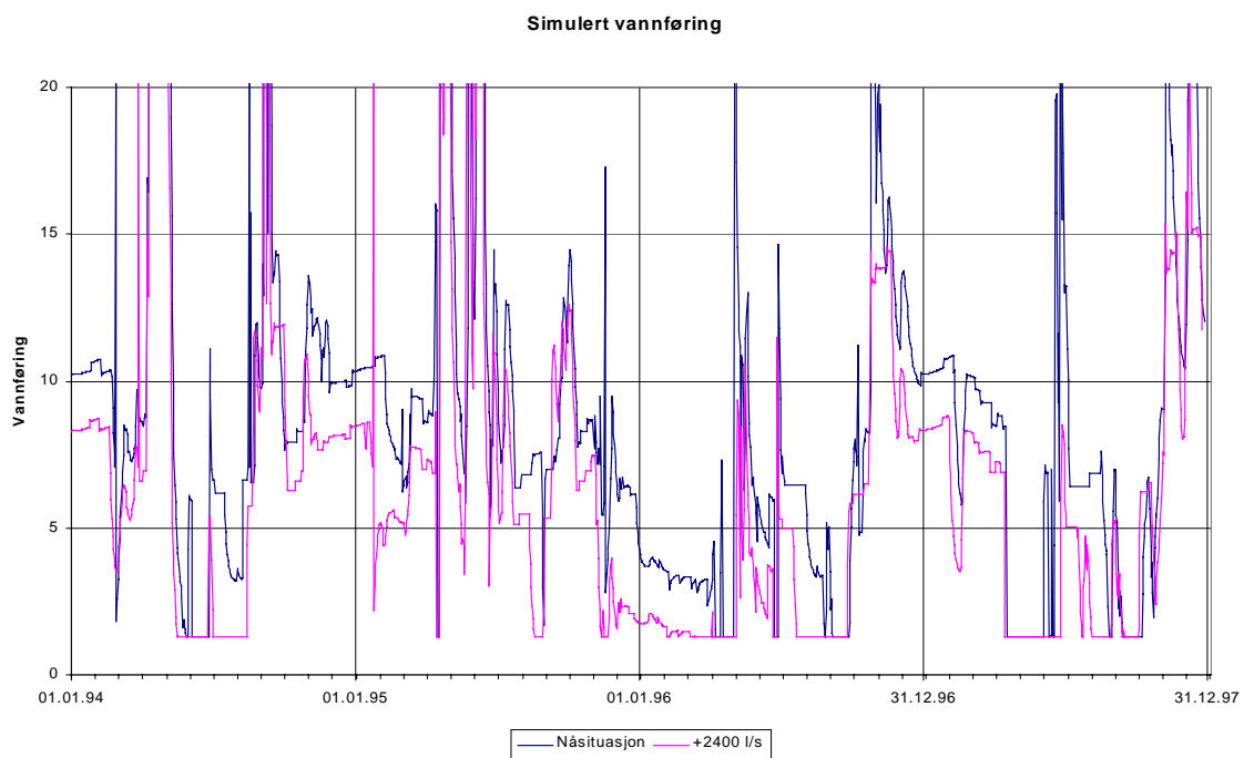
Figur 3.6 Konstant uttak, 2432 l/s, vannføring i Vestfosselva sammenlignet med "nåsituasjon".
