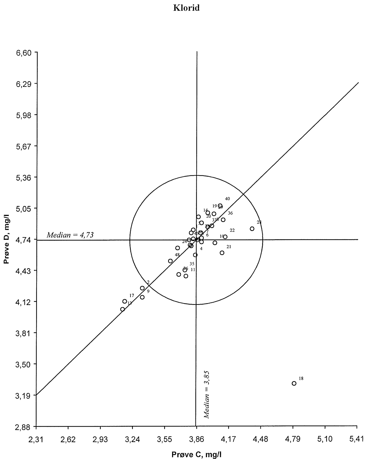
Figur 14. Youndendiagram for klorid, prøvepar CD Akseptansegrensen, angitt med en sirkel, er 15 %
