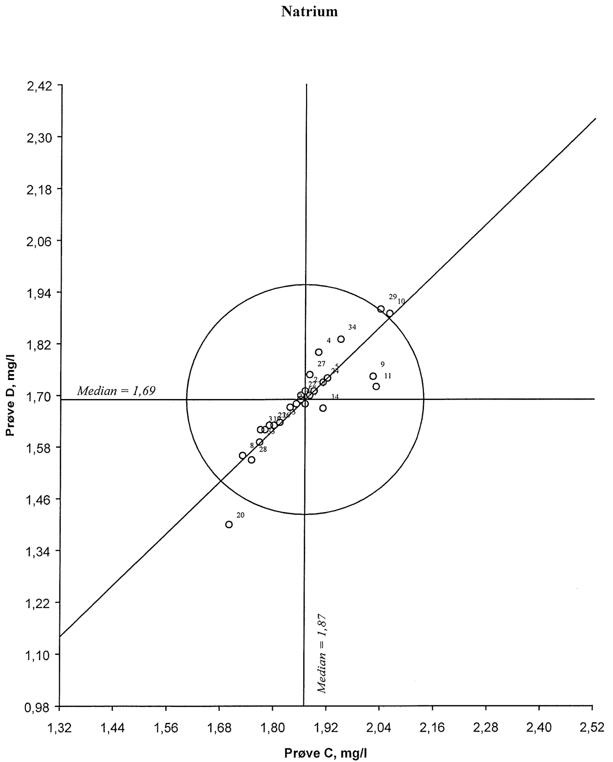
Figur 6. Youdendiagram for natrium, prøvepar CD Akseptansegrensen, angitt med en sirkel, er 15 %
