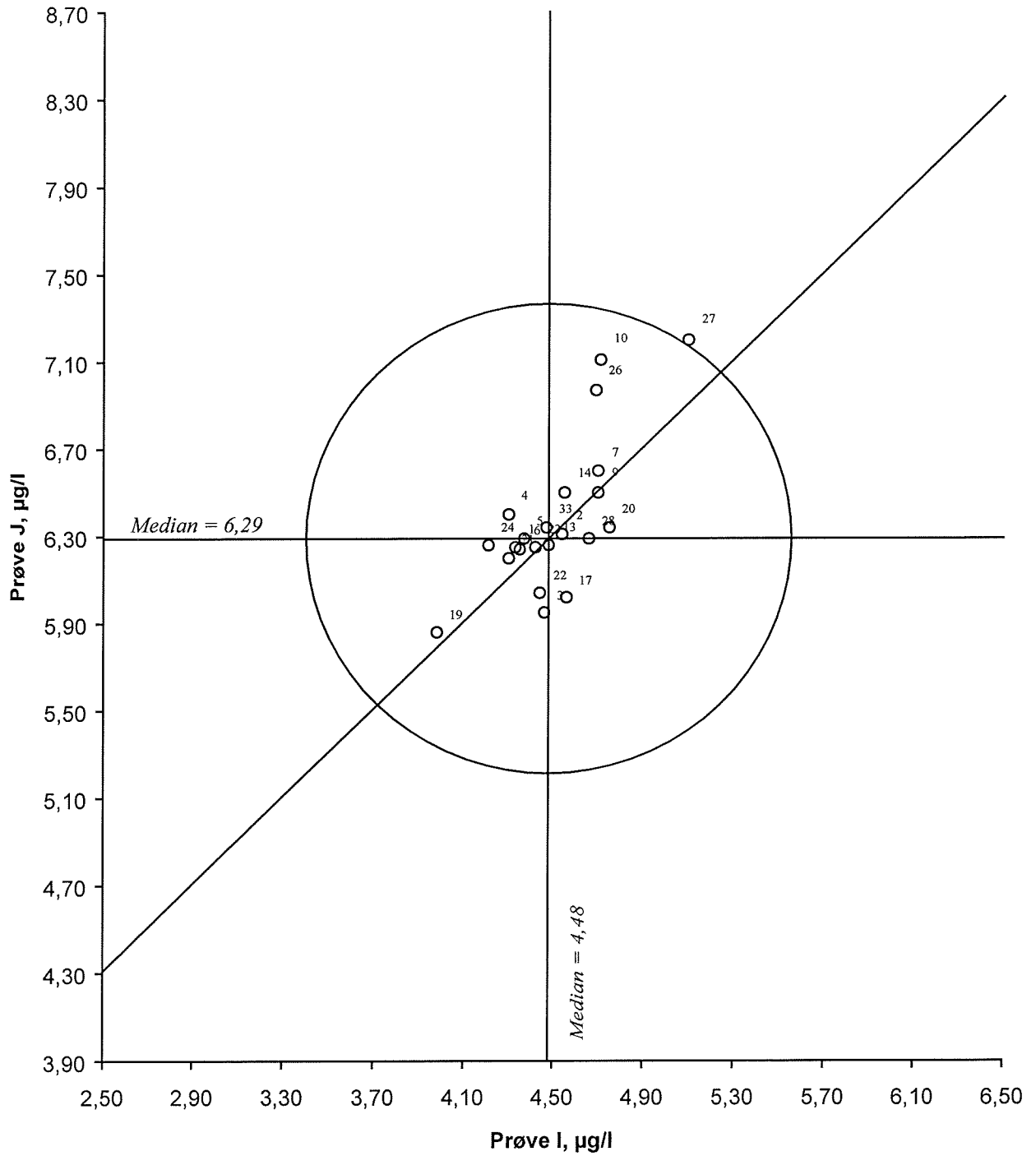
Figur 35. Youndendiagram for kadmium, prøvepar IJ Akseptansegrensen, angitt med en sirkel, er 20 %
