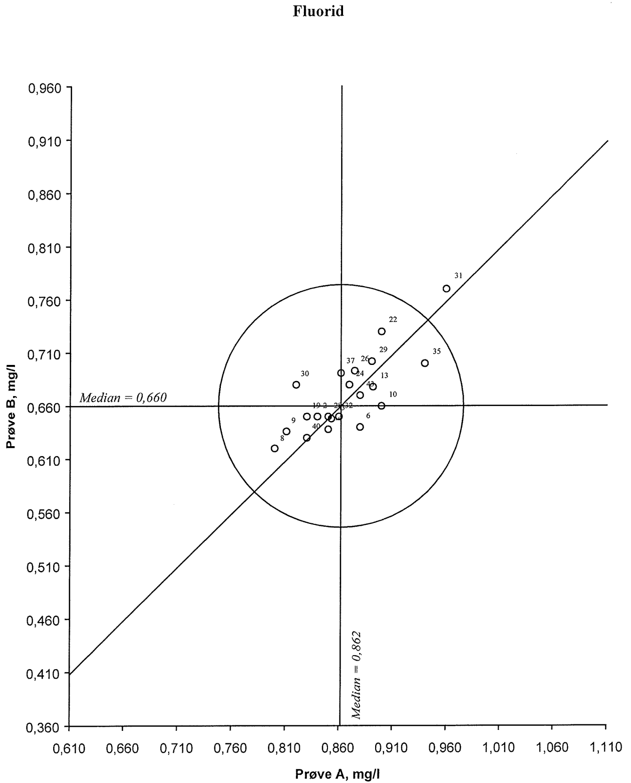
Figur 17. Youdendiagram for fluorid, prøvepar AB Akseptansegrensen, angitt med en sirkel, er 15 %
