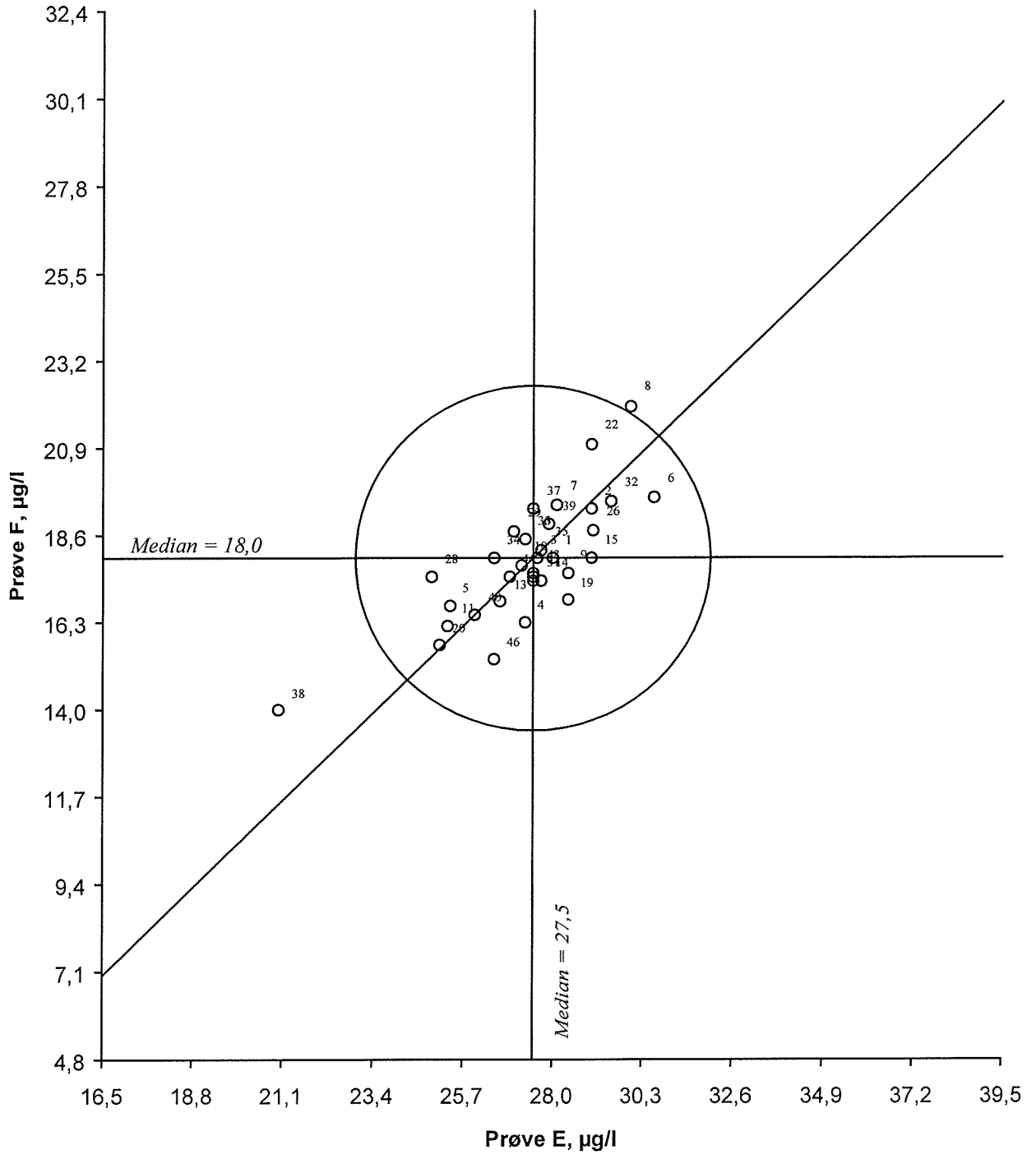
Figur 25. Youndendiagram for totalfosfor, prøvepar EF Akseptansegrensen, angitt med en sirkel, er 20 %
