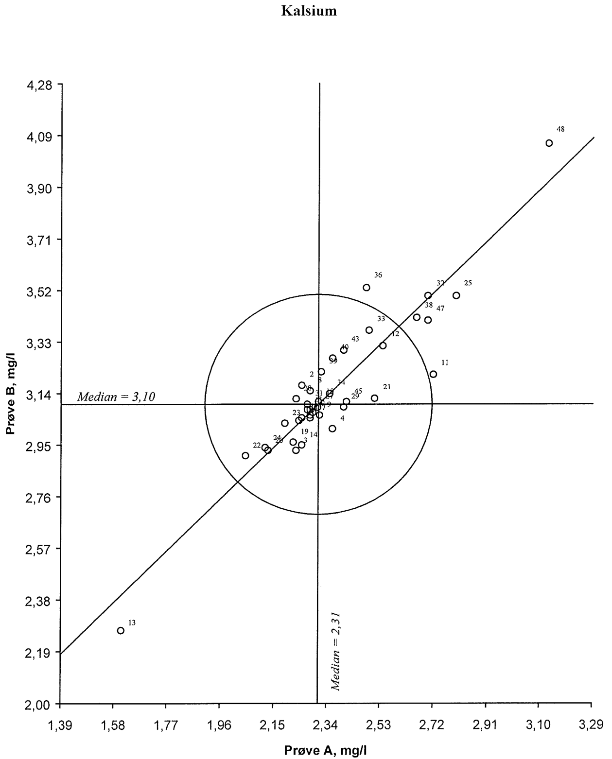
Figur 9. Youtendigram for kalsium, prøvepar AB Akseptansegrensen, angitt med en sirkel, er 15+F405 %
