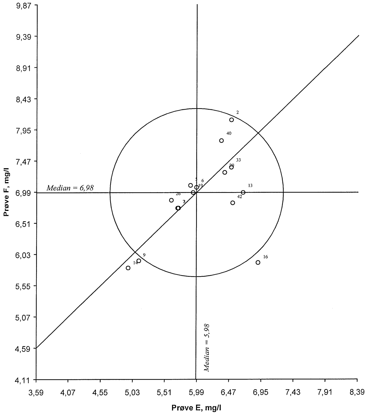
Figur 19. Youdendigram for totalt organisk karbon, prøvepar EF Akseptansegrensen, angitt med en sirkel, er 20 %
