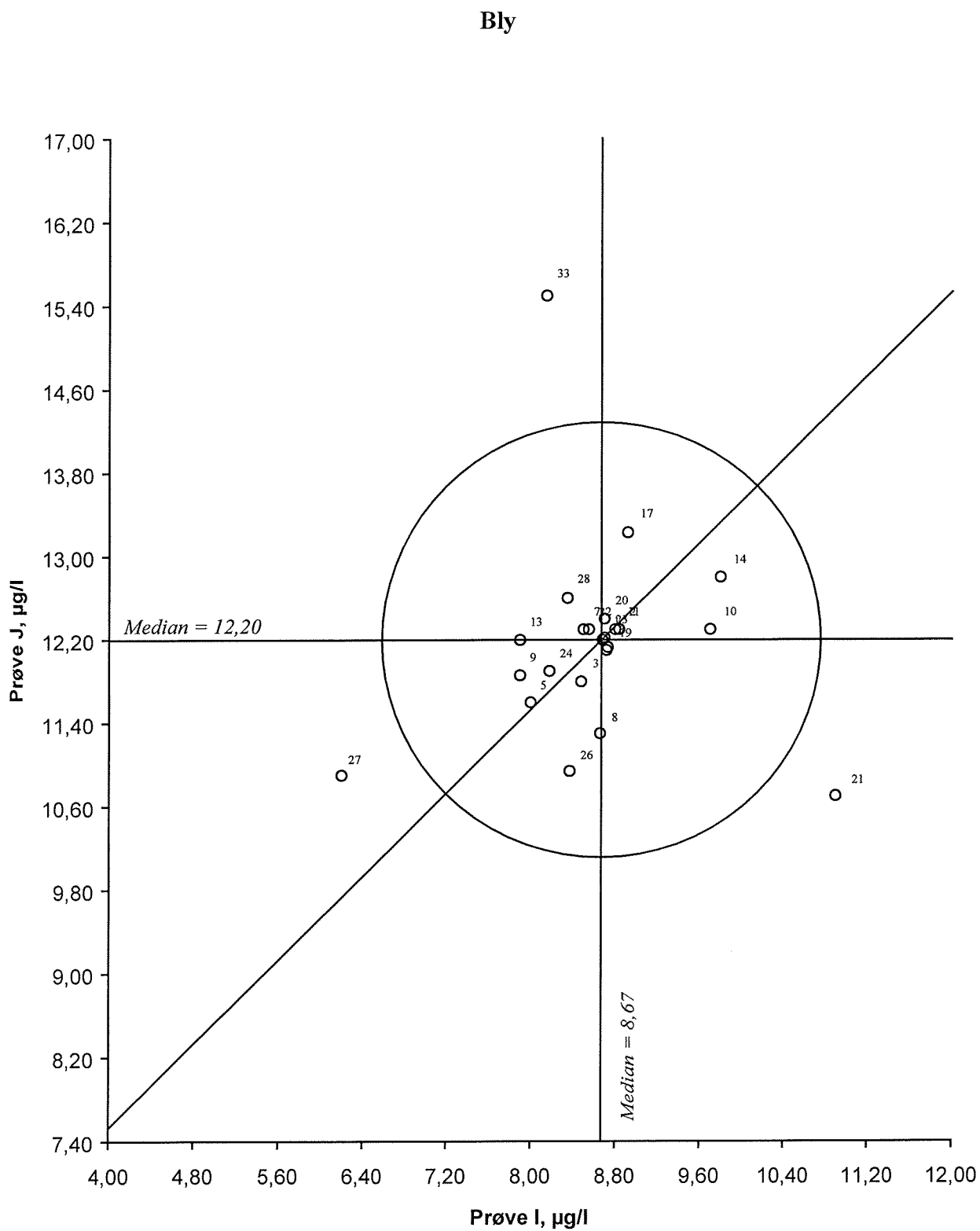
Figur 33. Youdendiagram for bly, prøvepar IJ Akseptansegrensen, angitt med en sirkel, er 20 %
