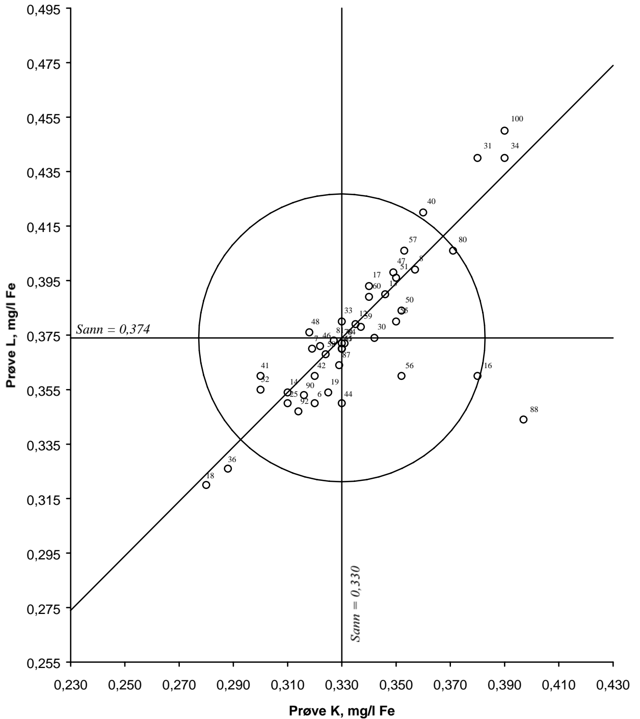
Figur 20. Youdendiagram for jern, prøvepar KL Akseptansegrensen, angitt med en sirkel, er 15 %
