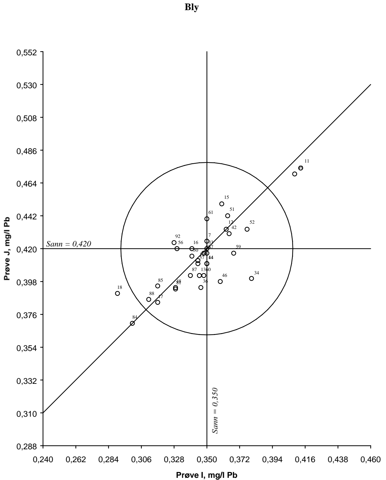
Figur 17. Youdendigram for bly, prøvepar IJ Akseptansegrensen, angitt med en sirkel, er 15 %
