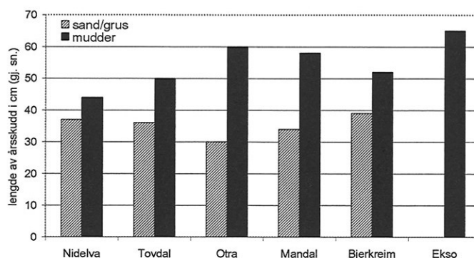
Figur 14. Typisk årsvekst av krypsiv i elver. Årsskuddene på mudder i stilleflytende områder er normalt lengre enn årsskuddene på sand og grus i strømløp. Basert på målinger av de 10 lengste årsskuddene for hver lokalitet. Snittverdier for periodene 1995-98 (Tovdal, Mandal), 1996-98 (Nidelva), 1996-97 (Bjerkreim, Ekso) og 1988-89 (Otra).
