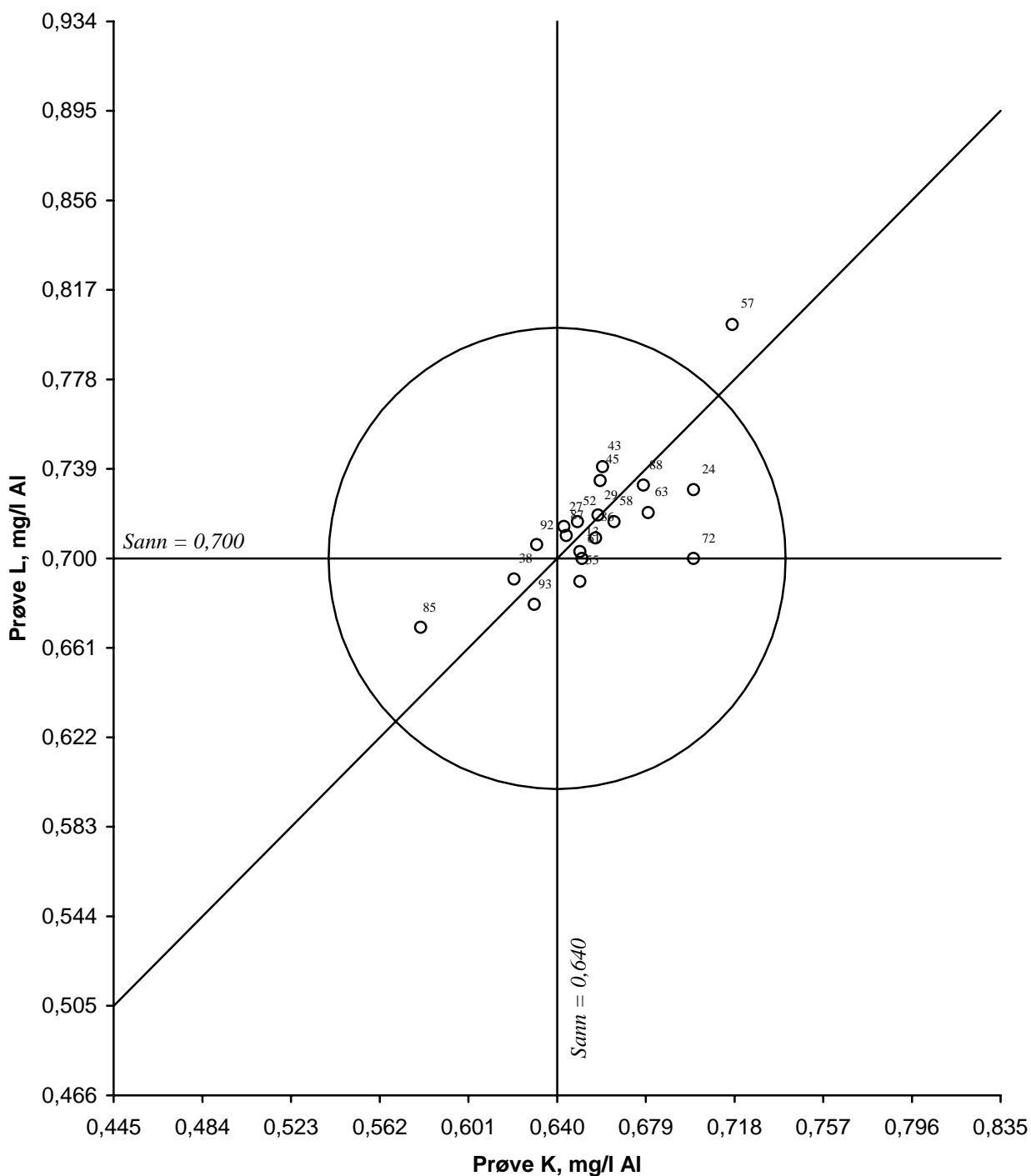
Figur 16. Youdendigram for aluminium, prøvepar KL Akseptansgrensen, angitt med en sirkel, er 15 %
