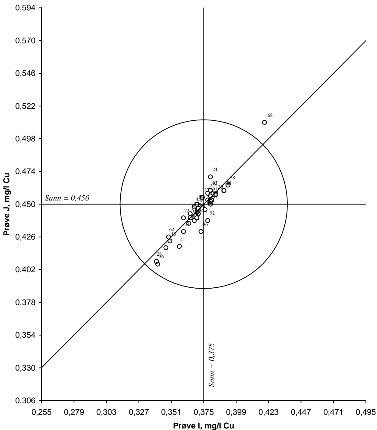
Figur 23. Youndendiagram for kobber, prøvepar IJ Akseptansgrensen, angitt med en sirkel, er 15 %
