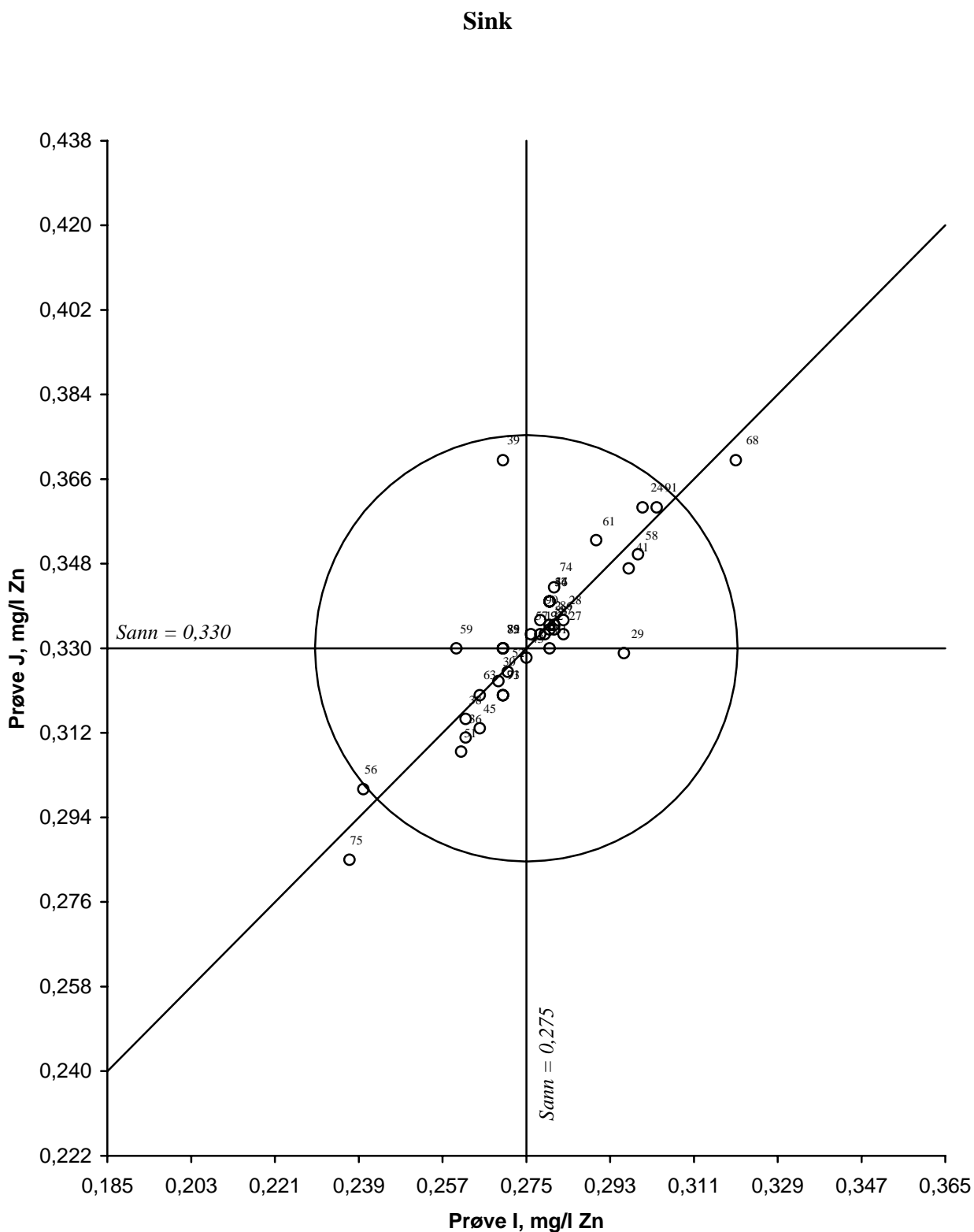
Figur 31. Youndendiagram for sink, prøvepar IJ Akseptansgrensen, angitt med en sirkel, er 15 %
