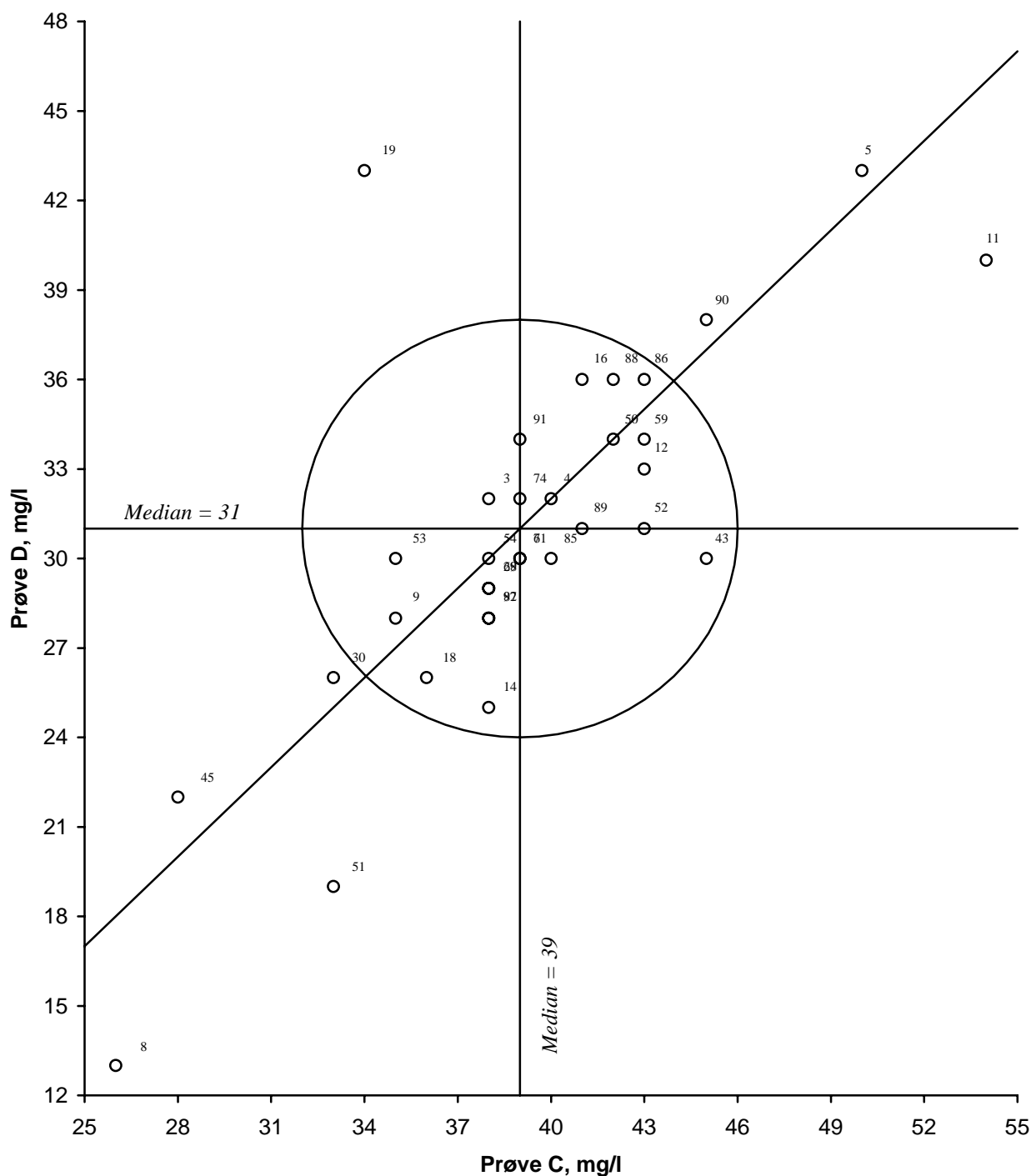
Figur 6. Youtendiagram for suspendert stoff, gløderest, prøvepar CD Akseptansgrensen, angitt med en sirkel, er 20 %
