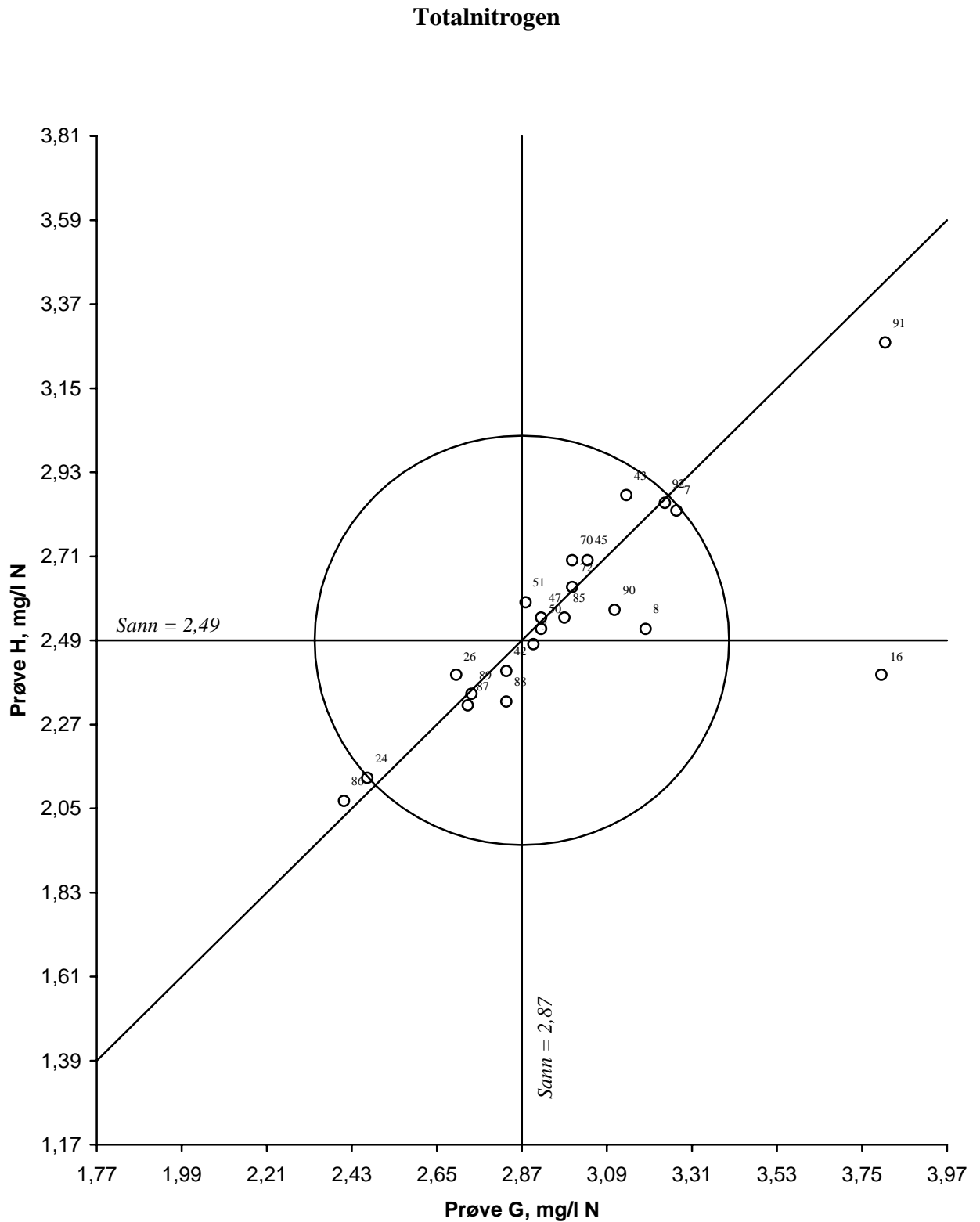
Figur 14. Youdendigram for totalnitrogen, prøvepar GH Akseptansegrensen, angitt med en sirkel, er 20 %
