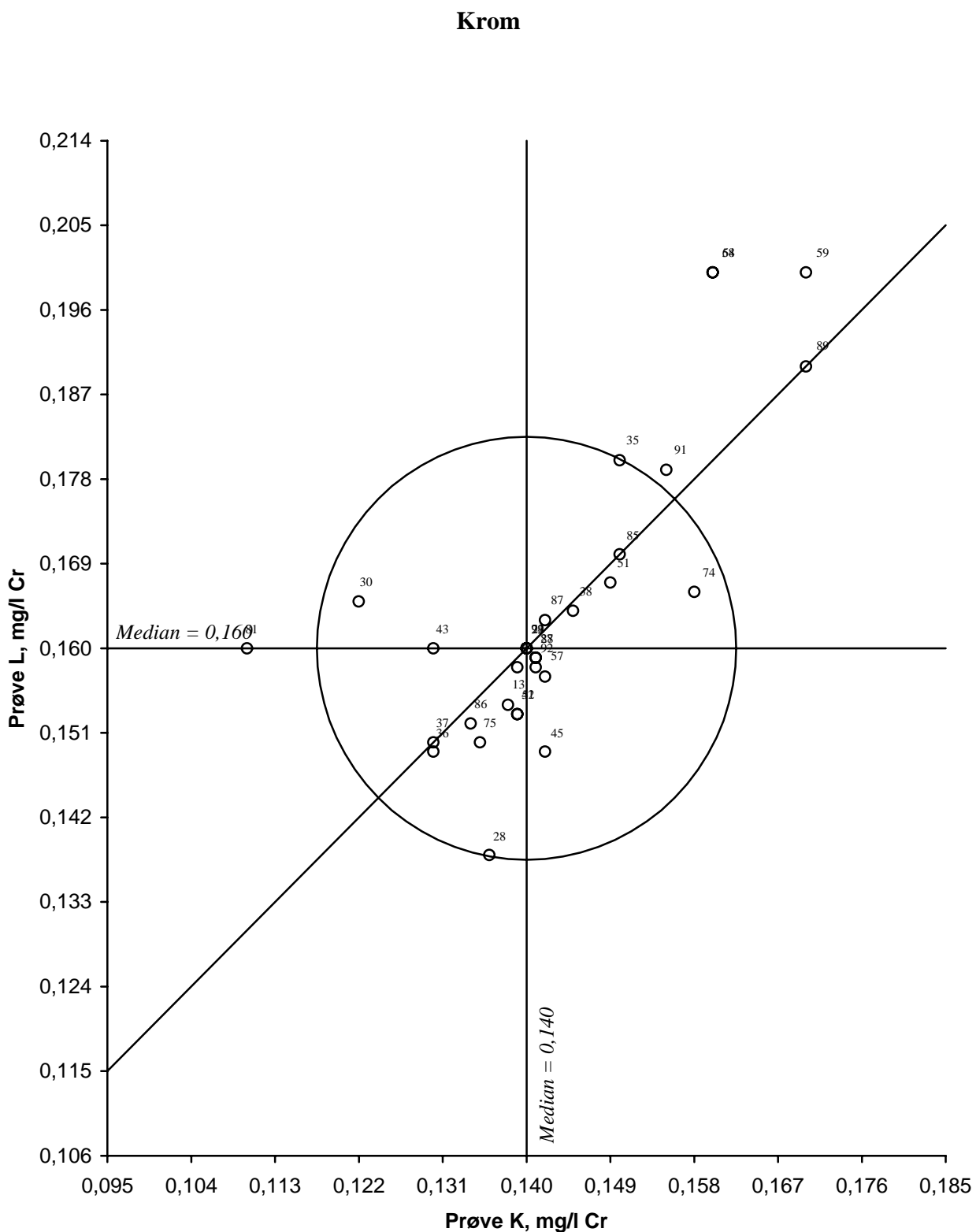
Figur 26. Youtenddiagram for krom, prøvepar KL Akseptansgrensen, angitt med en sirkel, er 15 %
