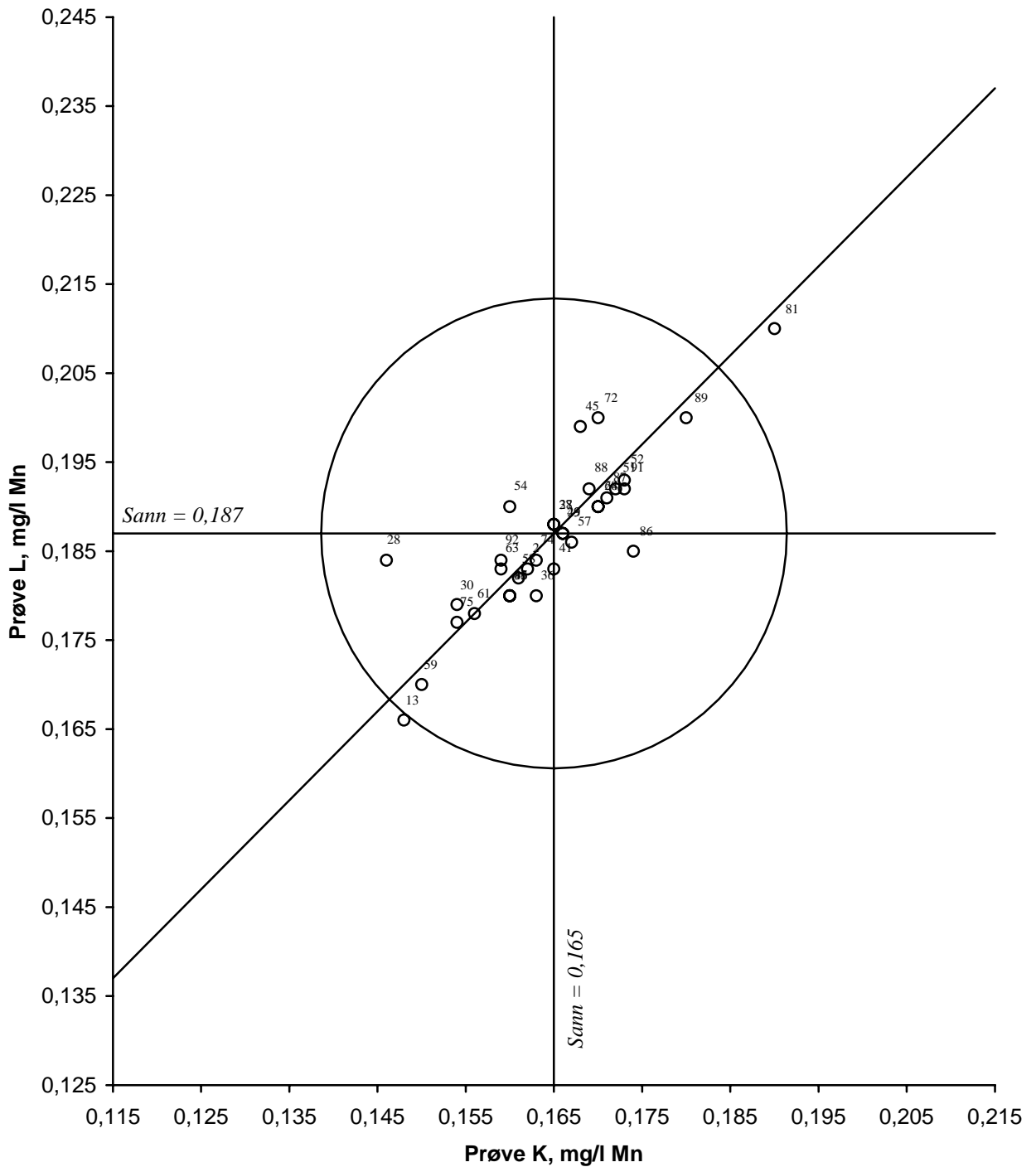
Figur 28. Youndendiagram for mangan, prøvepar KL Akseptansgrensen, angitt med en sirkel, er 15 %
