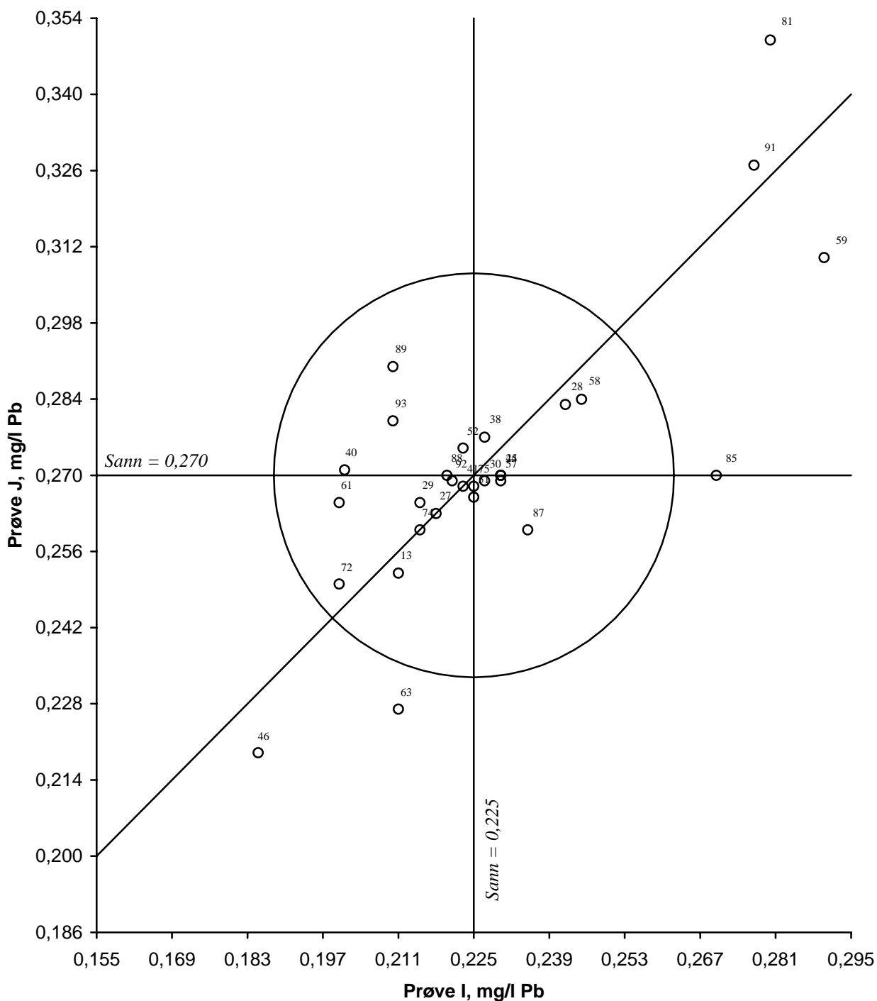
Figur 17. Youndendiagram for bly, prøvepar IJ Akseptansgrensen, angitt med en sirkel, er 15 %
