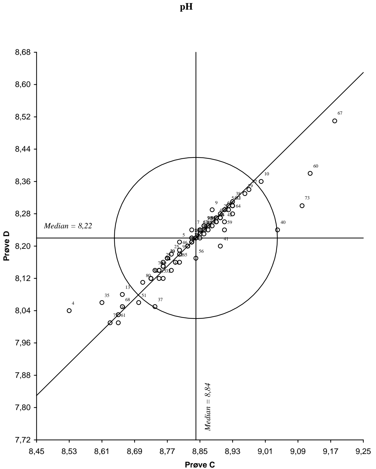
Figur 2. Youndendiagram for pH, prøvepar CD Akseptansgrensen, angitt med en sirkel, er 0,2 pH enheter
