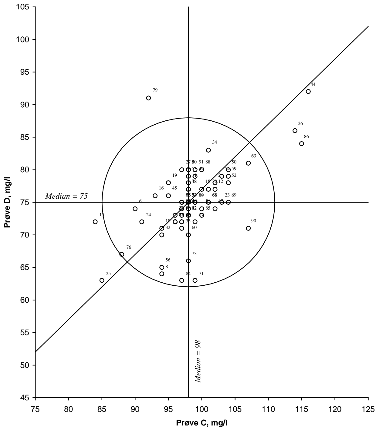
Figur 4. Youtendigram for suspendert stoff, tørrstoff, prøvepar CD Akseptansegrensen, angitt med en sirkel, er 15 %
