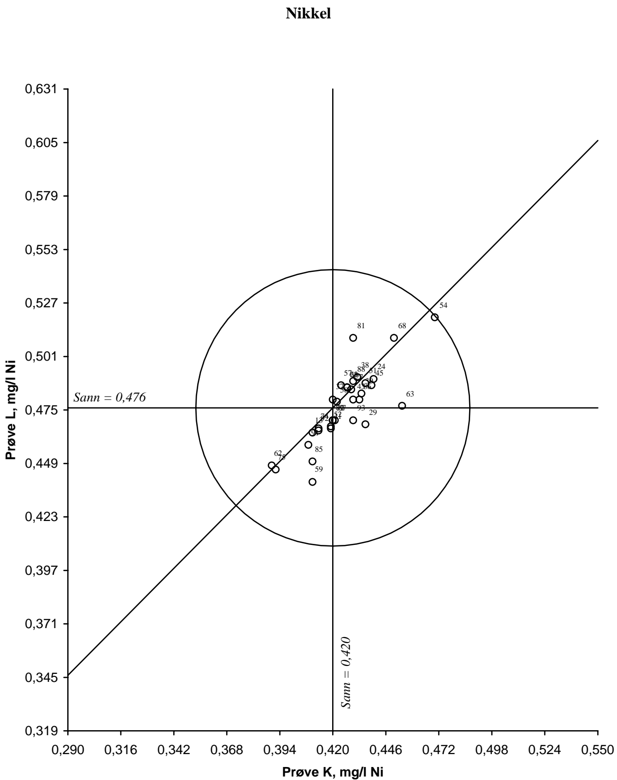
Figur 30. Youdendiagram for nikkel, prøvepar KL Akseptansesgrensen, angitt med en sirkel, er 15 %
