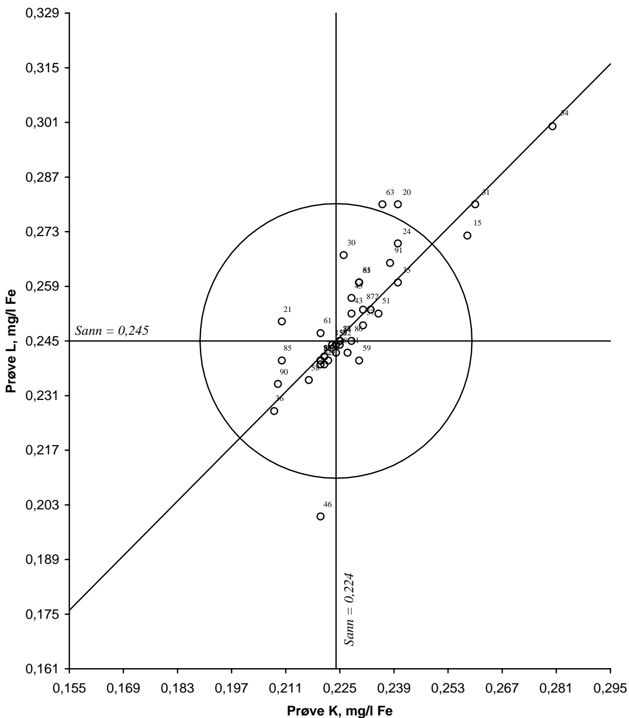
Figur 20. Youdendigram for jern, prøvepar KL Akseptansesegrensen, angitt med en sirkel, er 15 %
