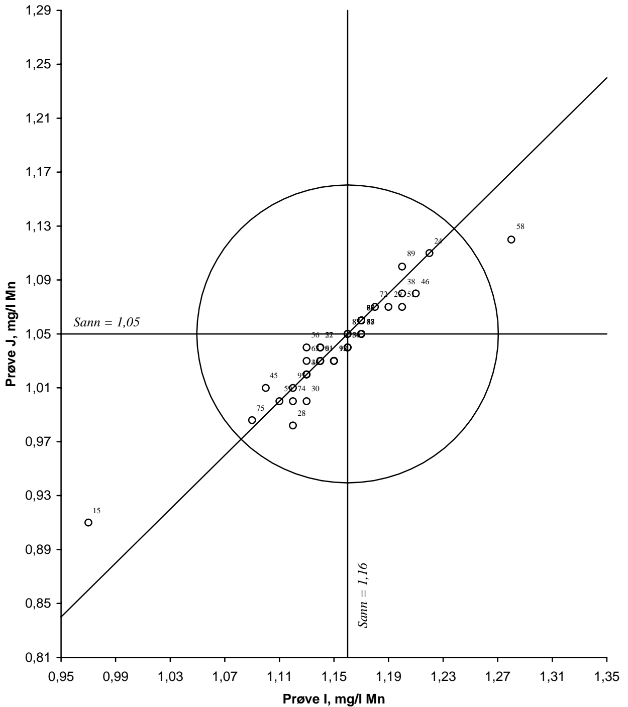
Figur 27. Youndendiagram for mangan, prøvepar IJ Akseptansgrensen, angitt med en sirkel, er 10 %
