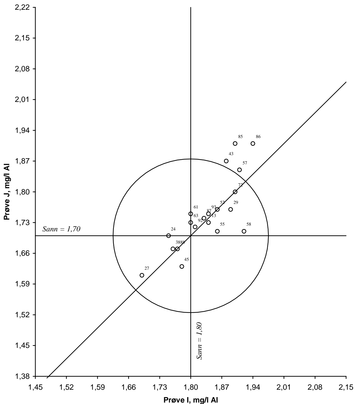
Figur 15. Youdendigram for aluminium, prøvepar IJ Akseptansgrensen, angitt med en sirkel, er 10 %
