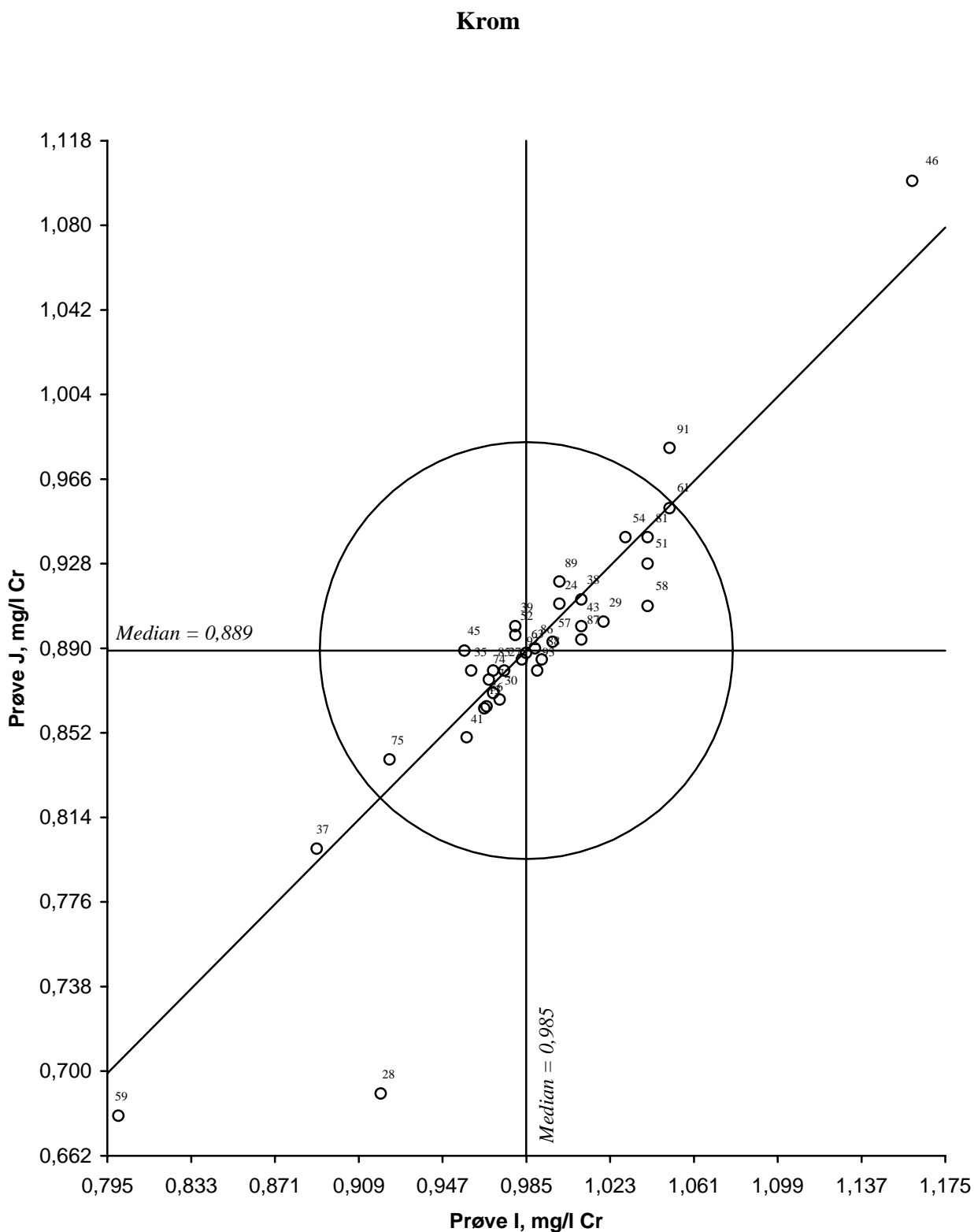
Figur 25. Youtend diagram for krom, prøvepar IJ Akseptansegrensen, angitt med en sirkel, er 10 %
