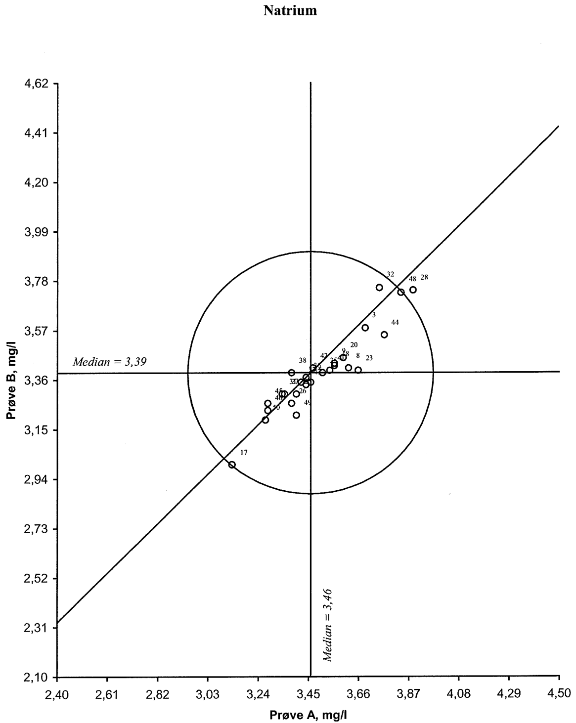
Figur 5. Youtendiagram for natrium, prøvepar AB Akseptansegrensen, angitt med en sirkel, er 15 %
