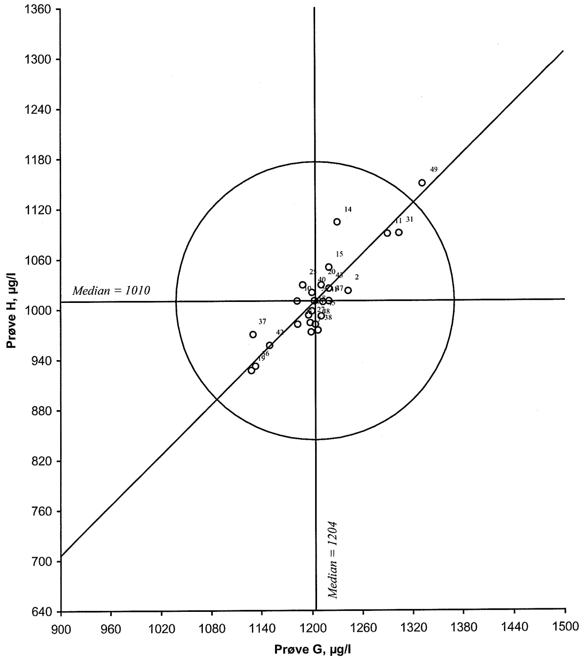
Figur 28. Youndendiagram for nitrat, prøvepar GH Akseptansegrensen, angitt med en sirkel, er 15 %
