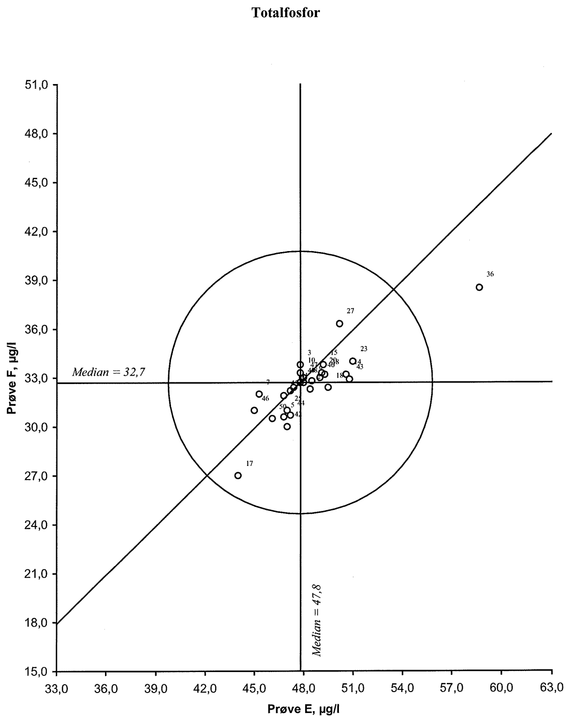
Figur 25. Youtendigram for totalfosfor, prøvepar EF Akseptansegrensen, angitt med en sirkel, er 20 %
