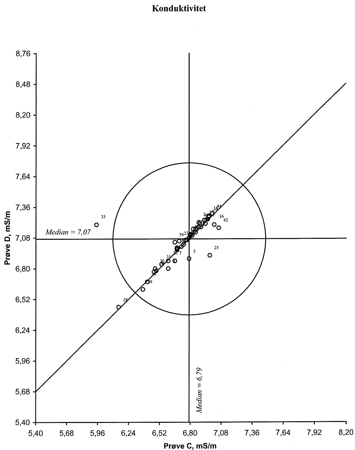
Figur 4. Youdendiagram for konduktivitet, prøvepar CD Akseptansegrensen, angitt med en sirkel, er 10 %
