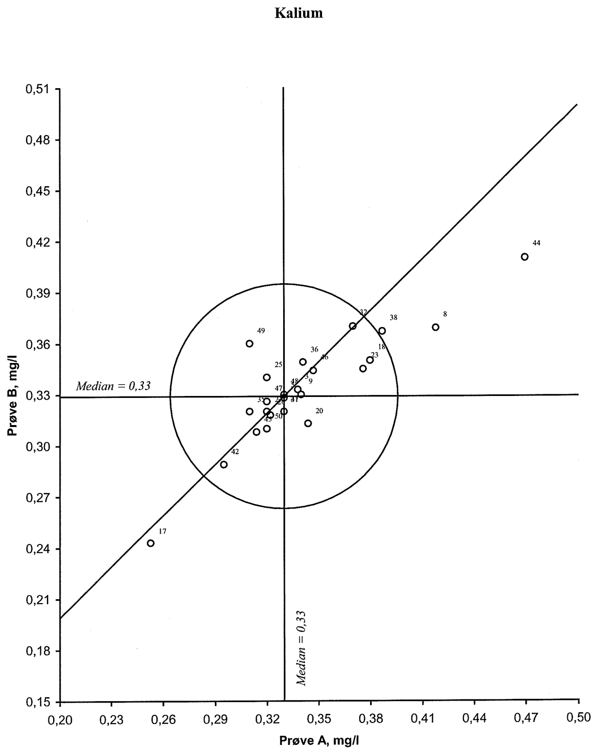
Figur 7. Youdendiagram for kalium, prøvepar AB Akseptansgrensen, angitt med en sirkel, er 20 %
