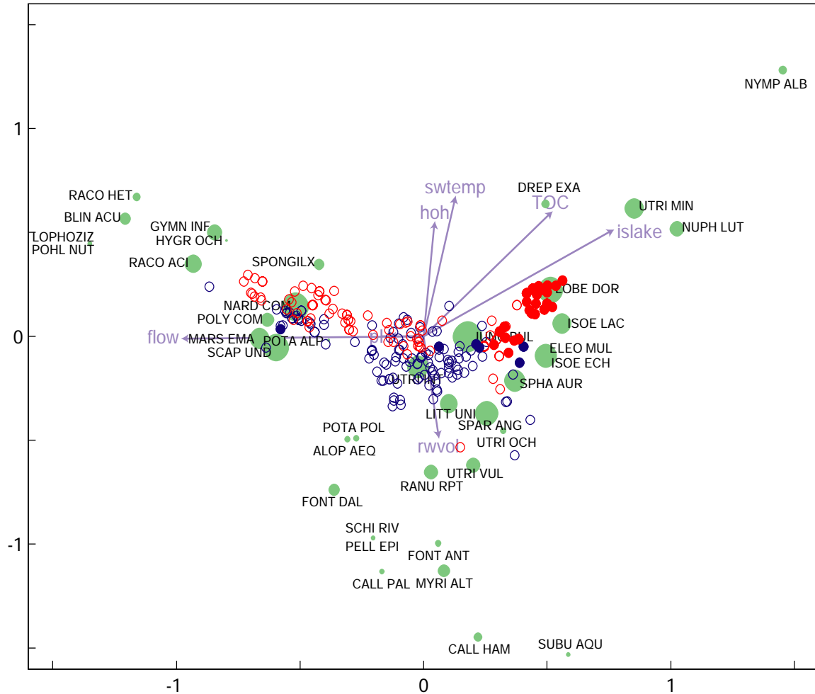
Figur 5. Ordinasijonsdiagram for hele datamaterialet (elve- og innsjøstasjonene) i forhold til 7 miljøvariable (lys blå piler og tekst). Grønne sirkler er artsvekter, med sirkelareal i proporsjon til total forekomst av arten. Stasjonsscorene er vist som røde (Tovdal) og blå (Mandal) sirkler, som er fylte for innsjøstasjonene og åpne for elvestasjonene.
