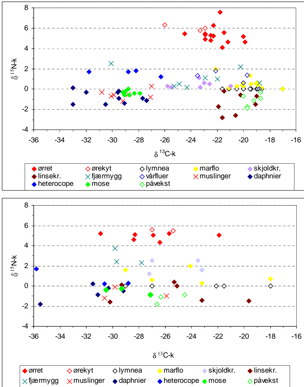
Figur 30. Sammenhengen mellom \delta^{13}\text{C-k} og \delta^{15}\text{N-k} for fisk og næringsdyr i uregulete innsjøer (øvre panel) og regulerte (nedre panel). Alle verdier representerer middelveier for de ulike grupper av organismer.
