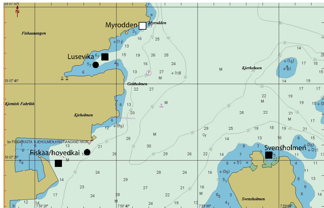
Figur 1. Oversikt over prøvetakingsområdet. Svarte firkanter: utsatte blåskjell/SPMD stasjoner, hvit firkant: stedegne blåskjellpopulasjon, fylt sirkel: sedimentkjernestasjoner.
