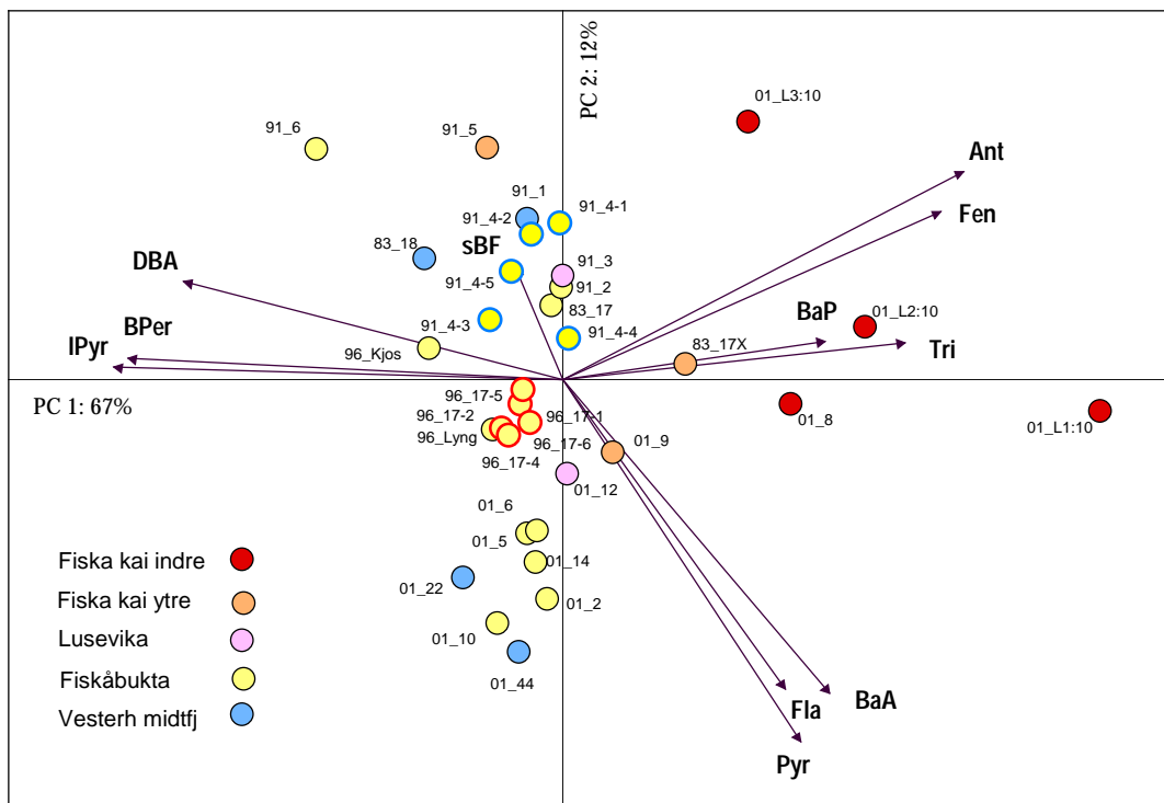
Figur 6. Sammenfattende analyse av PAH-profiler i overflatesedimenter fra Fiskåbukta og midtjords i Vesterhavn utført ved Prinsipal komponentanalyse (PCA). Analysen omfatter prøvene på transekt fra Elkem i Kristiansand til Vesterhavn (se Figur 2), samt prøver tatt ved indre kai ved Elkem i Kristiansand og i indre Fiskåbukta. Forbindelsen fluoren (Flu) mangler i enkelte prøver og er ikke tatt med i analysen.
