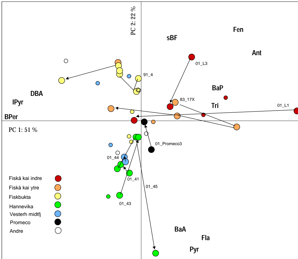
Figur 9. Prinsippal komponentanalyse (PCA) av PAH-profiler i dypsnitt i sedimenter fra Elkem i Kristiansand, i Fiskåbukta og Vesterhav. I analysen er følgende stasjoner og sedimentdyp (cm) tatt med: Fiskå kai indre: Stoveland Consult 2001 st. L1 (10, 50), st. L3 (10, 50); Fiskå kai ytre: st. 17x 1983 (0, 4, 10, 18); Fiskåbukta: st. 4 1991 (0, 2, 4, 6, 8, 12); Hannevika: st. 41 (0, 15), st. 43 (0, 60), st. 45 (0, 30, overgang leire); Vesterhav midt fjords: st. 44 (0, 20); Promeco: st. 3 2001 (0, 30). Piler forbinder prøver fra samme snittserie fra overflate til dypeste snitt. Andre stasjoner (overflatesedimenter) i analysen er vist ved små symboler. Vektorer for PAH-forbindelser er ikke inntegnet for klarhets skyld. Forbindelsen fluoren (Flu) mangler i enkelte prøver og er ikke tatt med i analysen.
