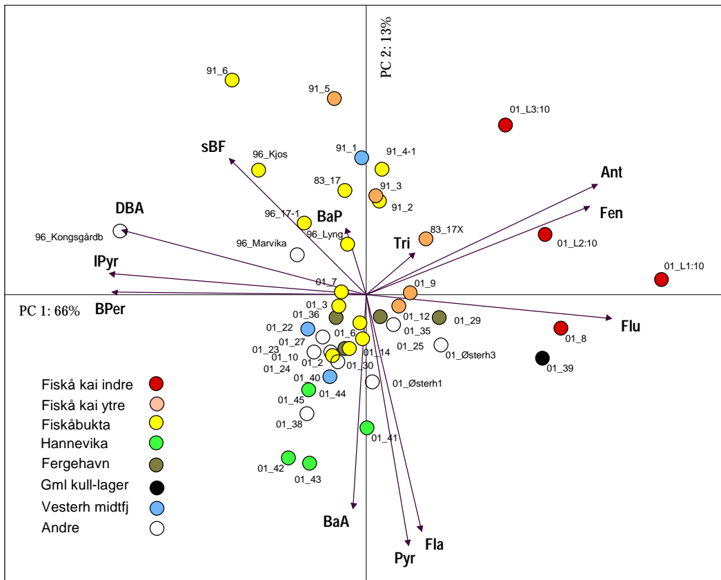
Figur 7. Prinsipal komponentanalyse (PCA) av PAH i overflatesediment ved Elkem i Kristiansand, i Fiskåbukta og Vesterhav.
