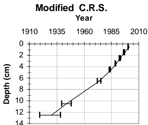
Figur 11. Sedimentets alder med 95 % prediksjonsintervall som funksjon av dybden ved hovedkaia.
