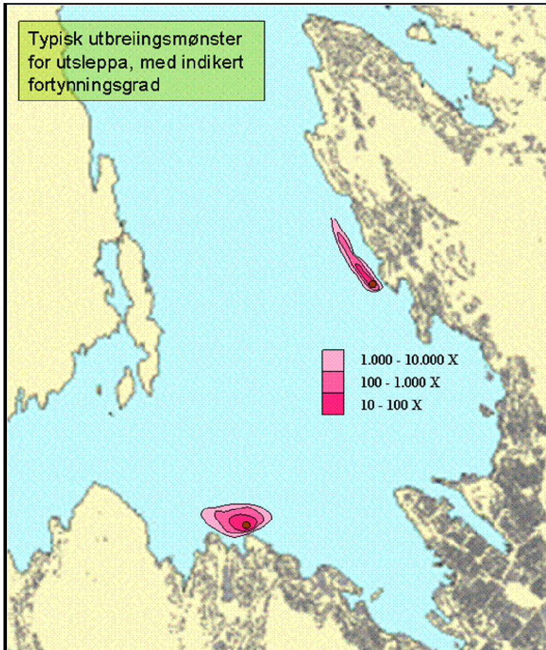
Figur 24. Skisse av typisk fordeling av sporstoffet 3-6 timar etter dosering, med antyda fortynningsgrad.
