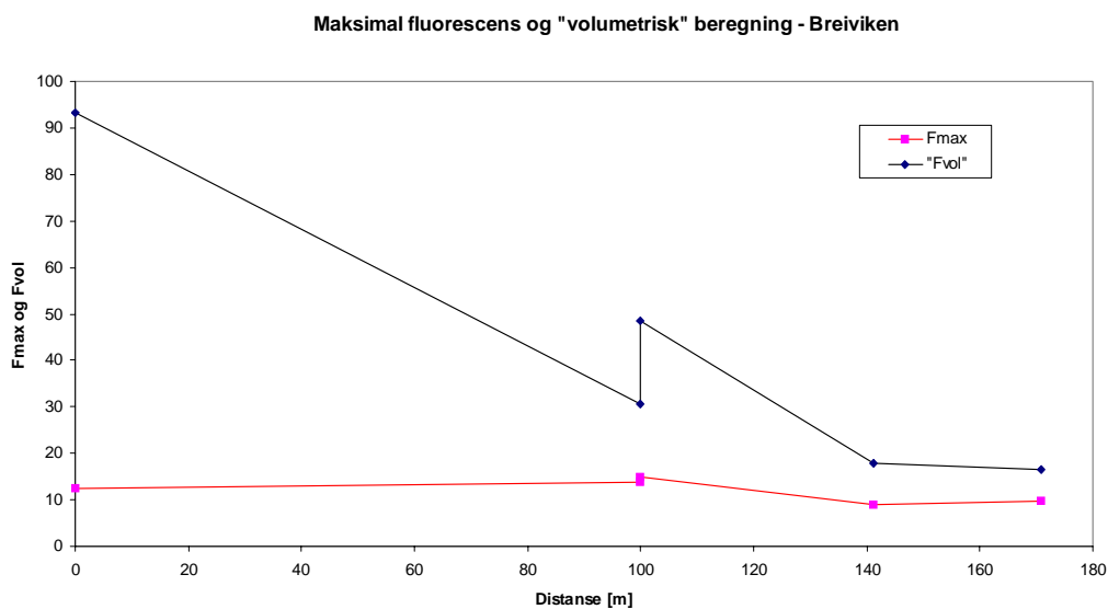
Figur 23. Maksimal F-verdi ved Breiviken 21. mars med eit volumetrisk overslag for fleire profiler (i relasjon til avstand frå utsløppspunktet). "Fvol" er berekna som lag-tjukkjeiken av kvart måleintervall d.v.s. basert på gjennomsnittet for målepunkta i over- og underkant av kvart intervall.
