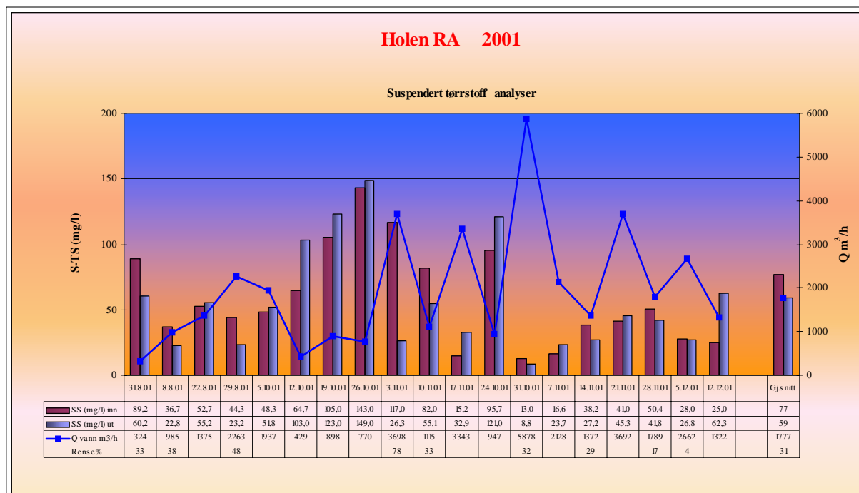
Figur 5. Resultat av analyser for suspendert stoff ved Holen rensanlegg, h.h.v. før og etter silreising, 2001. Vassmengder på dagen for prøvetakinga er også gitt (heiltrekt kurve). Kjelde: Bergen kommune.
