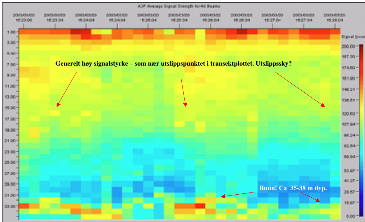
Figur 26. Signalstyrke for to ADP transekt målt 20. mars 2003 over utseppet ved Laksevåg.
