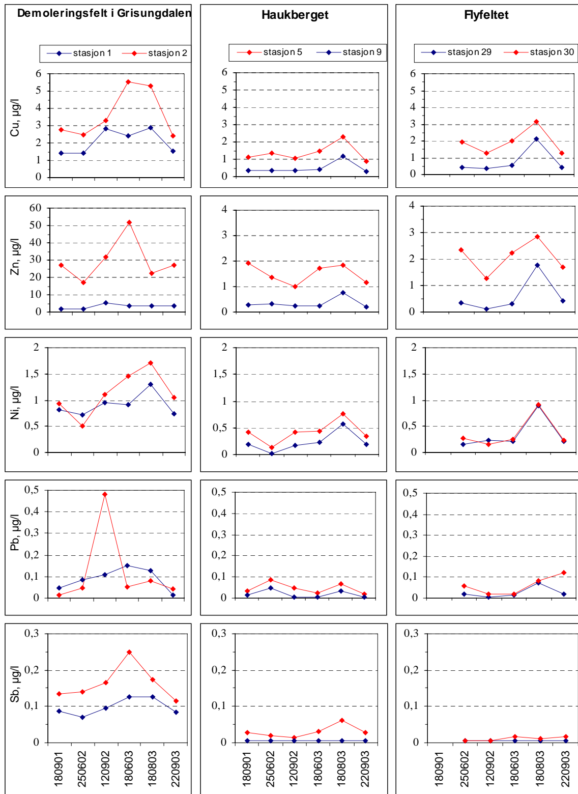
Figur 7. Konsentrasjoner av kobber (Cu), sink (Zn), nikkel (Ni), bly (Pb) og antimon (Sb) i bekkene fra tre viktige delområder i Hjerlinn skytefelt ved 6 ulike tidspunkt i perioden 2001-2003. Blå kurver er målepunktene oppstrøms feltene og rød nedstrøms.
