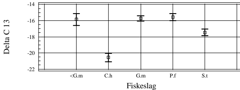
Figur 19. Delta ^{13}\text{C} i fisk fanget i Eidangerfjorden og Frierfjorden i april og juni 2000 og januar 2001. Fiskeslag (G.m=torsk, <G.m=småtorsk, P.f=skrubbe, S.t.=Sjøørret, C.h.=sild) er avmerket.
