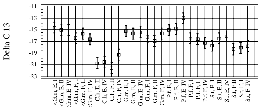
Figur 27. Delta ^{13}\text{C} i fisk fanget i Eidangerfjorden (E) og Frierfjorden (F) i april og juni 2000 og januar 2001. Fiskeslag (G.m=torsk, <G.m=småtorsk, P.f=skrubbe, S.t.=Sjørørret, C.h=Sild), fjordavsnitt (F=Frierfjorden, E=Eidangerfjorden) og tidspunkt (I=april 2000, II=juni 2000, III=januar 2001, IV=januar 2001) er avmerket
