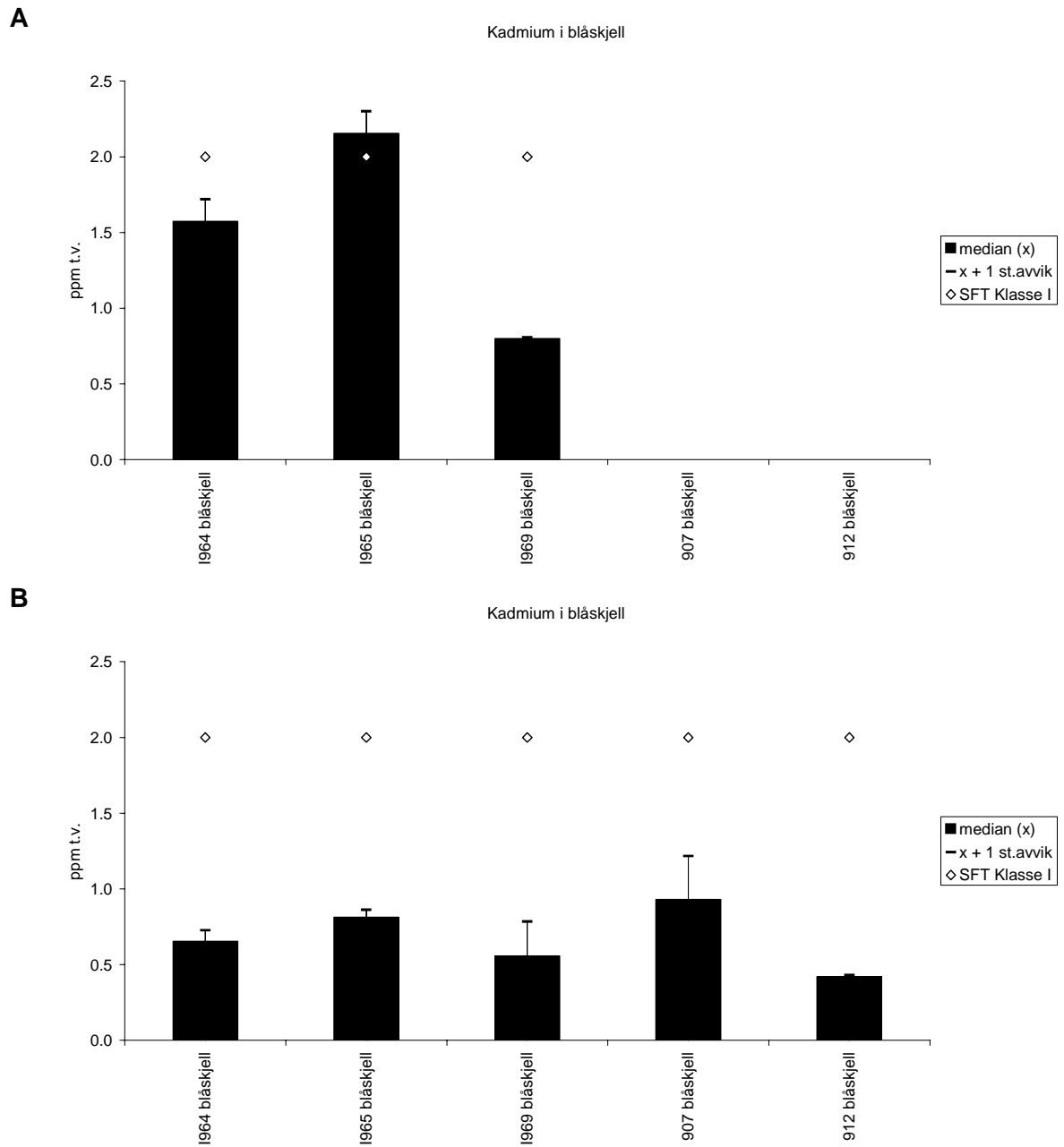
Figur 2. Median, standardavvik og antatt "høy bakgrunn" konsentrasjon (SFT klasse I) for kadmium (Cd) i blåskjell ( Mytilus edulis ) 2002 ( A ) og 2003 ( B ), ppm tørrvekt.
