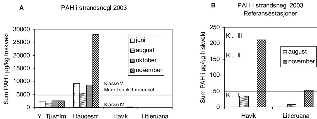
Figur 3. Dagens nivå av PAH i strandsnegl ved Lista. Figuren viser enkeltverdier fra fire ulike stasjoner og fire prøvetakinger gjennom året. Verdiene er oppgitt som sum PAH i \mu\text{g/kg} friskvekt. A viser alle 4 stasjoner mens B viser kun referansestasjoner.
