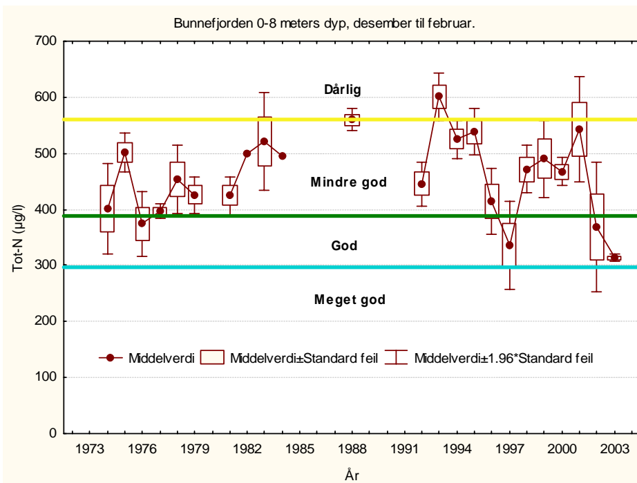
Figur 44. Vinterobservasjoner av Tot-N i Bunnefjorden (Ep 1) i 0, 4 og 8 meters dyp 1973-2003. Utviklingen er sammenlignet med SFT's miljøklassifiseringssystem for vannkvalitet i overflatelaget. Det er ingen endring i vannkvaliteten over tid, som varierer fra dårlig til god . Enkelte år kan avvike som følge av lokale flommer eller varierende tidspunkt for dypvannsfornyelse.
