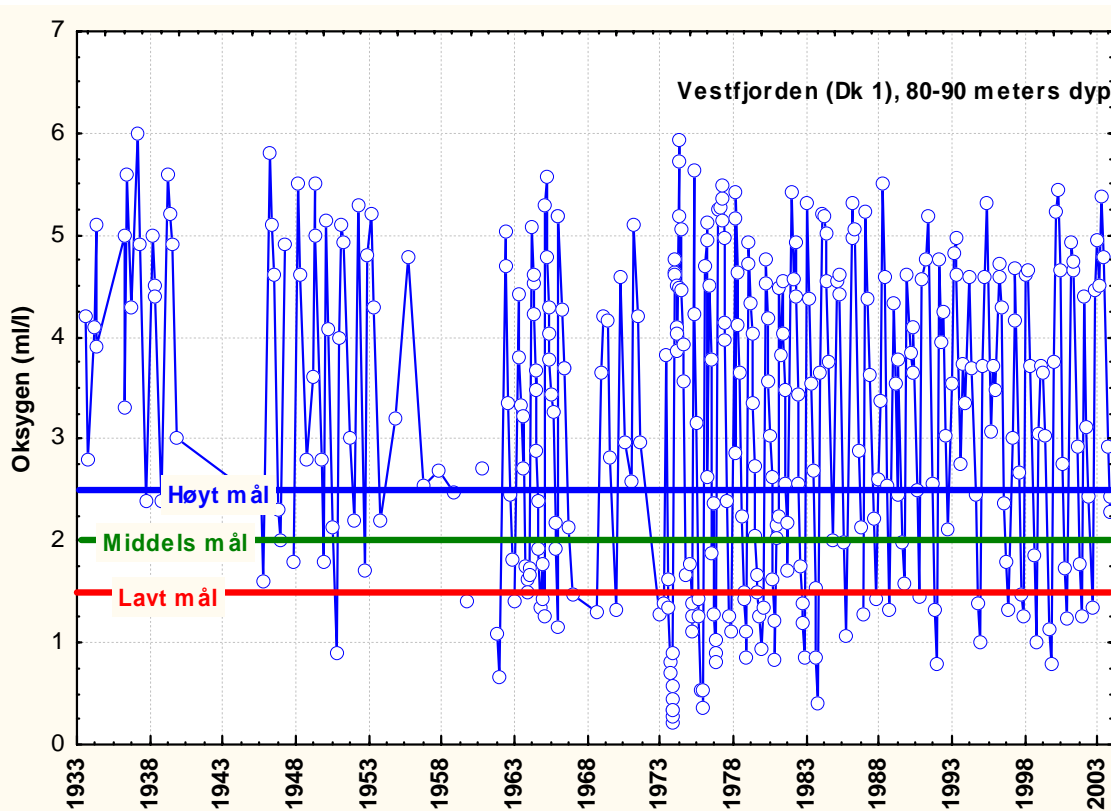
Figur 25. Oksygenkonsentrasjonen på 80-90 meters dyp i Vestfjorden 1934 – 2003. Data fra Braarud og Ruud (1937), Dannevig (1945), Beyer og Føyn (1951), Havforskningsinstituttet Forskningstasjonen Flødevigen (1952-61) og NIVA (1962-2003).
