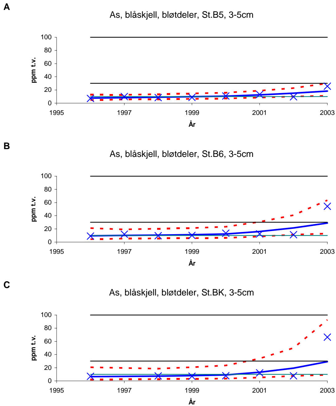
Figur 12. Mediankonsentrasjoner av arsen i blåskjell ( Mytilus edulis ) fra stasjonene B5 ( A ), B6 ( B ) og BK ( C ). Den blå kurven viser glidende middel og rød stiple linje konfidensintervall (cf. Green et al. 2004). De horisontale strekene viser grenser mellom SFTs tilstandsklasser (hhv. I-II, II-III og III-IV).
