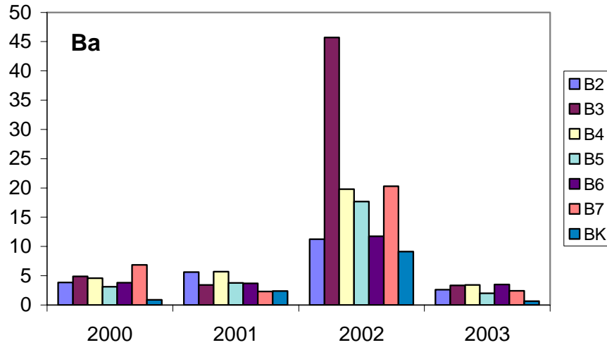
Figur 5. Nivåer av barium i blåskjell fra 6 stasjoner i området rundt Langøya samt på kontrollstasjonen BK. Gjennomsnitt av tre parallelle prøver uttrykt i mg/kg på tørrvektsbasis.
