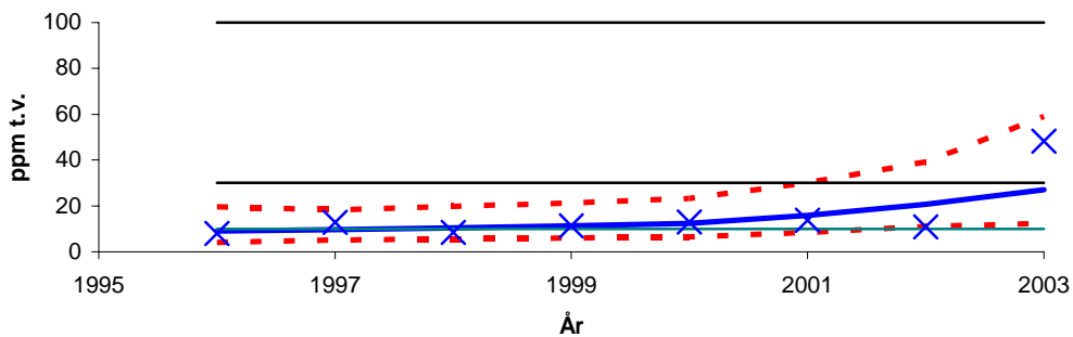
Figur 11. Mediankonsentrasjoner av arsen i blåskjell ( Mytilus edulis ) fra stasjonene B2 ( A ), B3 ( B ) og B4 ( C ). Den blå kurven viser glidende middel og rød stiple linje konfidensintervall (cf. Green et al. 2004). De horisontale strekene viser grenser mellom SFTs tilstandsklasser (hhv. I-II, II-III og III-IV).
