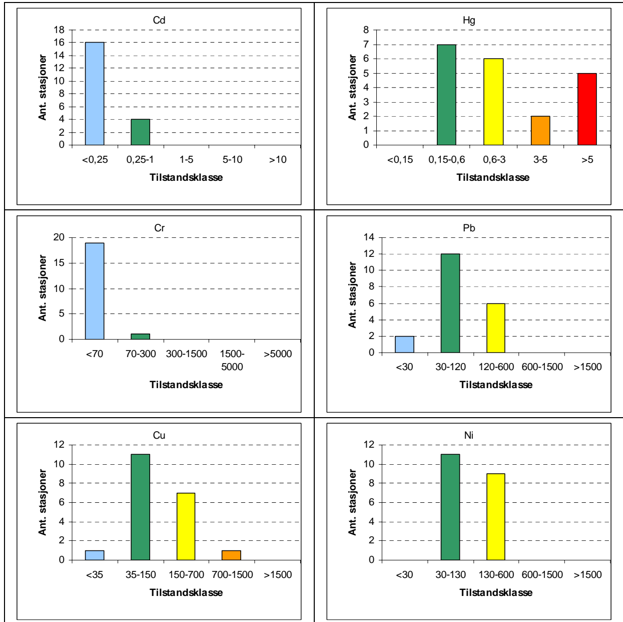
Figur 19. Frekvensdiagram for innhold av kadmium (Cd), kvikksølv (Hg), krom (Cr), bly (Pb), kobber (Cu) og nikkel (Ni) i overflatesedimentene ved Bredalsholmen 2004. Alle konsentrasjoner i mg/kg tørrstoff. Figurene viser antall stasjoner innenfor hver tilstandsklasse i SFTs klassifiseringssystem.
