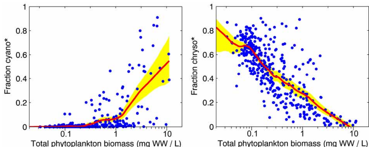
Figur 6. Andel av indikatorgruppene cyano* og chryso* som funksjon av total algebiomasse, basert på middelverdier fra 399 norske innsjøer. Røde linjer er LOWESS-baserte trendlinjer, mens de gule feltene er bootstrapping-genererte 95% konfidensbelter for trendelinjene.
