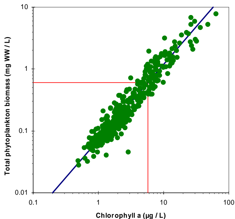
Figur 8. Relasjon mellom middelverdier av total algebiomasse og klorofyll a for 403 norske innsjøer. Klorofyll a -konsentrasjon tilsvarende den foreslåtte grenseverdien for skillet mellom god og moderat økologisk status (uttrykt som total planteplanktonbiomasse) er beregnet fra lineær regresjon mellom log-transformerte variable (blå linje, r^2 = 0.92 , n = 403 ).
