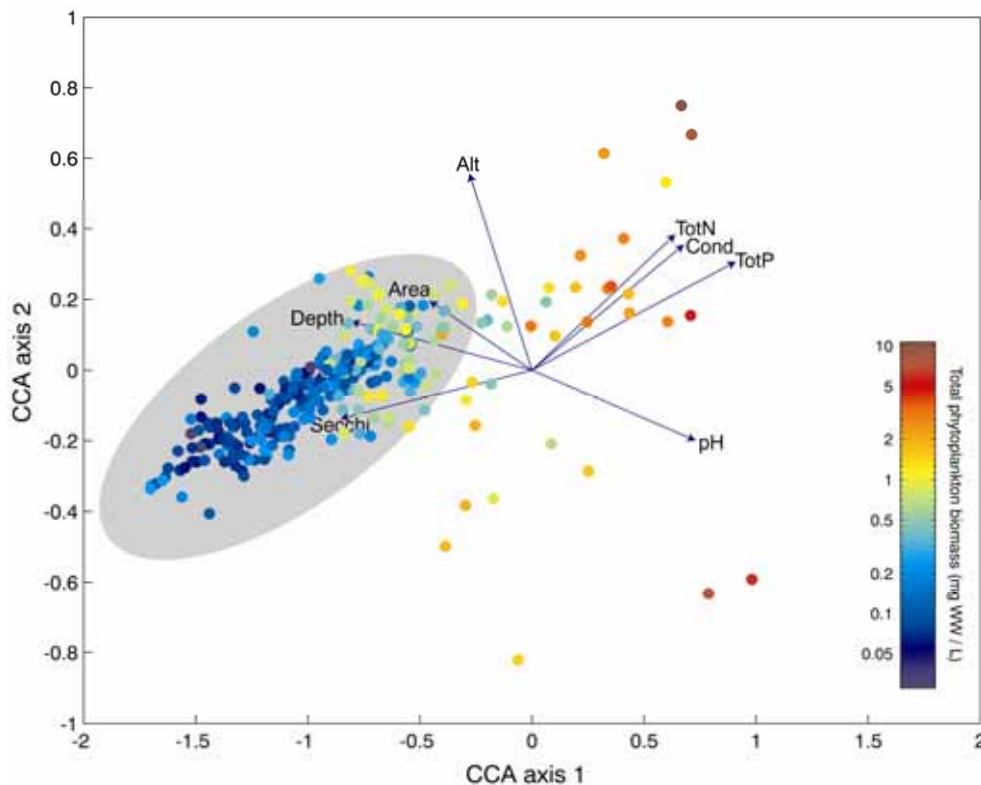
Figur 1. Biplot av de to første ordinasjonsaksene i en CCA-analyse av planteplankton i 326 norske innsjøer, basert på kvadratrottransformerte biomassedata av 203 vanlig forekommende, gode arter. Piler viser gradientvektorer for 8 fysisk/kjemiske og morfo-edafiske miljøvariable. Prikker viser innbyrdes plassering av lokaliteter, fargekodet med hensyn på totalt algevolum. Skravert områder er en omslutningsellipse for lokaliteter med antatt god økologisk status.
