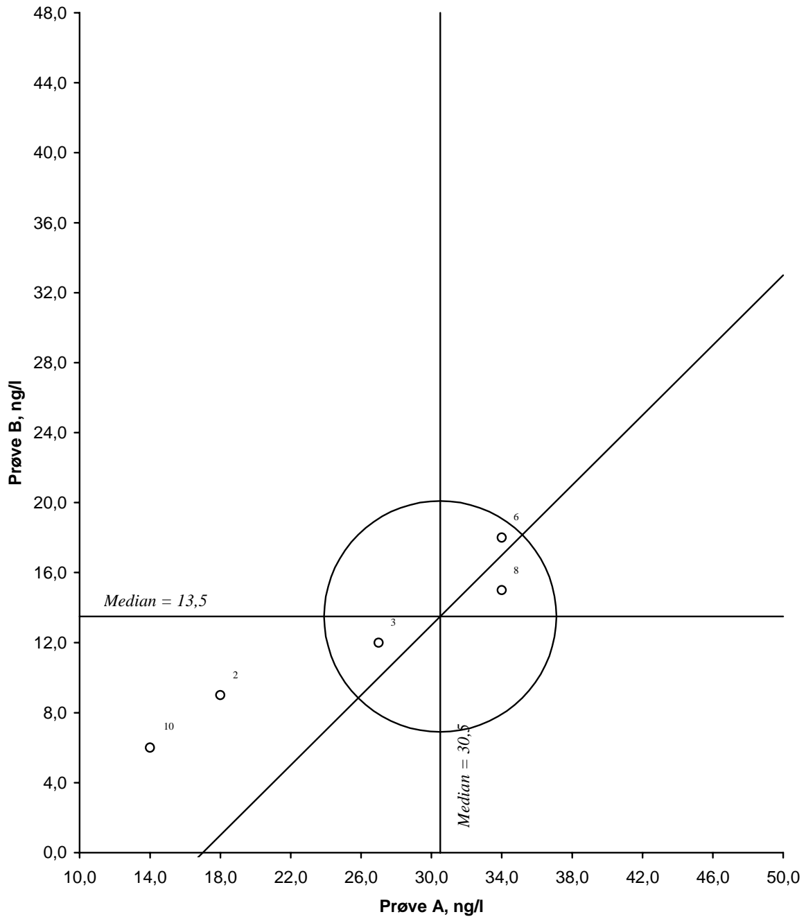
Figur 11. Youndendiagram for benzo(b)fluoranten, prøvepar AB Akseptansegrensen, angitt med en sirkel, er 30 %
