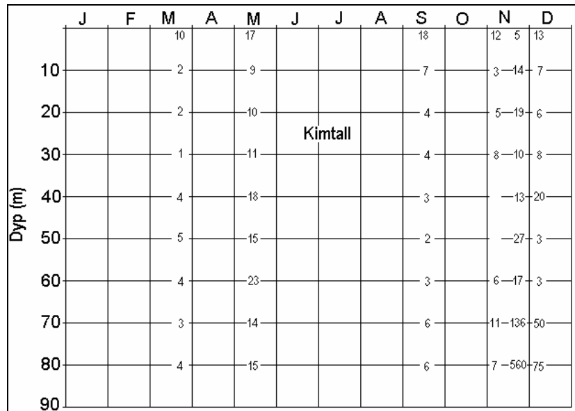
Figur 14. Kimtall (enkeltpøver - bakt per ml) ved hovedstasjonen over dypeste punkt ved de ulike prøvetakingene.
