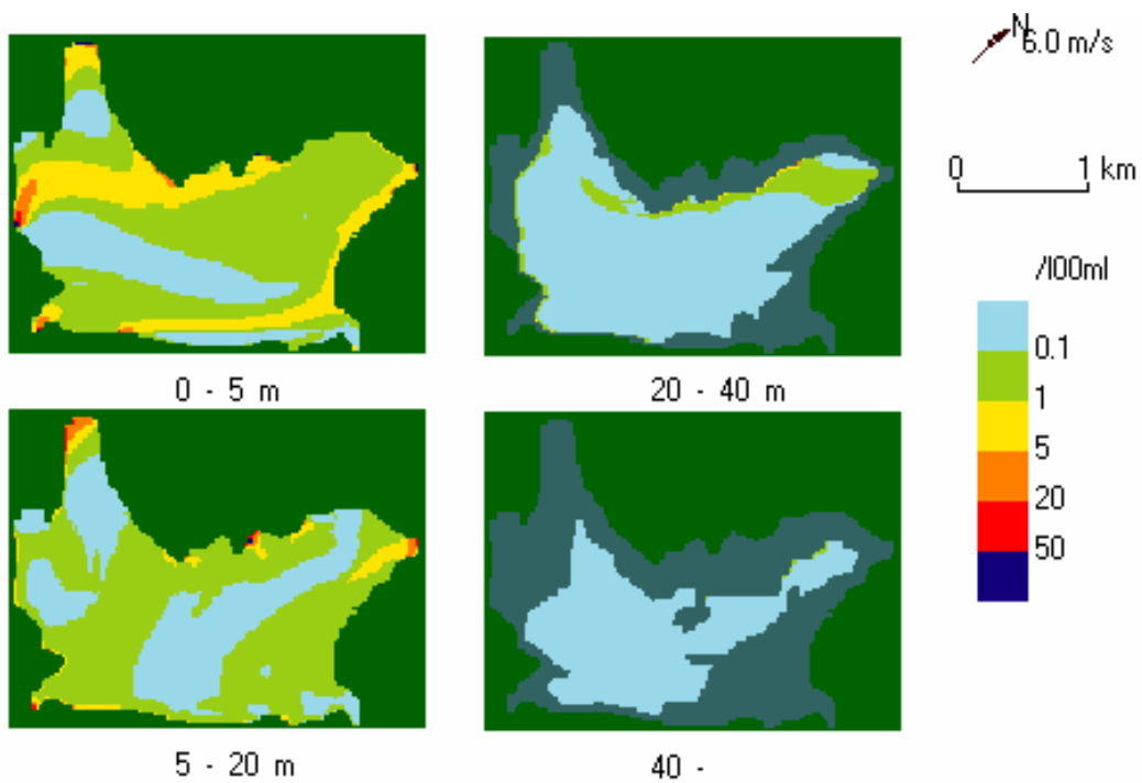
Figur 42. Vind 6 m/s mot nord. Det er lite sannsynlig at vanninntaket blir påvirket av bakterier.
