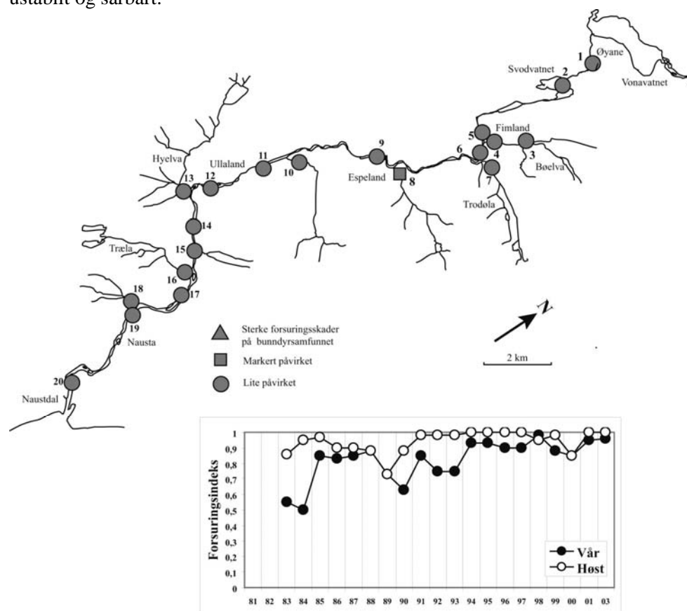
Figur 65. Oversikt over innsamlingslokaliteter og sammensetning av bunndyr i Nausta i 2003. Figuren viser også gjennomsnittlige forsuringssindeksverdier vår (V) og høst (H) i perioden 1983-2003.
