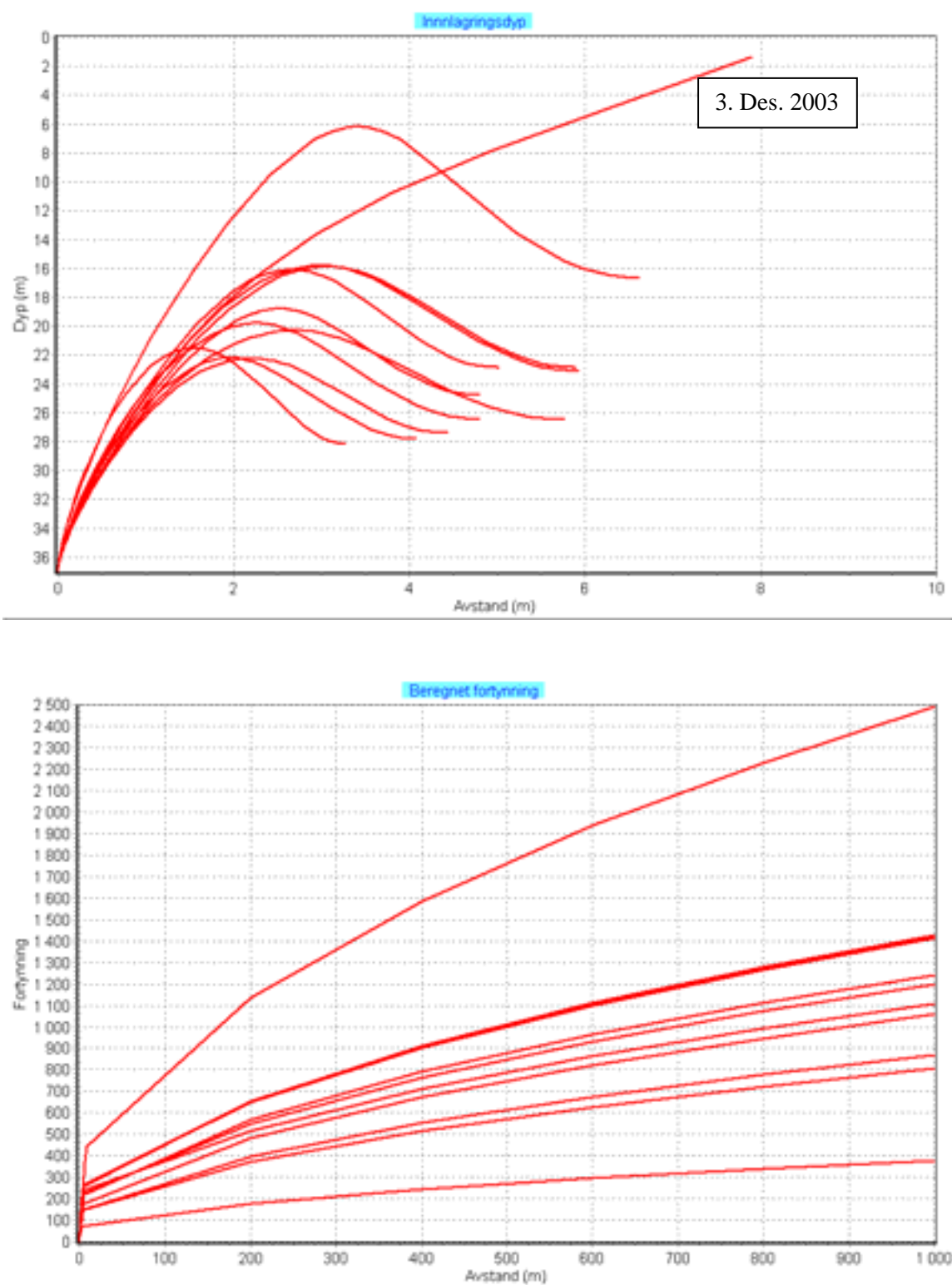
Figur 7. Beregnet innlagringsdyp og fortyning for avløpsvannet fra RA1 ved tidspunktene for prøvetaking. Beregningene er gjort med vannmengden og den vertikale profilen for temperatur og saltholdighet den aktuelle dato. Resultatene påvirkes også av strømhastigheten som varierer med tiden. Her er brukt strømhastighet 2 cm/s (en lav hastighet og som er relativt ugunstig mht. innlagring).
