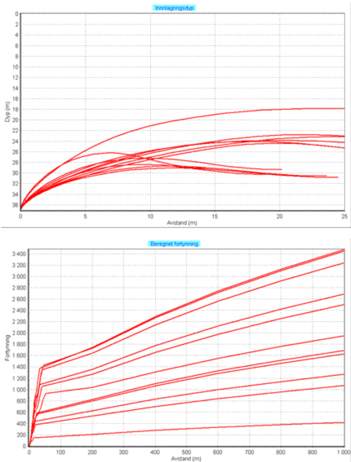
Figur 8. Beregnet innlagringsdyp og fortyning for avløpsvannet fra RA1 ved tidspunktene for prøvetaking. Beregningene er gjort med vannmengden og den vertikale profilen for temperatur og saltholdighet den aktuelle dato. Resultatene påvirkes også av strømhastigheten som varierer med tiden. Her er brukt strømhastighet 20 cm/s (en relativt høy hastighet og som er gunstig mht. innlagringsdyp).
