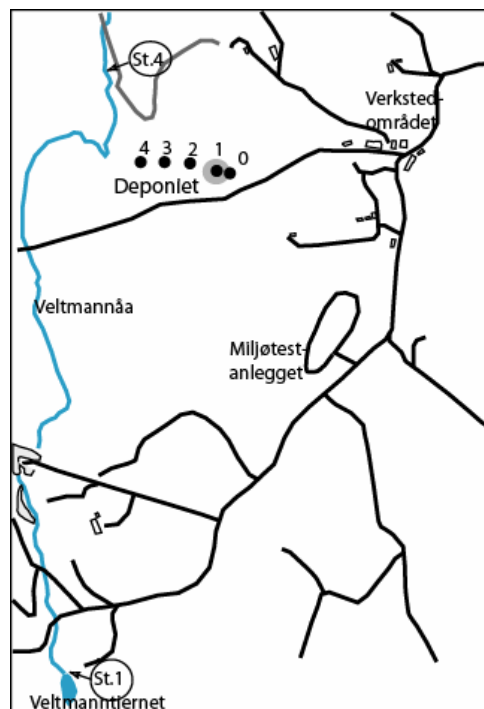
Figur 1. Bradalsmyra testsenter med veinett og prøvetakningspunktene i Veltmannåa (St.1 og 4) og i grunnvannsbrønnene oppstrøms deponiet (0), i deponiet (1) og nedstrøms (2, 3, 4).
