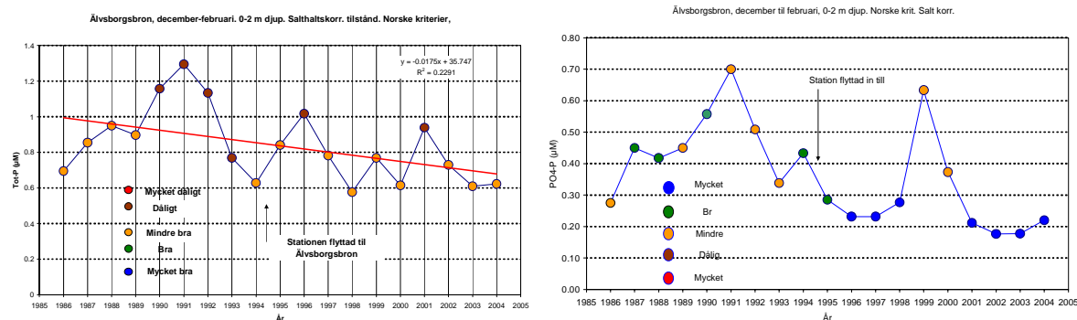
Figur 31. Vintervärden (dec-feb) för tot-P och \text{PO}_4\text{-P} i ytvattnet (0-2 m) vid Älvsborgsbron 1986-2004 ( \mu\text{M} ) jämförda med norska kriterier för miljöklassning (Molvær m fl 1997). Värdeklasserna är korrigerade för salthalten. Pilen markerar när mätstationen flyttades till öster om Älvsborgsbron 1994.
