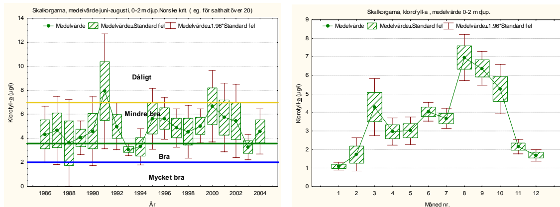
Figur 29. Mätvärden för klorofyll a i ytvattnet (0-2 m) vid Skalkorgarna 1986-2004 ( \mu\text{M} ). Till vänster jämförda med norska kriterier för miljöklassning (Molvær m fl 1997). Till höger variationen av klorofyll a över året. Sommarvärden, jun-aug.
