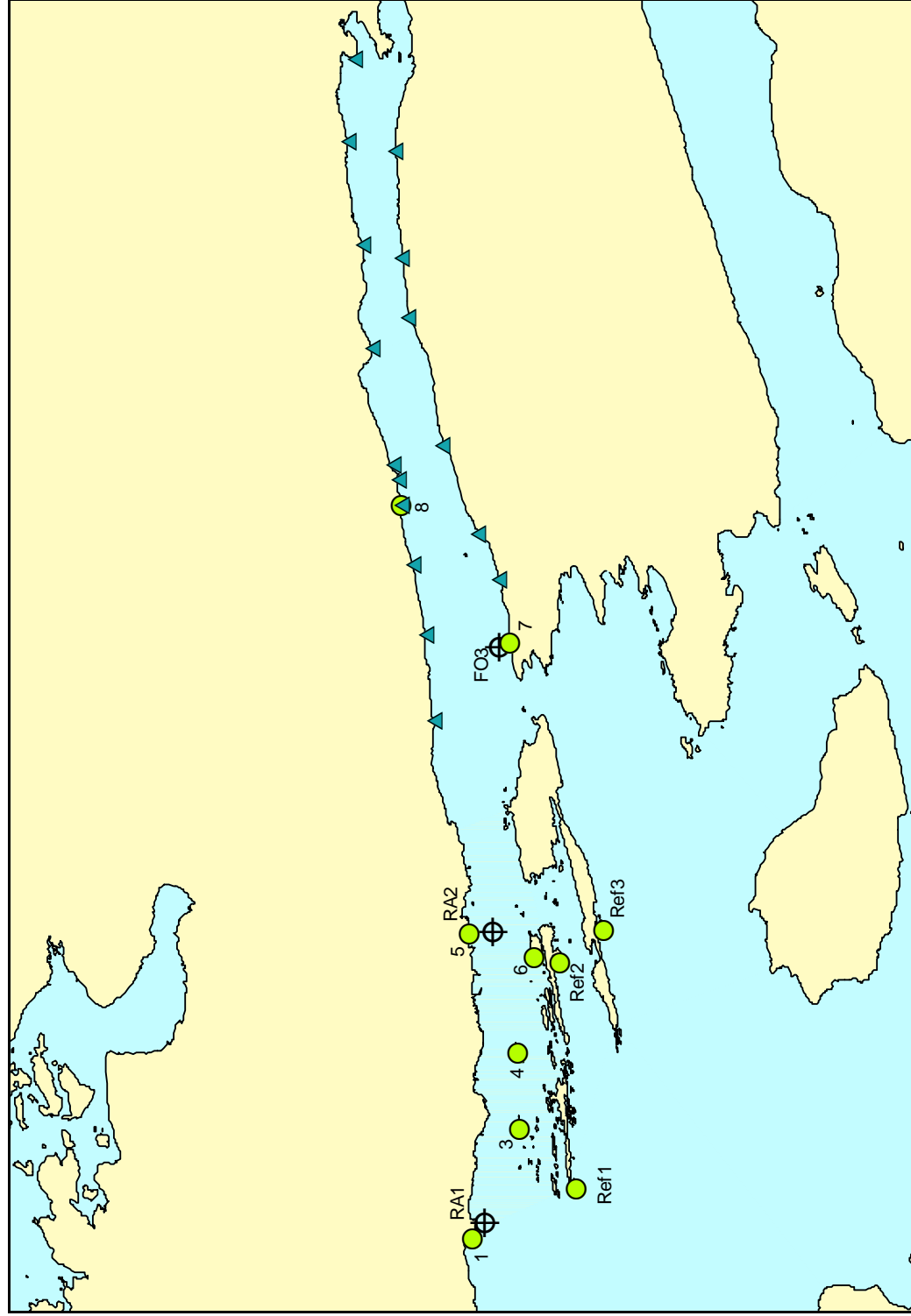
Figur 3. Viser plasseringen av stasjoner for undersøkelse av hardbunnsamfunn. Dykkeregistreringer ble gjort på st. 2 og st 13 (ref 3). Trekantene angir sted for befaring i fjæra. RA1 og RA2 er posisjon for kommunalt utslipp. FO3 er posisjon for oppdrettsanlegg.
