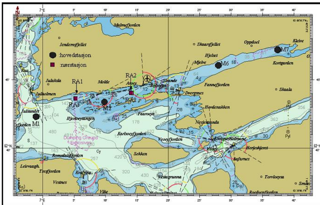
Figur 1. Oversiktskart med posisjon for rensenanleggene RA1 og RA2 og de viktigste hydrokjemiske stasjonene.
