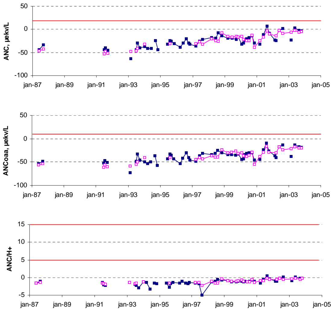
Figur 13. ANC, \text{ANC}_{\text{ooa}} og \text{ANC}/\text{H}^+ for Lille Hovvatn. De respektive kritiske verdier i forhold til fare for skader på aure er vist med røde linjer. Kritiske verdier er hhv. 19 og 8 \mu\text{ekv/L} for ANC og \text{ANC}_{\text{ooa}} (se avsnitt 4.1.1) og 5 og 15 (ubenevnt) for \text{ANC}/\text{H}^+ (se kapittel 3). Se forrige figur for stasjonsforklaring.
