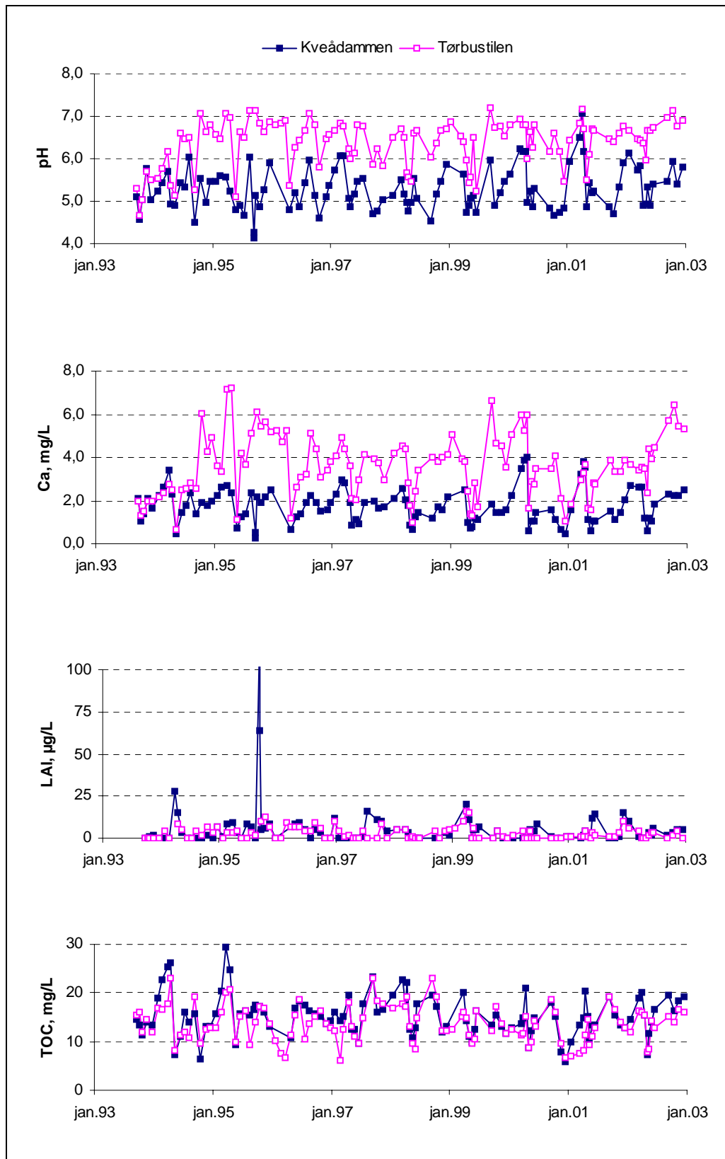
Figur 4. Vannkjemiske data fra Flakstadelva. LAI er løst, uorganisk Al ( Al_i ). Kveådammen er ukalket referansestasjon, mens Tørbustilen er nedstrøms kalking. Kalking startet i 1994.
