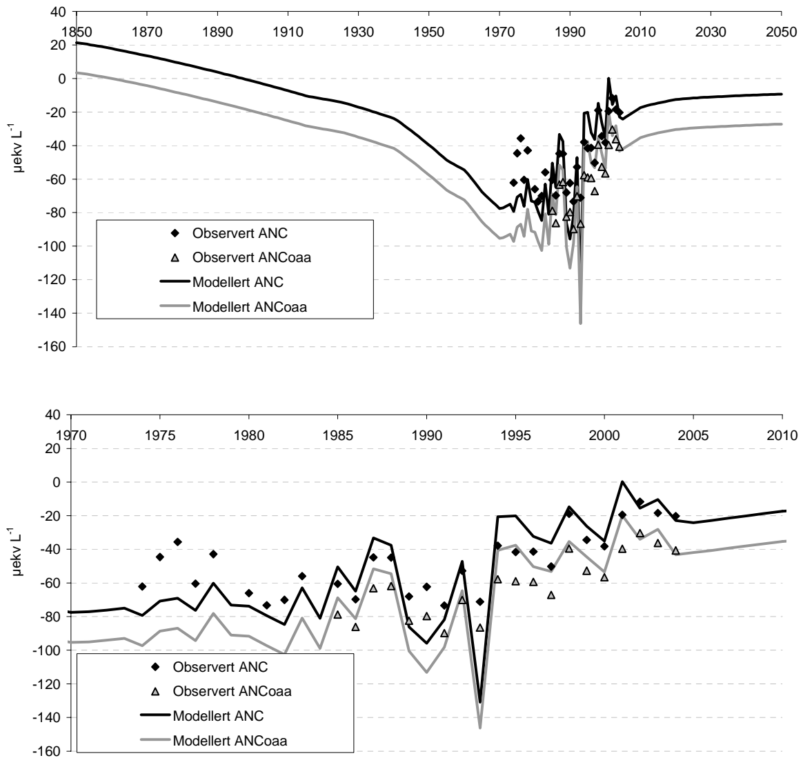
Figur 17. Eksempel på forskjellen mellom ANC og \text{ANC}_{\text{ooa}} ved dynamisk modellering. De heltrukne linjene viser modellberegninger med MAGIC modellen (svart linje er ANC, grå linje \text{ANC}_{\text{ooa}} ). Punktene viser beregnet ANC (svart) og \text{ANC}_{\text{ooa}} (grå) basert på observasjonene. Data benyttet i eksempelet er fra feltforskningsområdet Birkenes.
