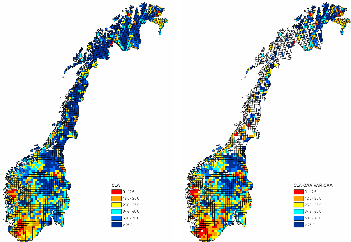
Figur 15. Tålegrenser for overflatevann med og uten hensyn til organiske anioner. I kartet til venstre er variabel ANC-grense (standard ANC_{limit, var} ) benyttet, til høyre variabel ANC-grense justert for organiske anioner ( ANC_{limit, var, oaa} ). Beregningene er gjort med SSWC modellen. For en del felt i Midt- og Nord-Norge er det brukt diverse dataserier uten TOC, derfor hvite felt i kartet til høyre.
