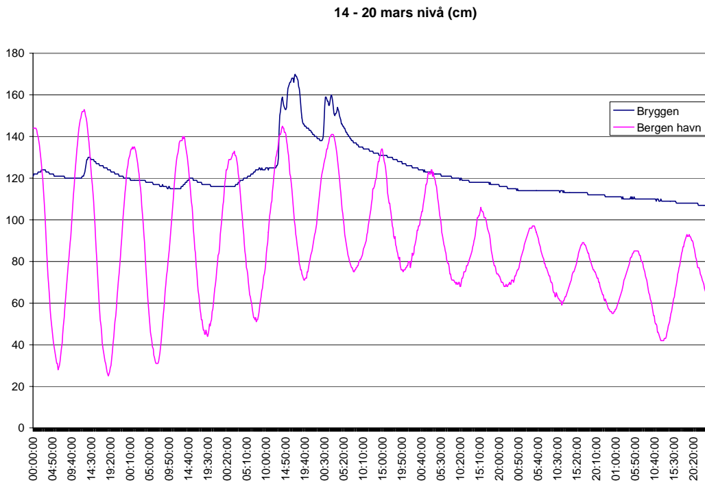
Figur 22. Målt vannstand i brønnen og i Vågen i perioden 14. – 20. mars.
