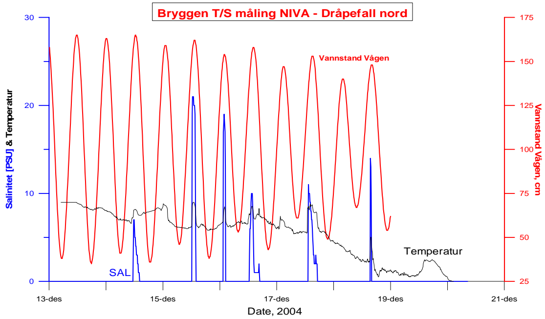
Figur 14. Målt salinitet og temperatur i posisjon C, i dråpefallet ved Bredsgården, 13. – 21. desember 2004. Kurve for vannstand i Vågen er også inkludert.
