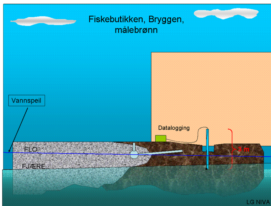
Figur 7. Skisse av måleopplegget for vannstand i brønnen i fiskebutikken. Toppen av brønnen er målt til 1,64 m o.h.
