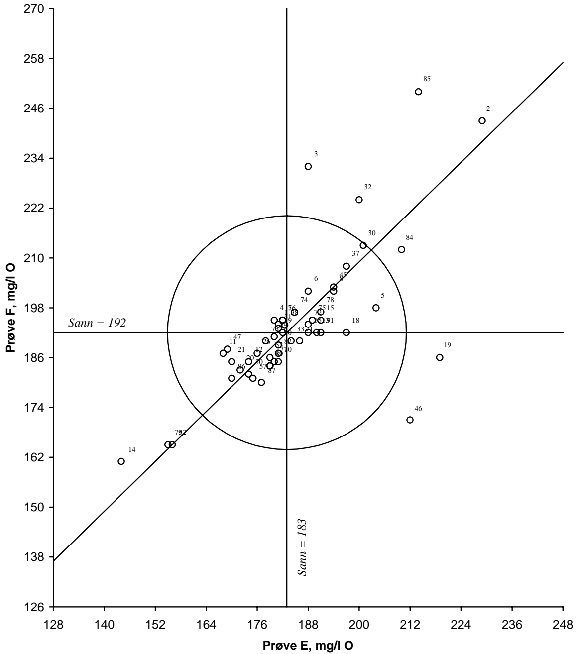
Figur 7. Youdendigram for kjemisk oksygenforbruk, COD_{Cr} , prøvepar EF. Akseptansegrensen, angitt med en sirkel, er 15 %
