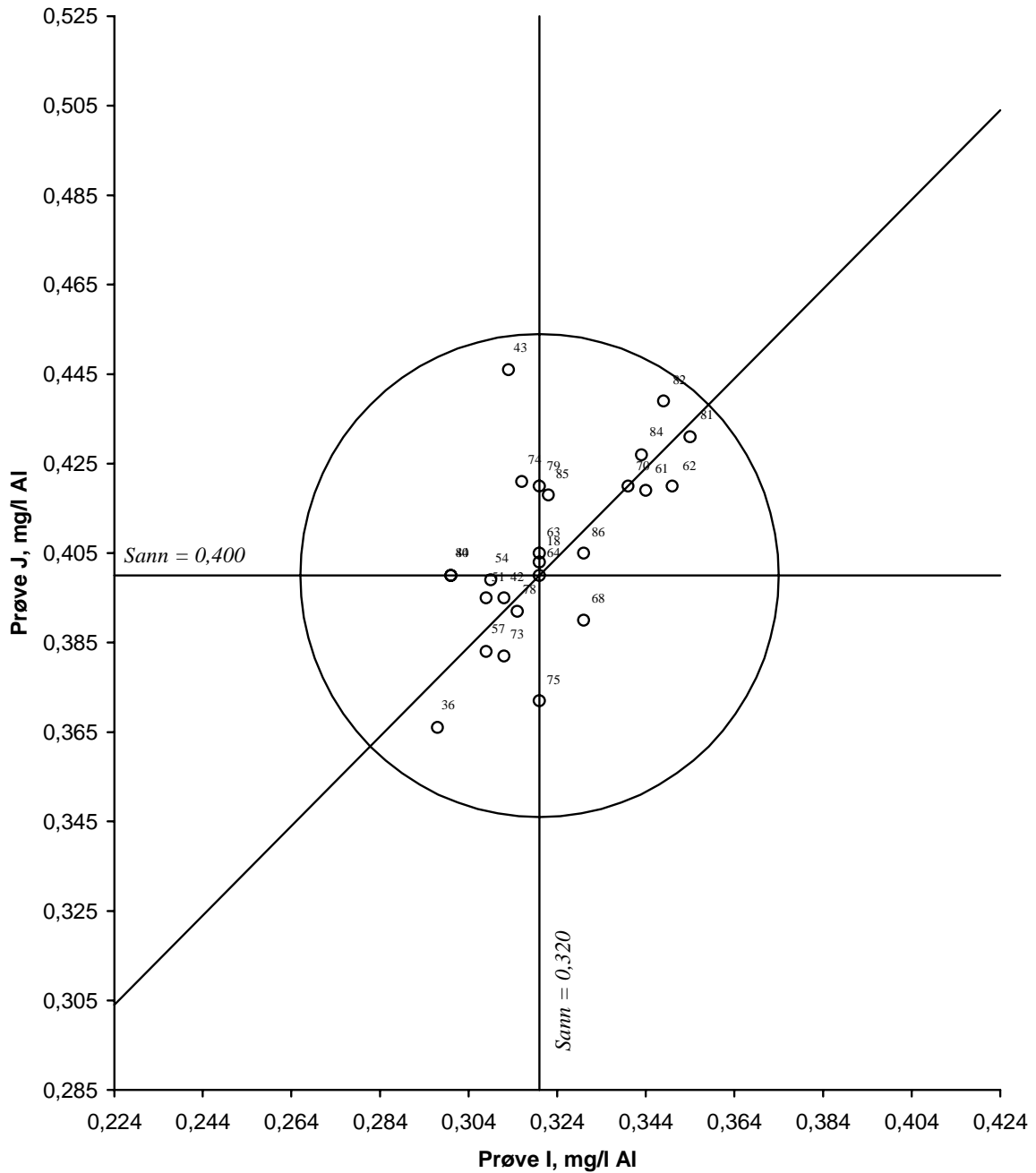
Figur 19. Youdendiagram for aluminium, prøvepar IJ Akseptansgrensen, angitt med en sirkel, er 15 %
