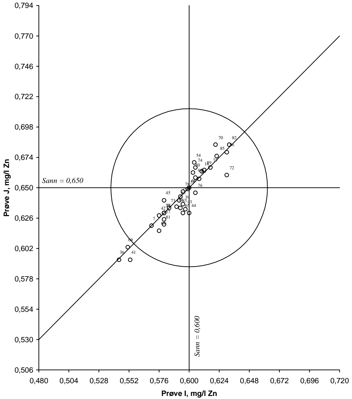
Figur 35. Youtendigram for sink, prøvepar IJ Akseptansegrensen, angitt med en sirkel, er 10 %
