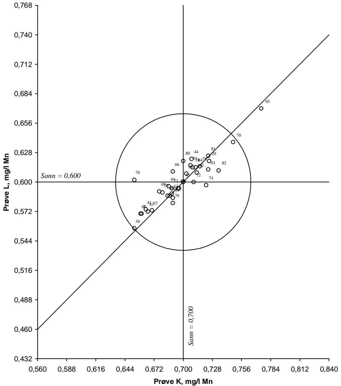
Figur 32. Youdendiagram for mangan, prøvepar KL Akseptansgrensen, angitt med en sirkel, er 10 %
