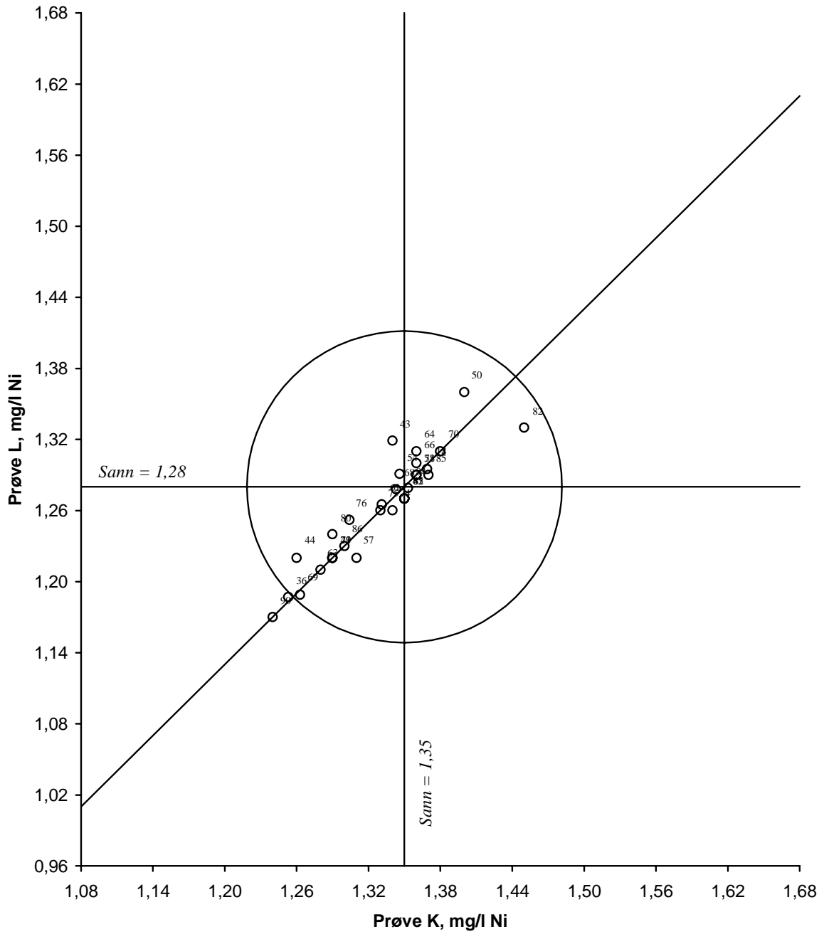
Figur 34. Youdendiagram for nikkell, prøvepar KL Akseptansgrensen, angitt med en sirkel, er 10 %
