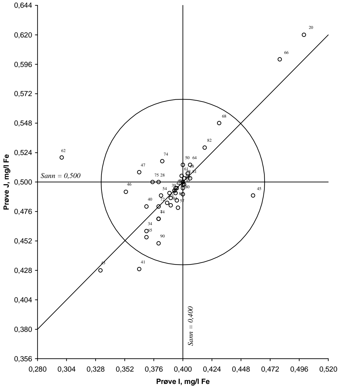
Figur 23. Youndendiagram for jern, prøvepar IJ Akseptansegrensen, angitt med en sirkel, er 15 %
