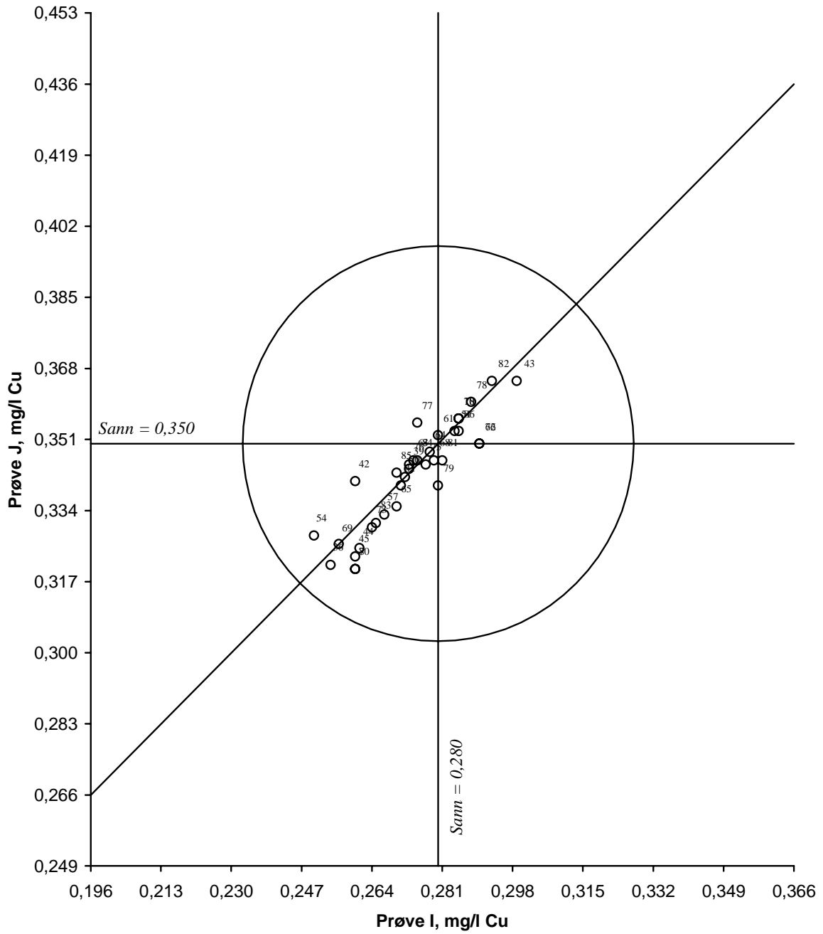
Figur 27. Youdendiagram for kobber, prøvepar IJ Akseptansgrensen, angitt med en sirkel, er 15 %
