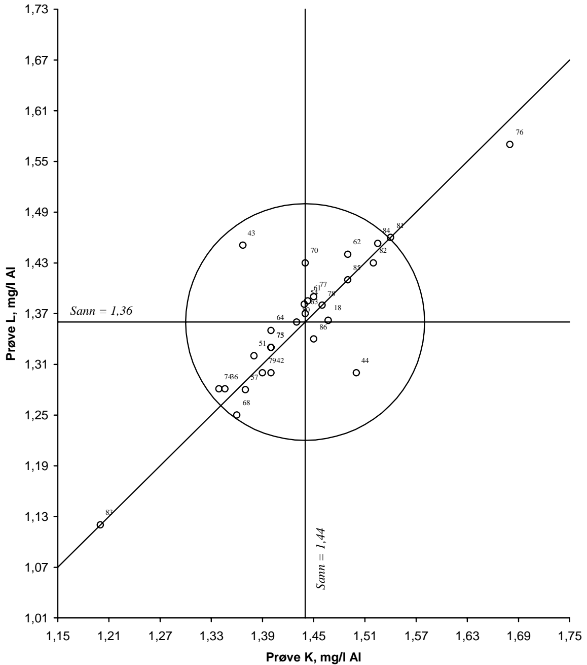
Figur 20. Youdendiagram for aluminium, prøvepar KL Akseptansgrensen, angitt med en sirkel, er 10 %
