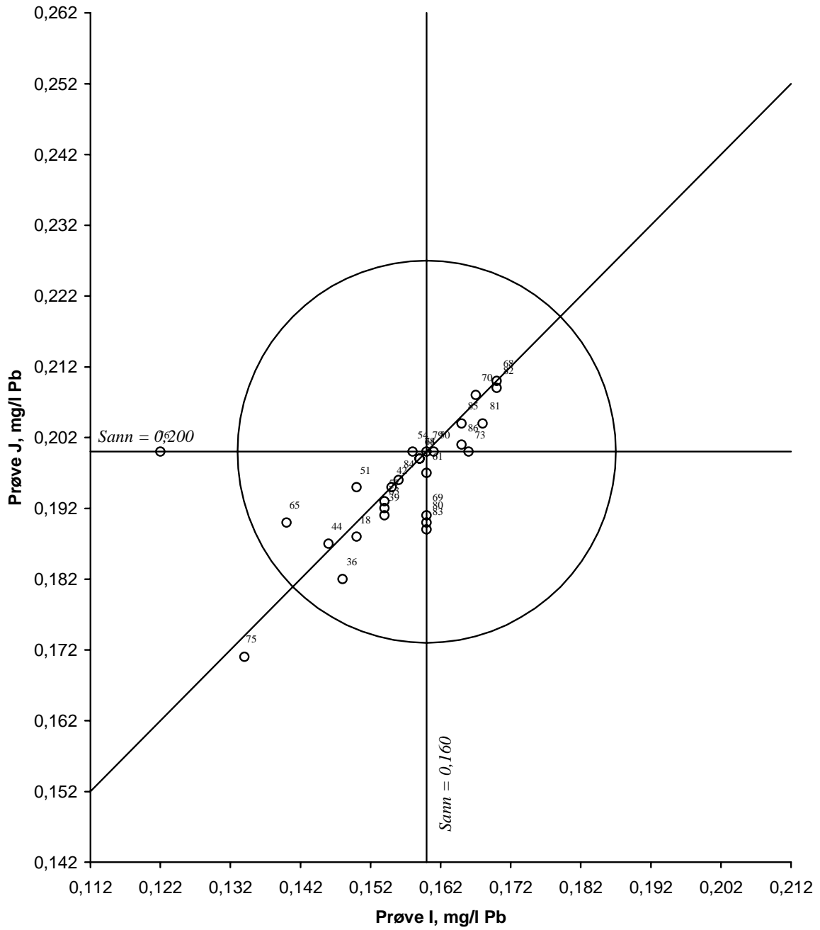
Figur 21. Youndendiagram for bly, prøvepar IJ Akseptansgrensen, angitt med en sirkel, er 15 %
